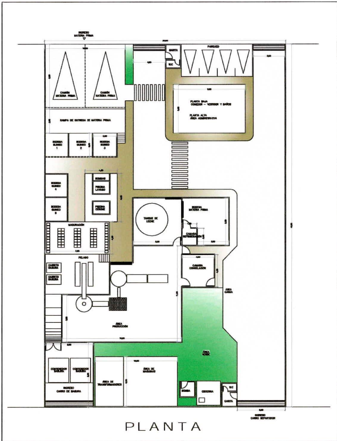
Gráfico 5.7 Diseño de la Planta CARMAGI S.A.
