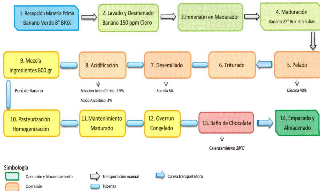
DIAGRAMA DE FLUJO DEL DIP DE CHOCOBANANO
