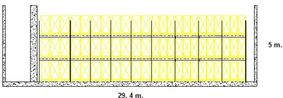
FIGURA 3.7 VISTA LATERAL DEL ALMACÉN.
