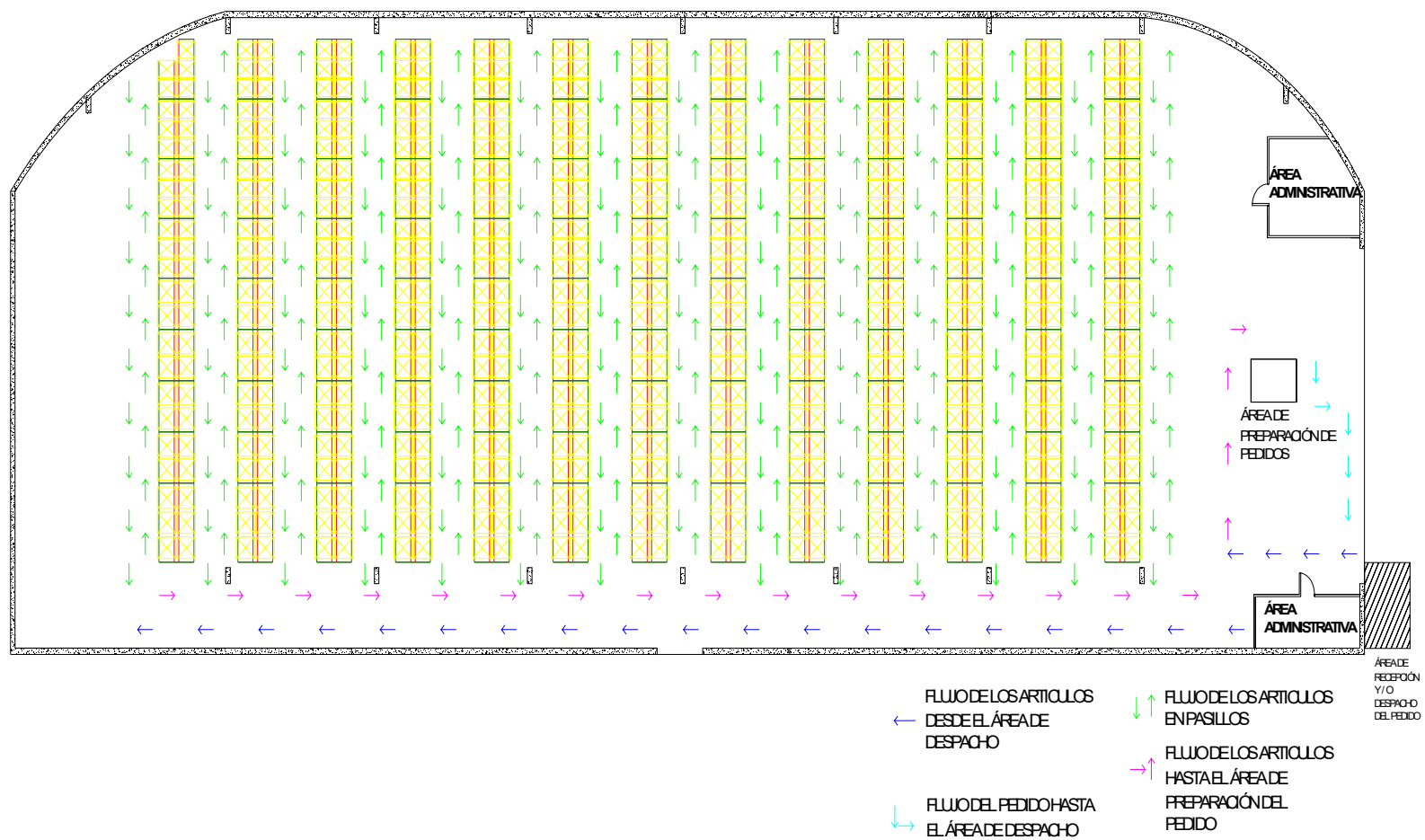
FIGURA 3.14 DISEÑO ACTUAL DEL ALMACÉN Y FLUJO DE MATERIALES
