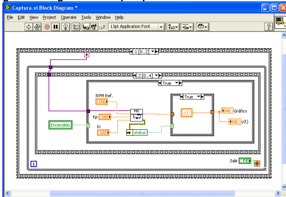
Figura 4.2 Diagrama de bloques para interfaz del control de motor
