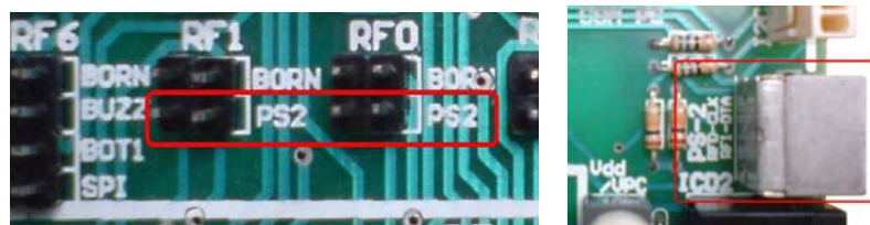
Figura 4.28. Conector PS/2 y sus habilitadores
