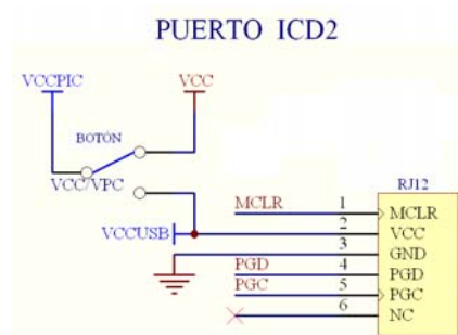
Figura 4.34. Esquema ICD2
