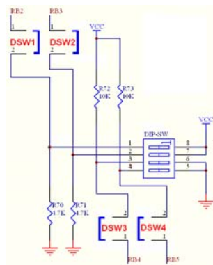
Figura 4.11. Esquema de micro-interruptores
