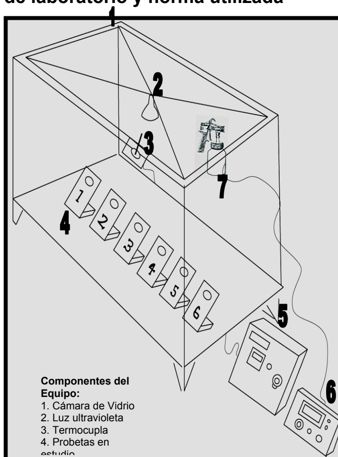
FIGURA 2.4 COMPONENTES DEL EQUIPO PARA ENSAYO DE CORROSION ACELERADA
