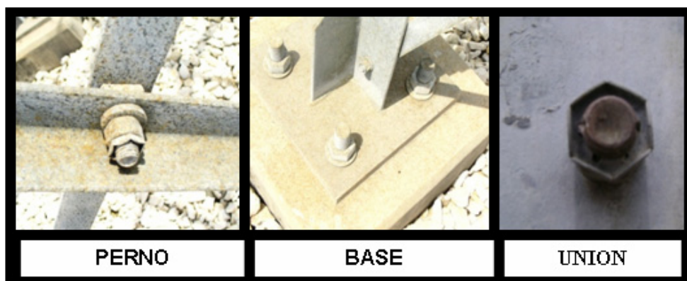
FIGURA1.6 DESTRUCCION DEL GALVANIZADO DE UNIONES SOLDADAS, BASES Y PERNOS
