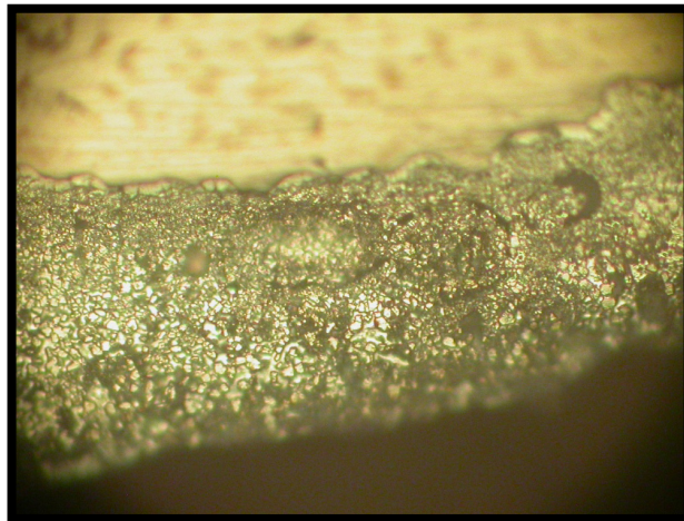
FIGURA 2.9 MICROESTRUCTURA DE ACERO GALVANIZADO EN CALIENTE
