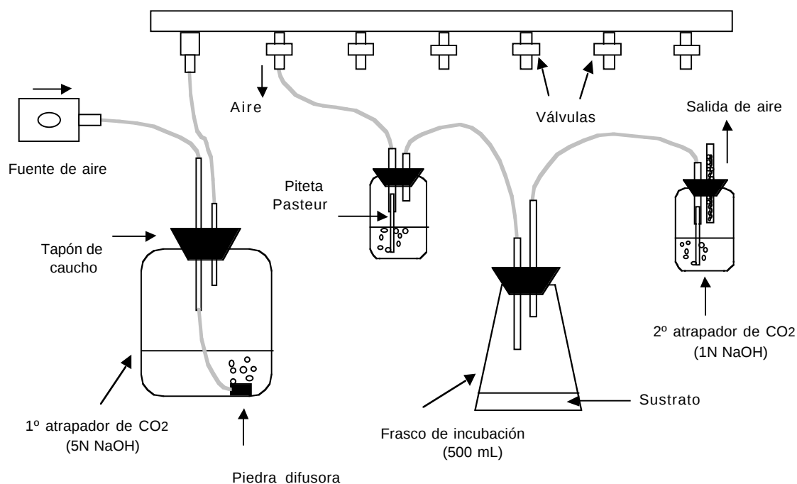
Figura 1: Esquema del aparato de aireación continua.
