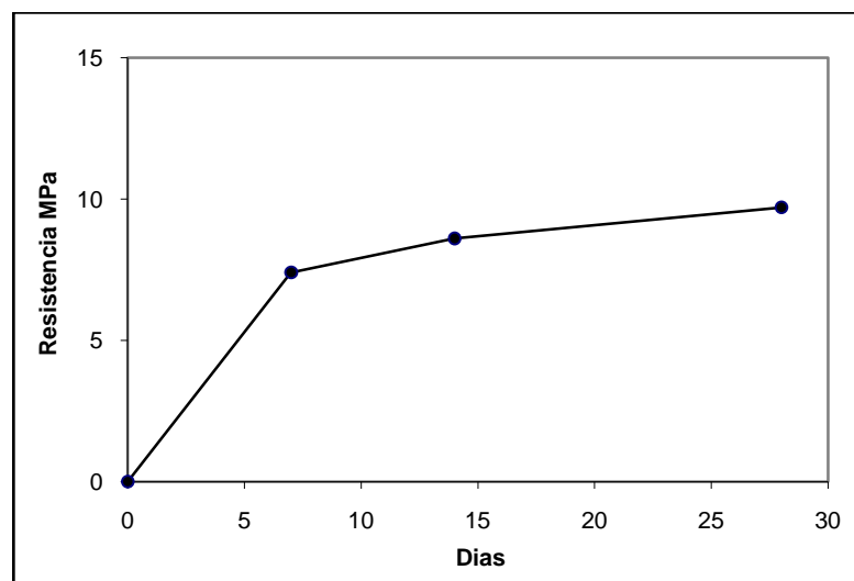
Curva Resistencia vs. Tiempo
