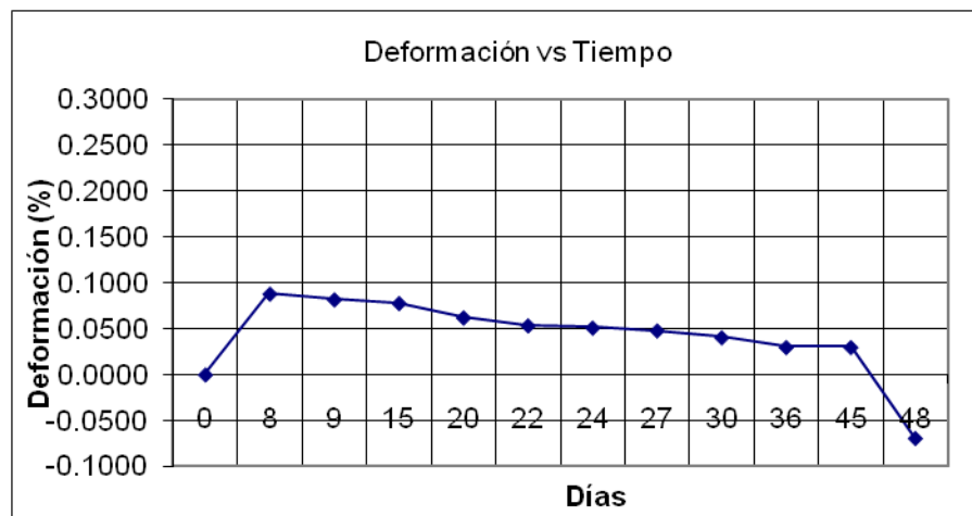
Grafico Contracción de Ensayo Patrón
