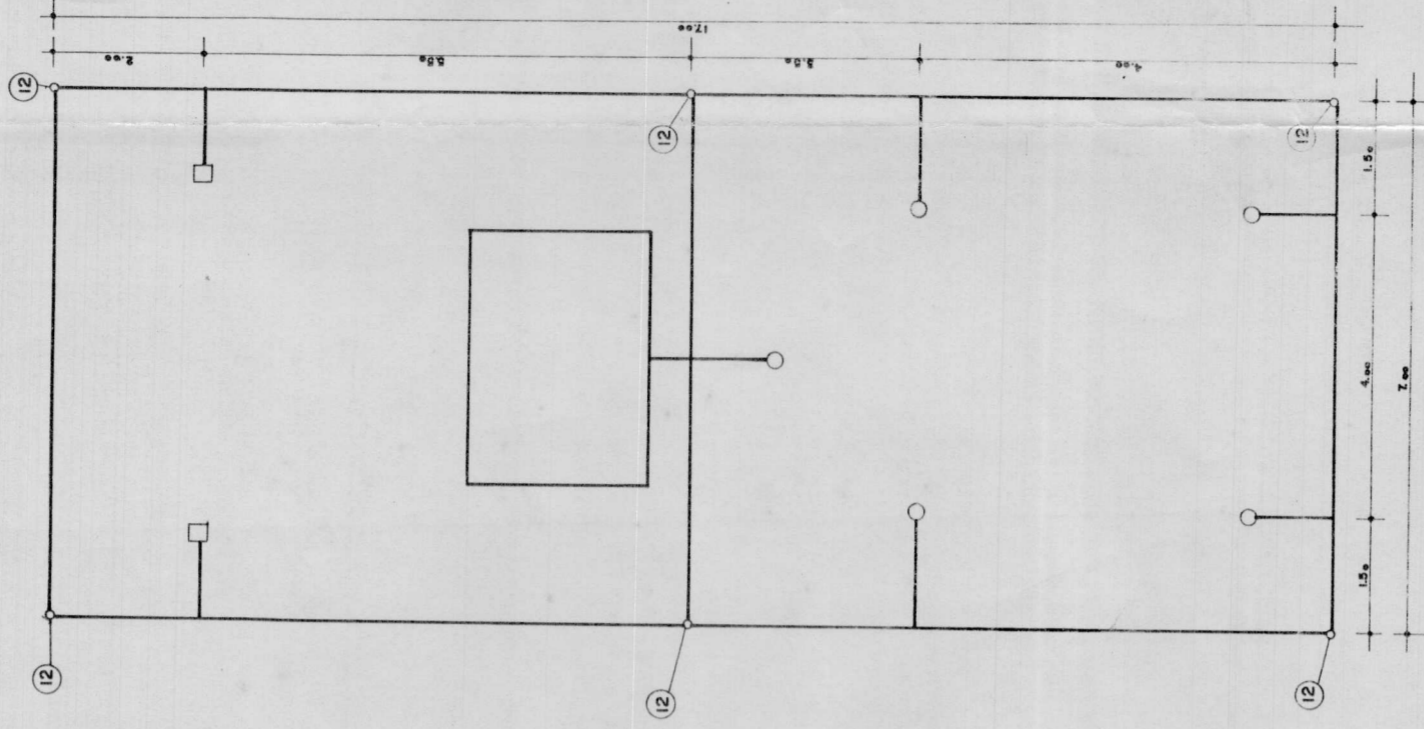
● malla de tierra esc. 1:30
