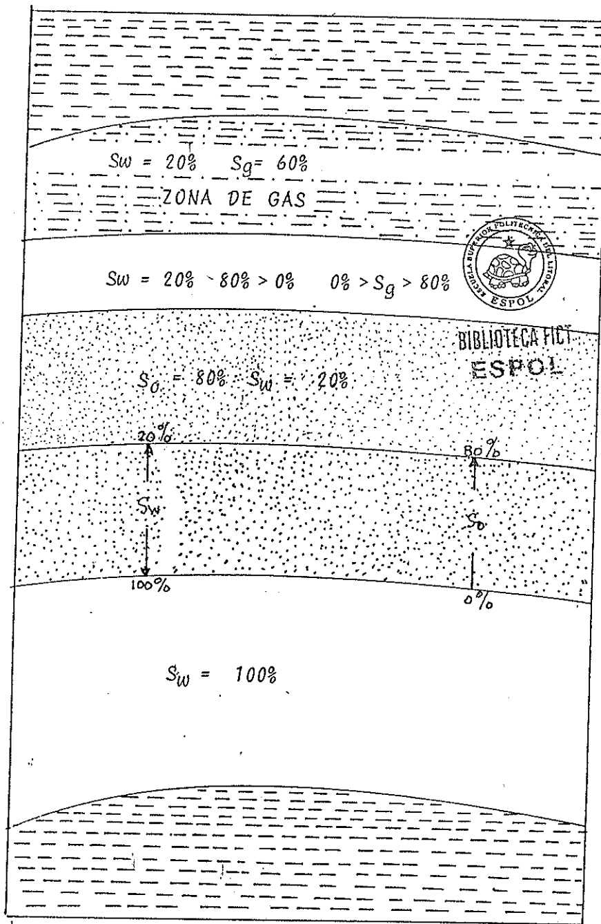
DISTRIBUCION IDEALIZADA DE LOS FLUIDOS EN EL YACIMIENTO
