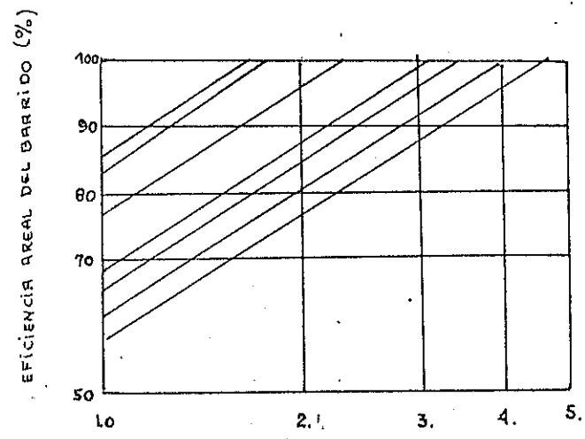
VOLUMEN INYECTADO ÷ VOLUMEN INYECTADO A LA RUPTURA. EFICIENCIA AREAL DEL BARRIDO EN FUNCION DEL VOLUMEN INYECTADO EXPRESADO EN VOLUMENES INYECTADOS A LA RUPTURA PARA UN ARREGLO DE 5 POZOS.
