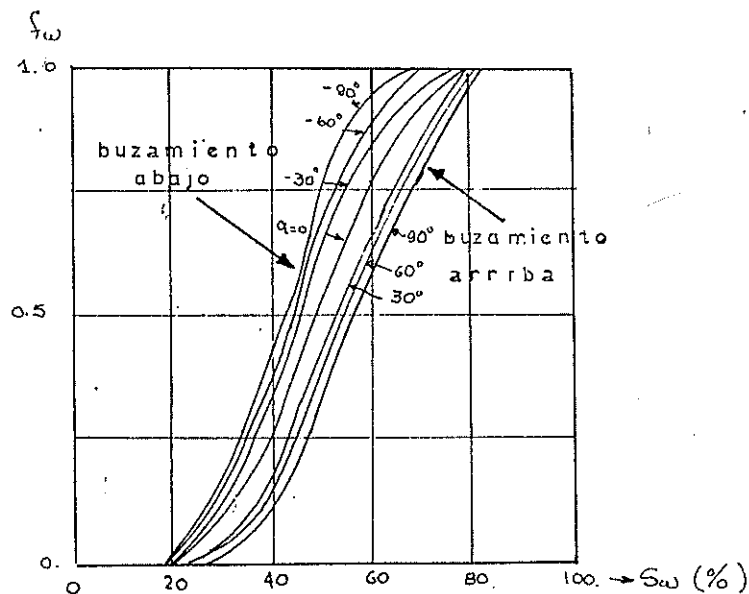
FLUJO FRACCIONAL DEL AGUA EN FUNCION DEL ANGULO \beta
