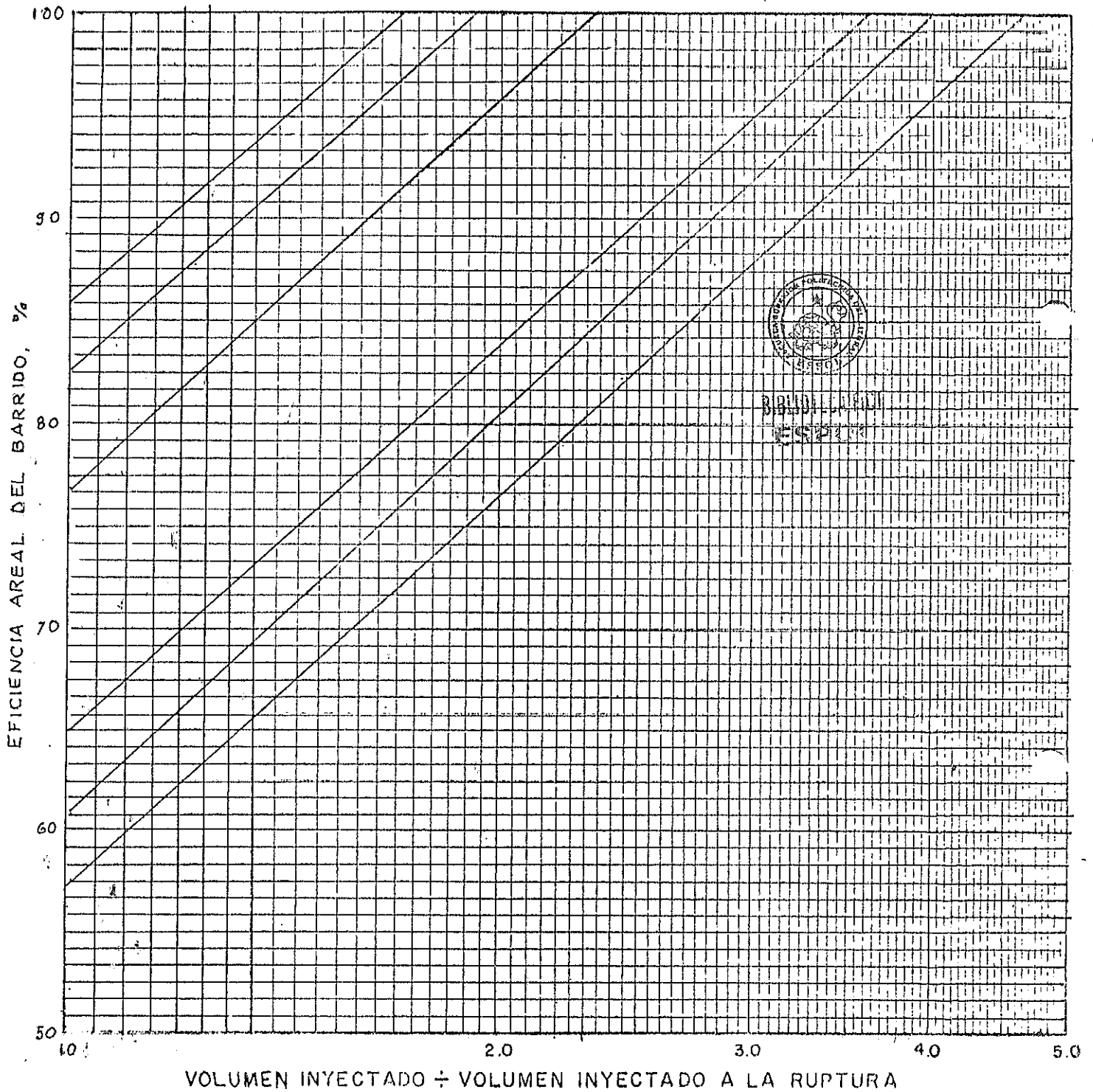
EFICIENCIA AREAL DEL BARRIDO EN FUNCIÓN DEL VOLUMEN INYECTADO EXPRESADO EN VOLÚMENES INYECTADOS A LA RUPTURA PARA UN ARREGLO DE 5 POZOS (TOMADO DE CRAIG Y ASOCIADOS (1)).
