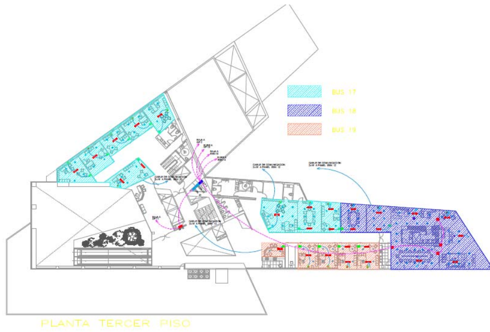
Figura 1.11: Plano Quantum Tercer Piso
