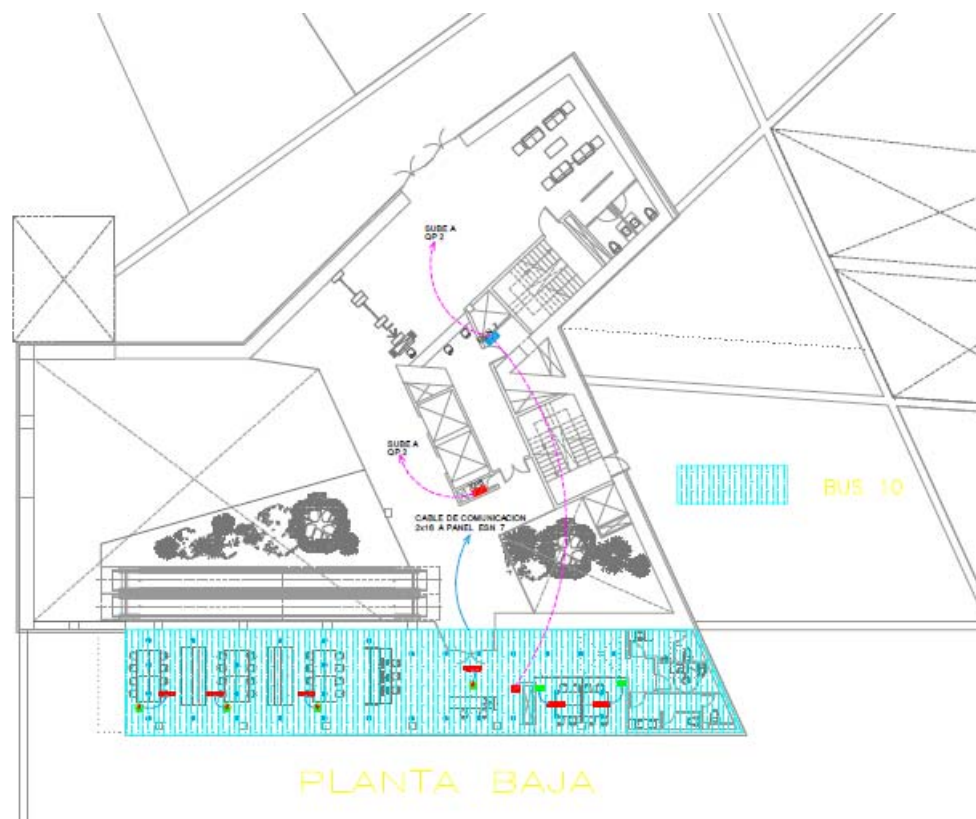
Figura 1.8: Plano Quantum Planta Baja.
