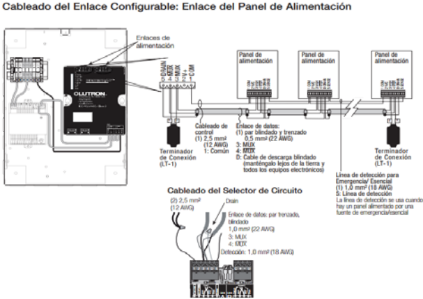
Figura 1.2: Enlace Paneles de Poder.
