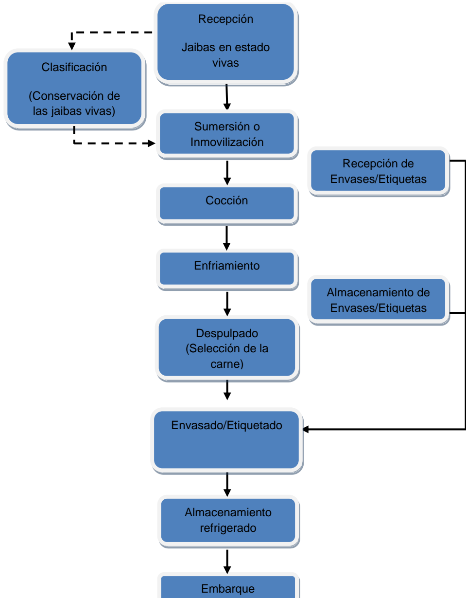
Figura N° 31 “Flujograma de proceso”
