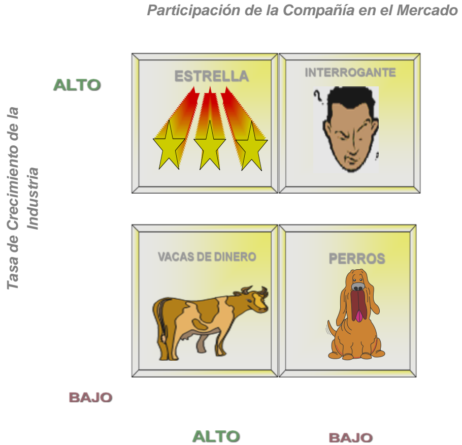
Figura N° 18 “Matriz BCG”
