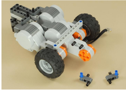
Figura 3-35: Robot Modelo Paso 12.2
