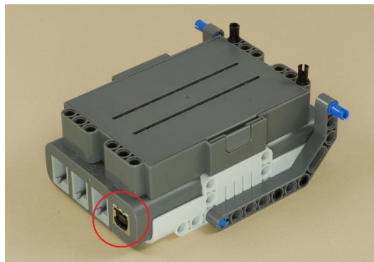
Figura 3-40: Robot Modelo Paso 13.3
