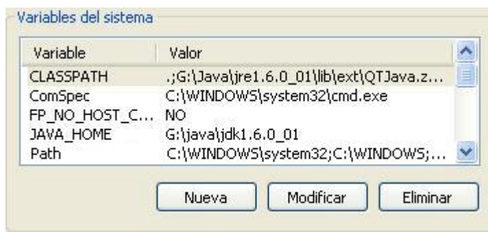
Figura 42: Variables de ambiente para J2SDK
