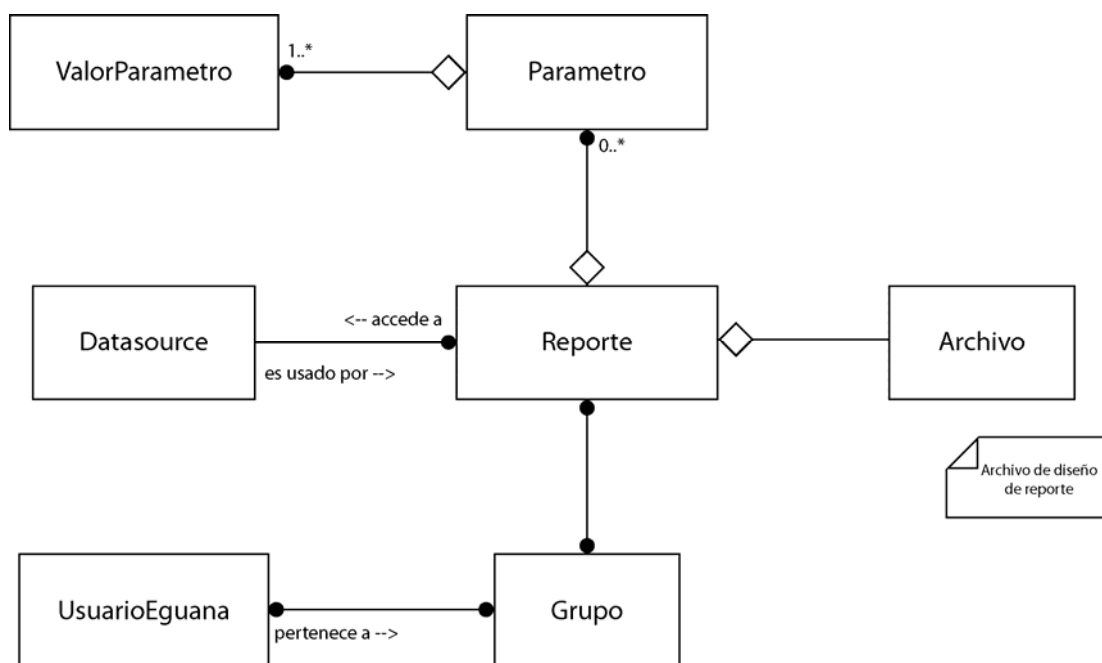
Figura 7: Diagrama simplificado de objetos
