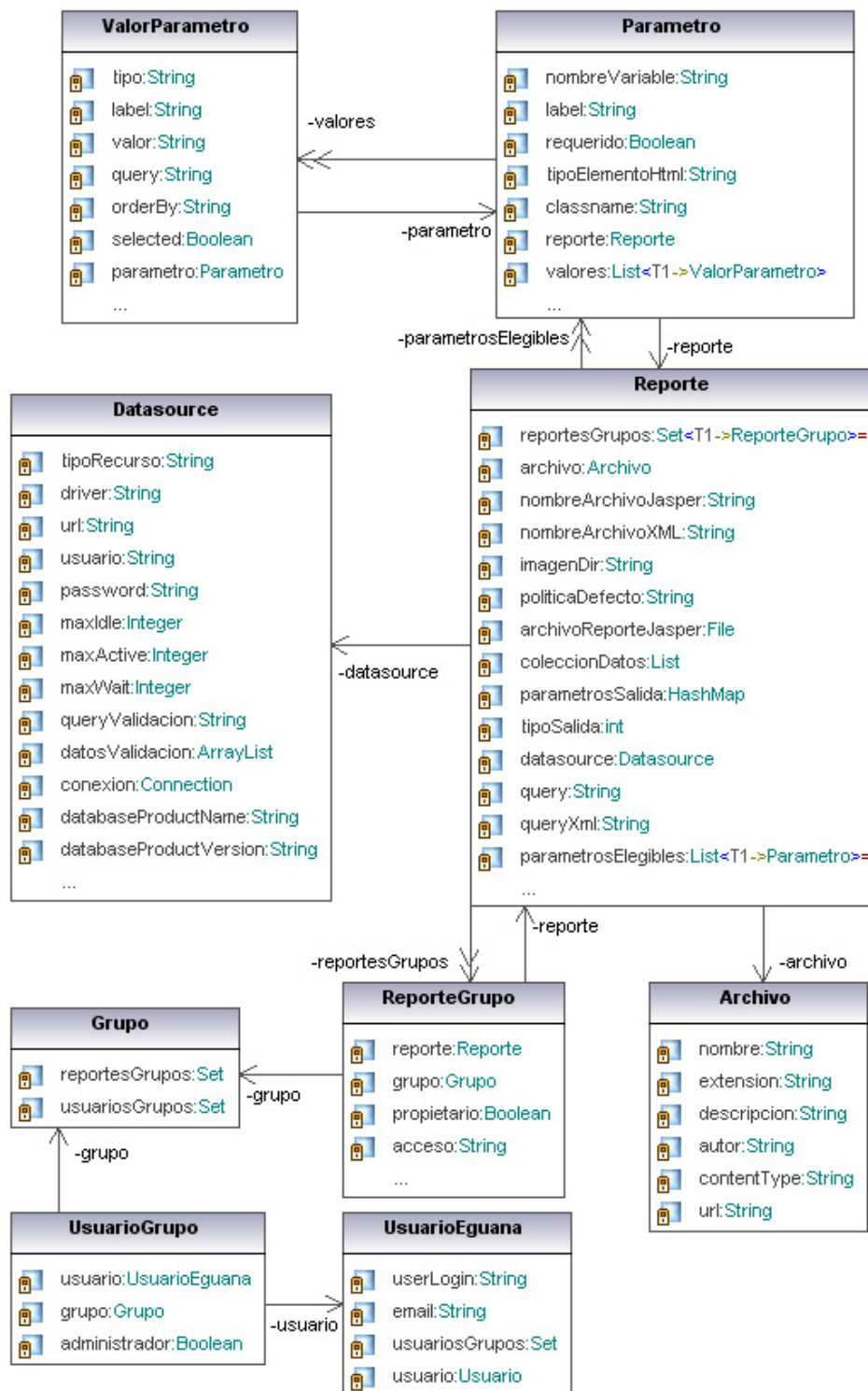
Figura 8: Diagrama de clases
