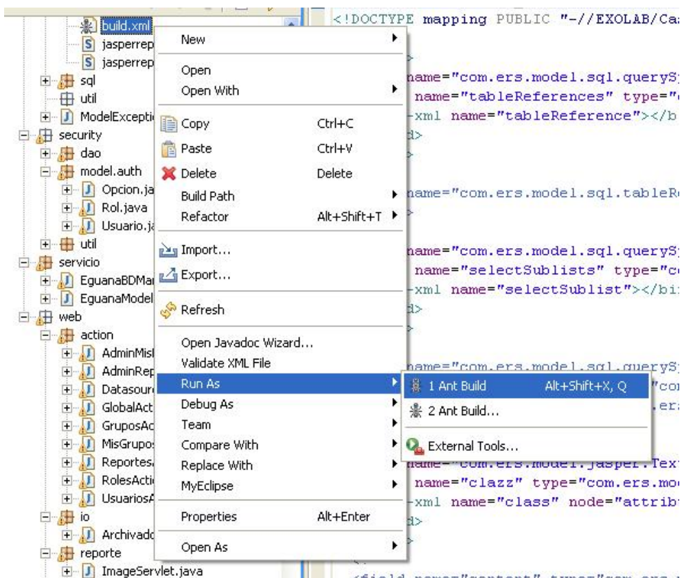
Figura 50: Ejecutando la tarea de Ant para Castor
