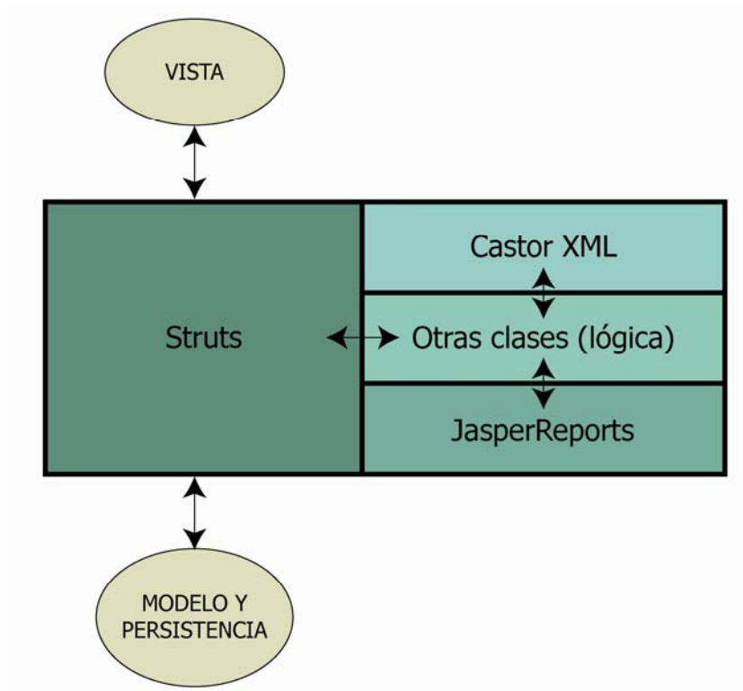
Figura 26: Capa de lógica y control
