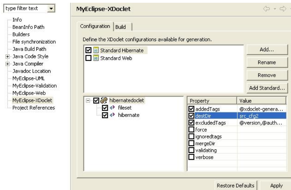
Figura 47: Configuración de MyEclipse-XDoclet para Hibernate
