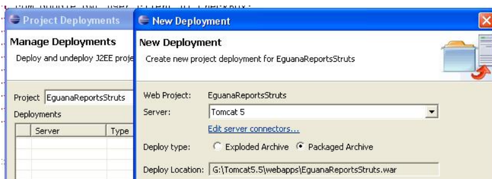
Figura 54: Creación de .war y despliegue en Tomcat
