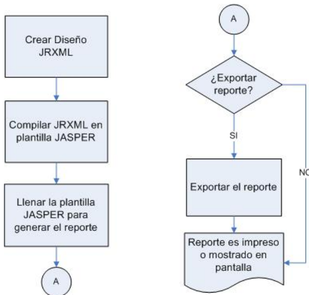
Figura 35: Diagrama de flujo para crear reportes en JasperReports
