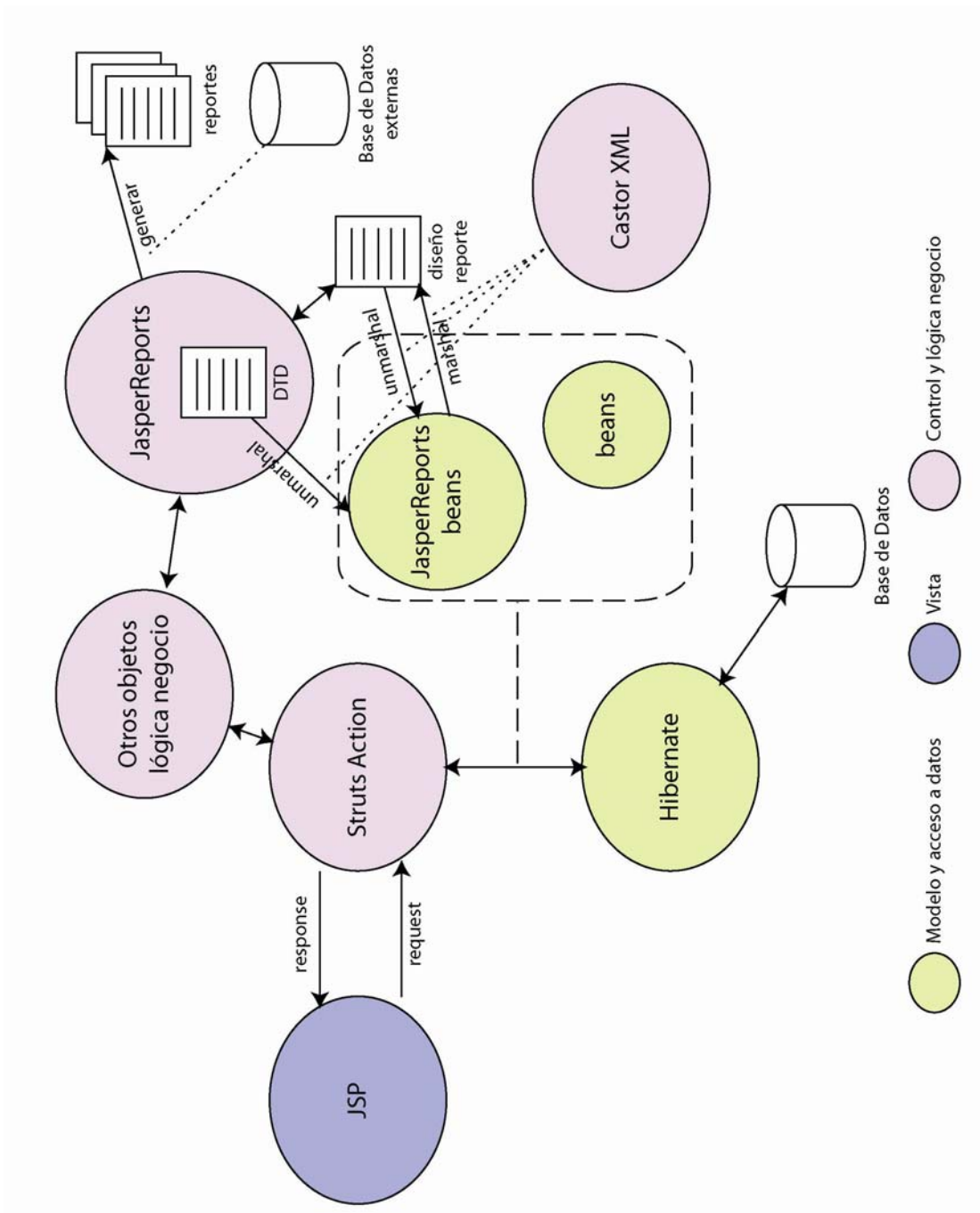
Figura 27: Tecnologías en arquitectura MVC de Eguana Reports
