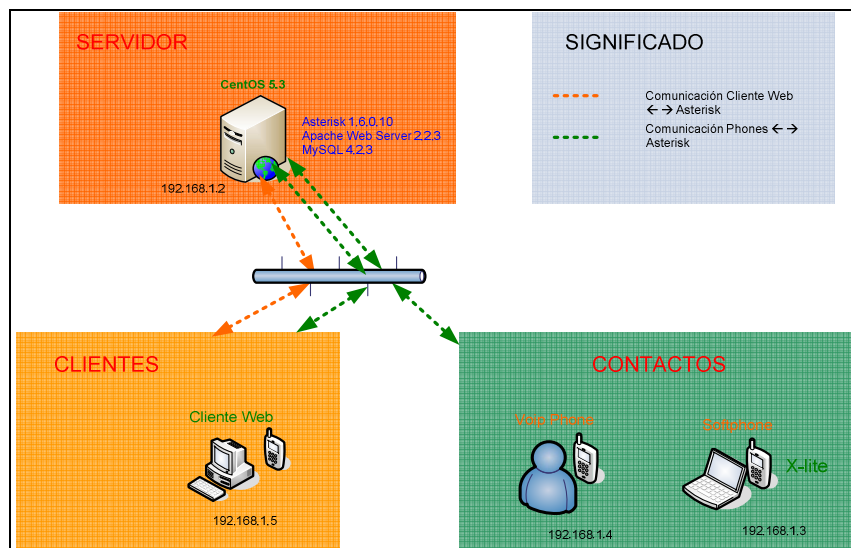
Figura 3.3 Diseño de red.
