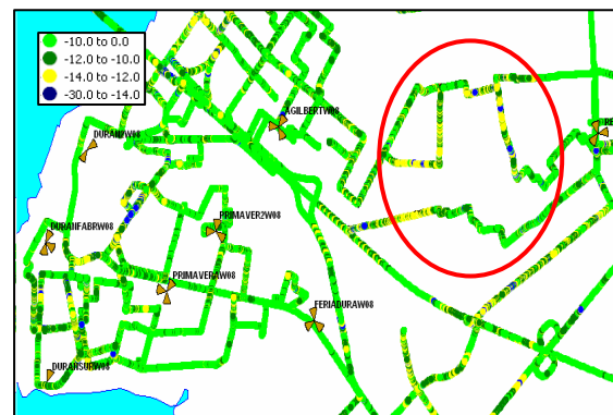
Figura 4.3 Plot Ec/Io
