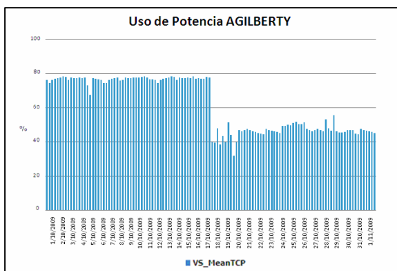
Figura 4.21 Uso de potencia AGILBERTY
