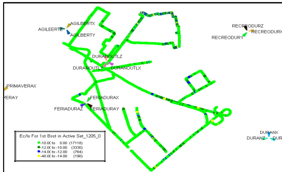
Figura 4.18 Plot Ec/Io con cambios
