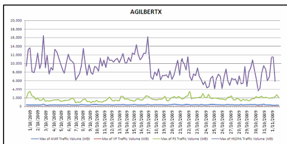
Figura 4.20 Tráfico AGILBERTX
