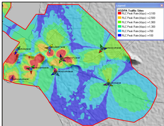
Figura 4.16 HSDPA con el nuevo Nodo B
