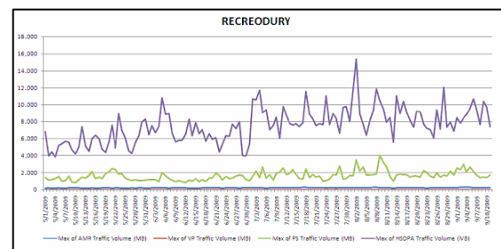
Figura 4.9 Tráfico RECREODURY
