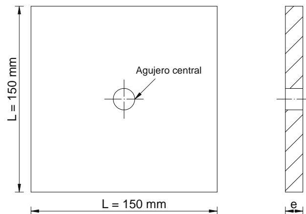
FIG. 4.11 PLACA PORTAPESAS.
