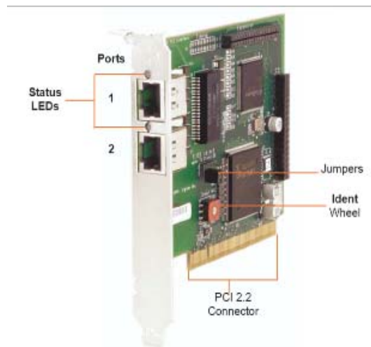
Figura 2.6 Tarjeta TE205P
