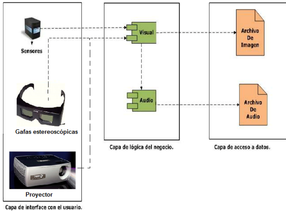
Fig. 13: Nivel de Interface Gráfica con el usuario
