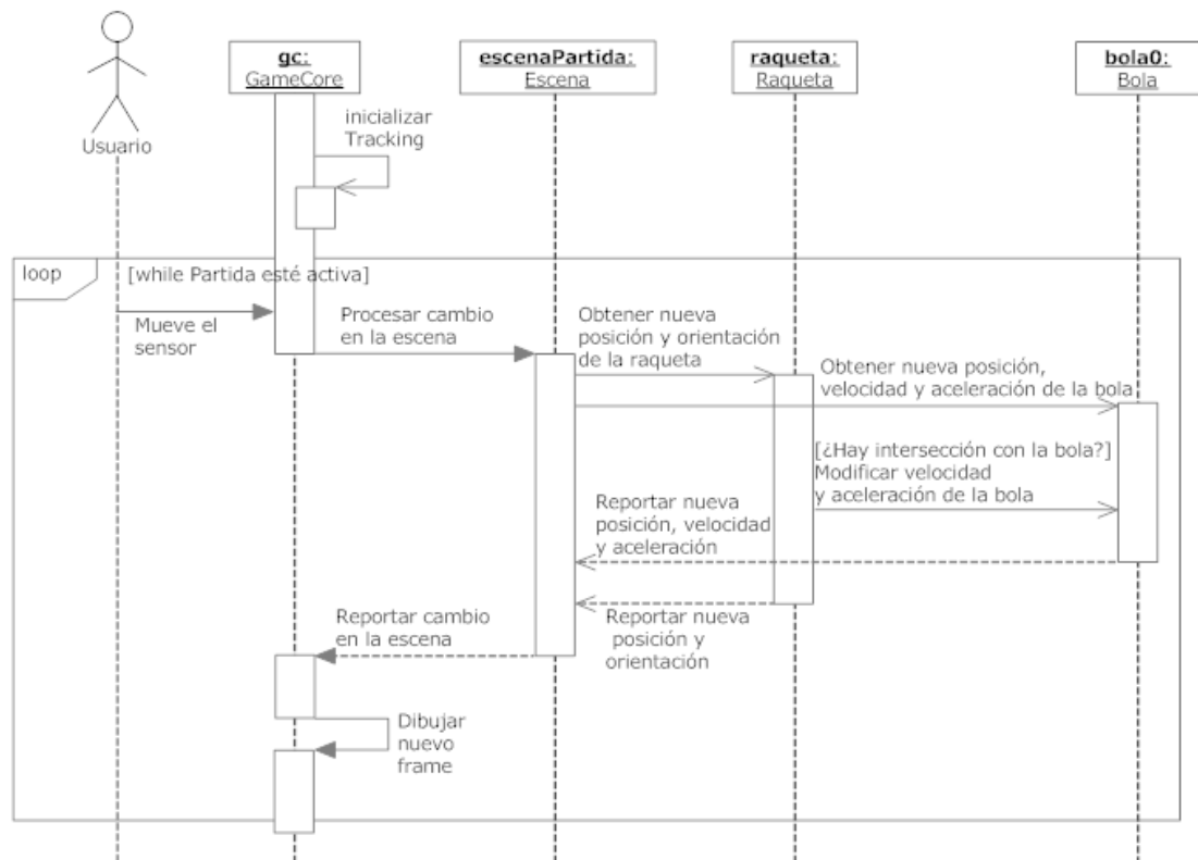
Fig. 19: Diagrama de interacción de objetos del caso de uso 2
