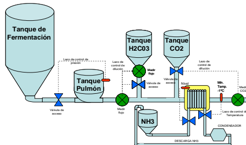
Figura 1.- flujograma para el proceso de dilución de cerveza.
