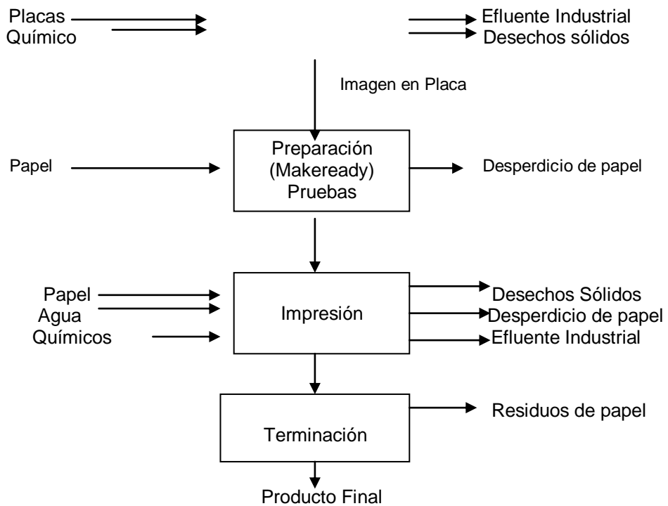
FIGURA 3.1 DIAGRAMA DEL PROCESO OFFSET
