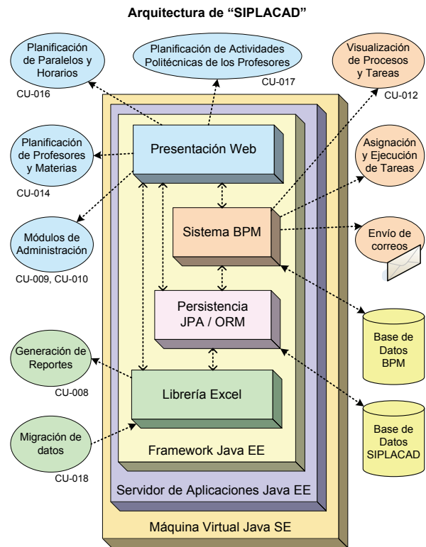
Figura 2. Arquitectura del sistema
