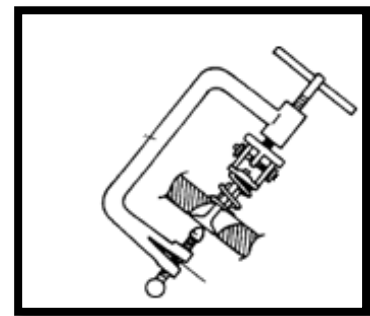
Fig. 3.2 Extracción de Válvulas
