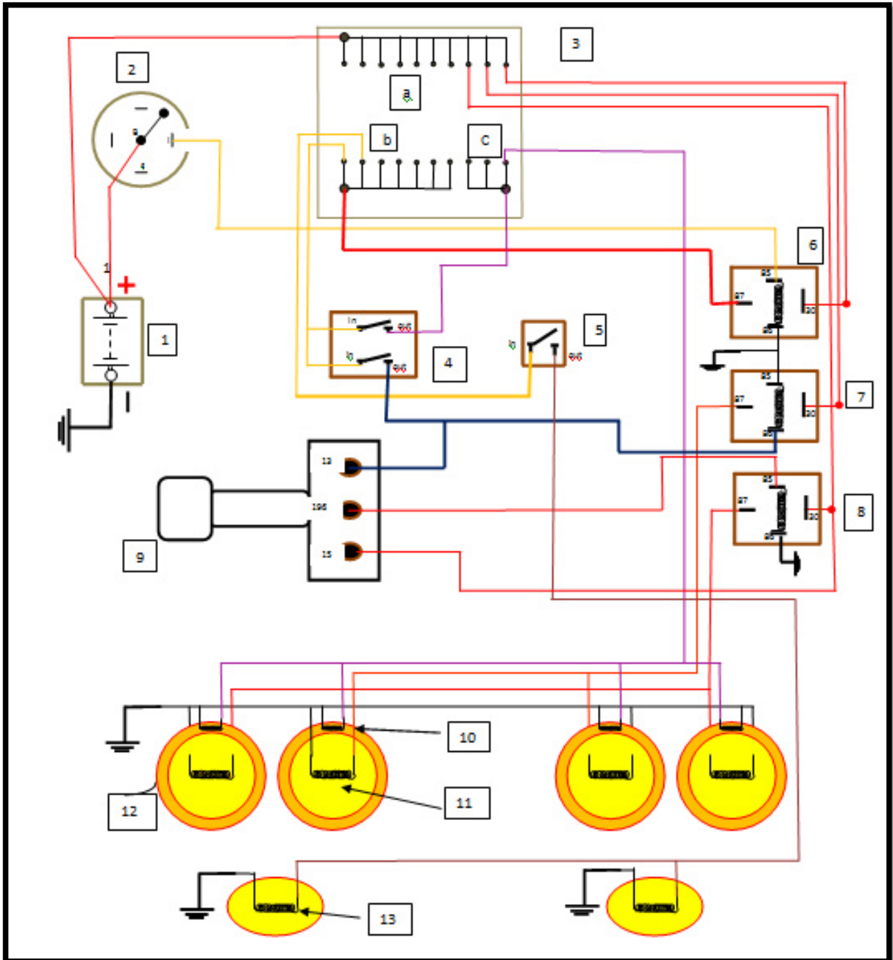
Diagra 1: Diagrama de luces Altas, Bajas, guías y neblineros del vehículo.
