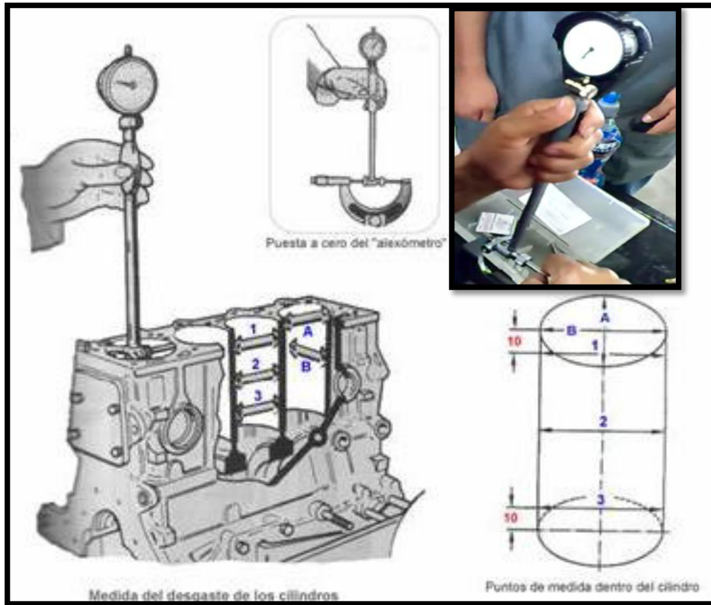
Fig. 3.5 Inspección de Cilantros
