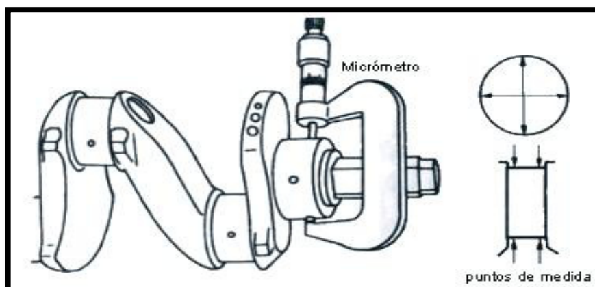
Fig. 3.7 Medición del Cigüeñal.
