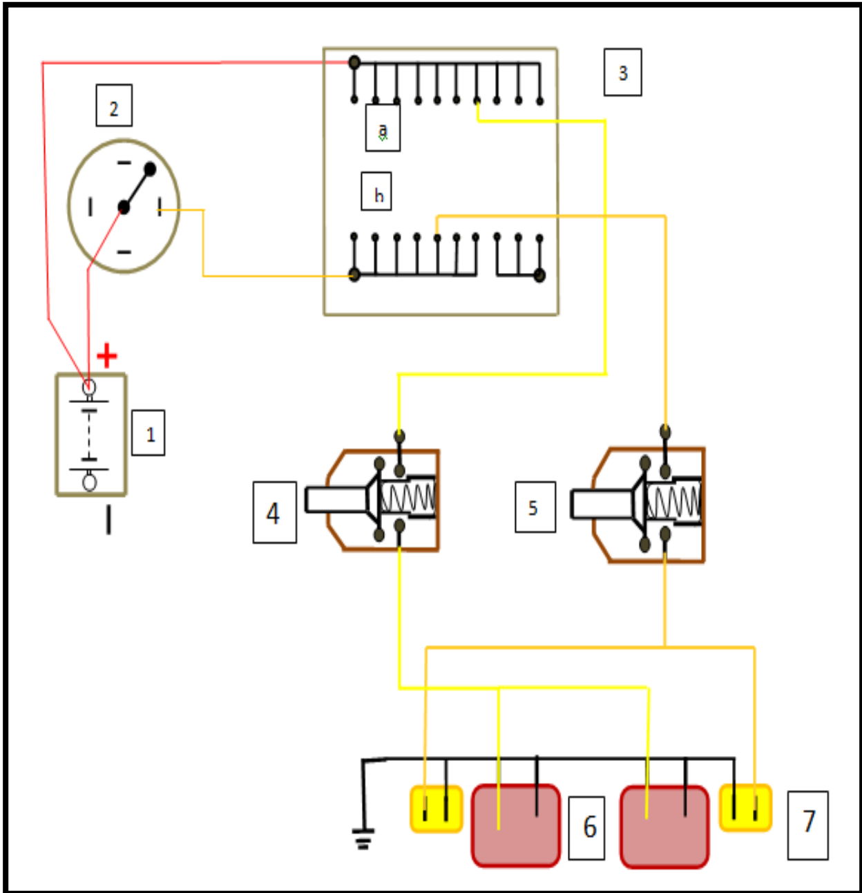
Diagrama 5.2. Diagrama de Luces Stop, Retro del vehículo
