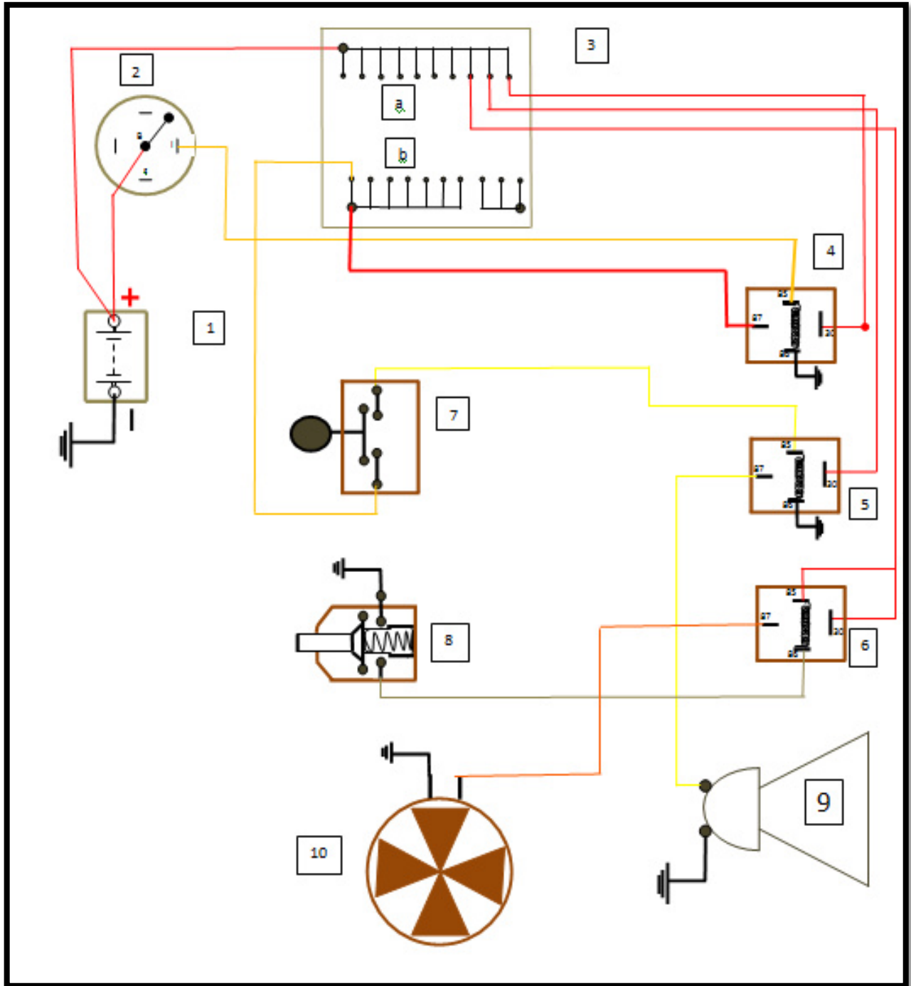
Diagrama 5.3: Diagrama del Electro ventilador y Pito
