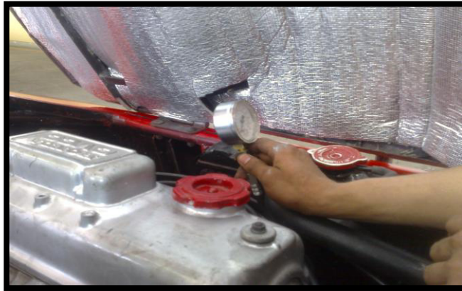
Fig. 3.14 Medición de la Compresión.
