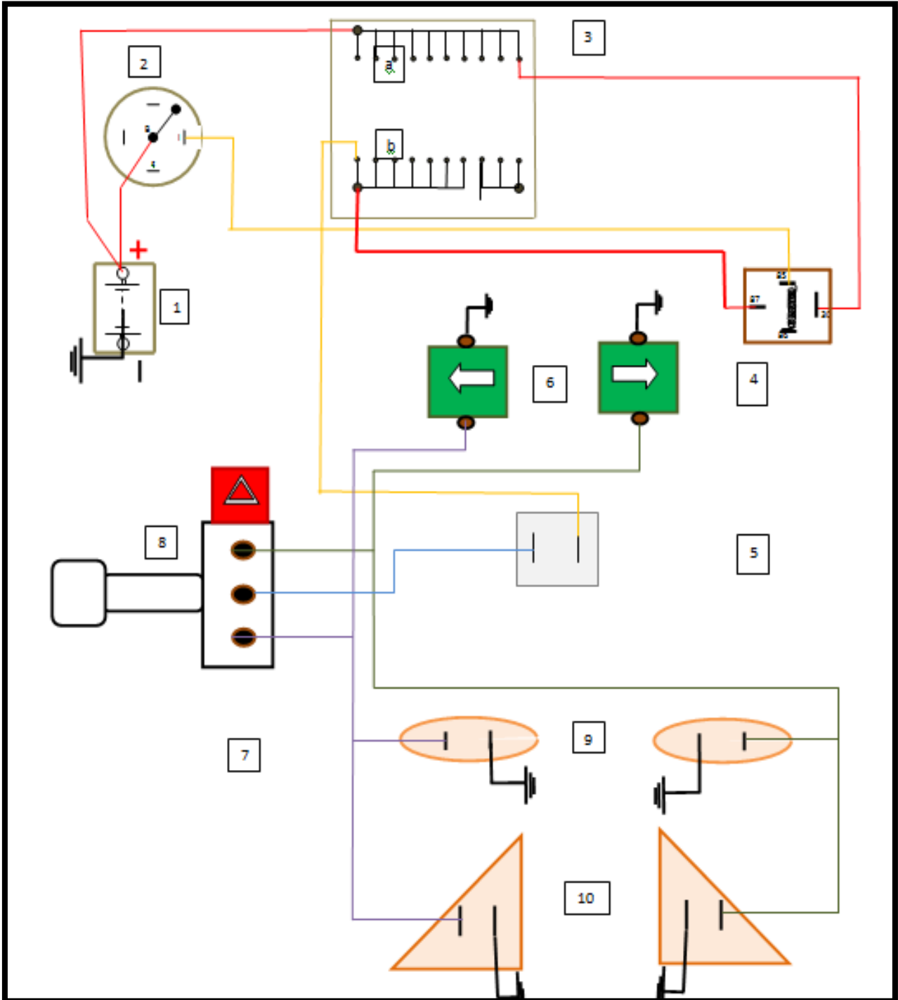
Diagrama5.5: Diagrama de luces Direccionales y de Parqueo del vehículo
