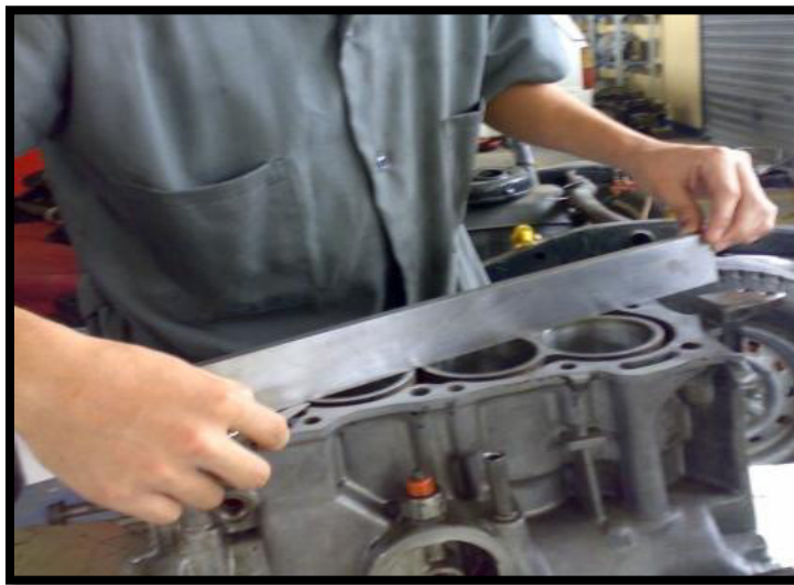
Fig. 3.4 Inspección Bloque de Cilindros.
