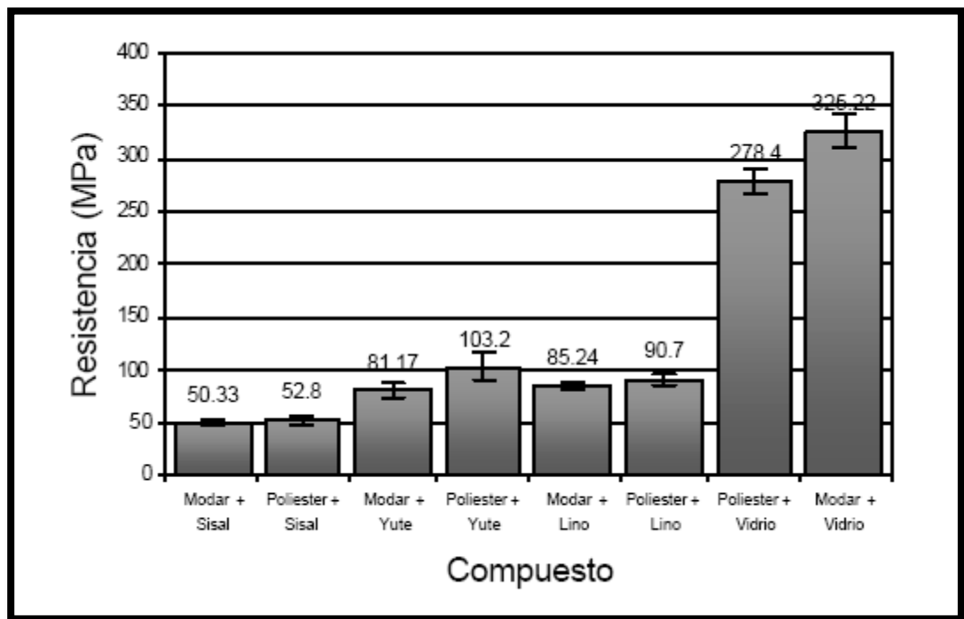
Grafico 6. Resistencia de Flexión
