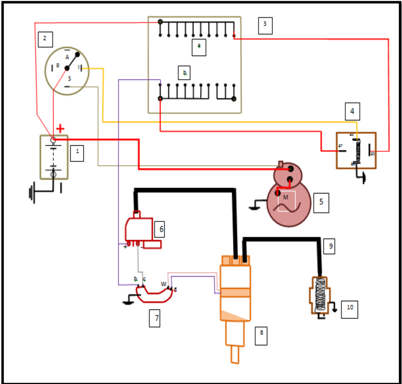
Diagrama 5.6. Diagrama del sistema de arranque y encendido del vehículo
