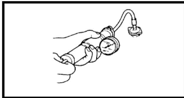
Fig.3.17 Prueba de Fuga de Agua.
