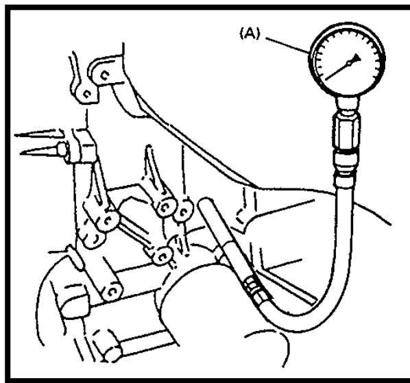
Fig.3.16 Medición de la presión del Aceite.
