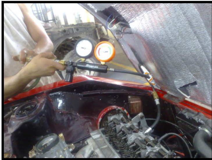
Fig. 3.15 Comprobación de Fugas.
