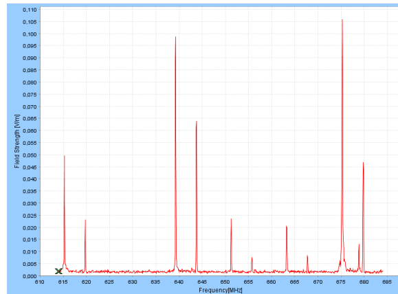
Figura 1.18 Espectro TV Abierta 644-686 MHz. 25
