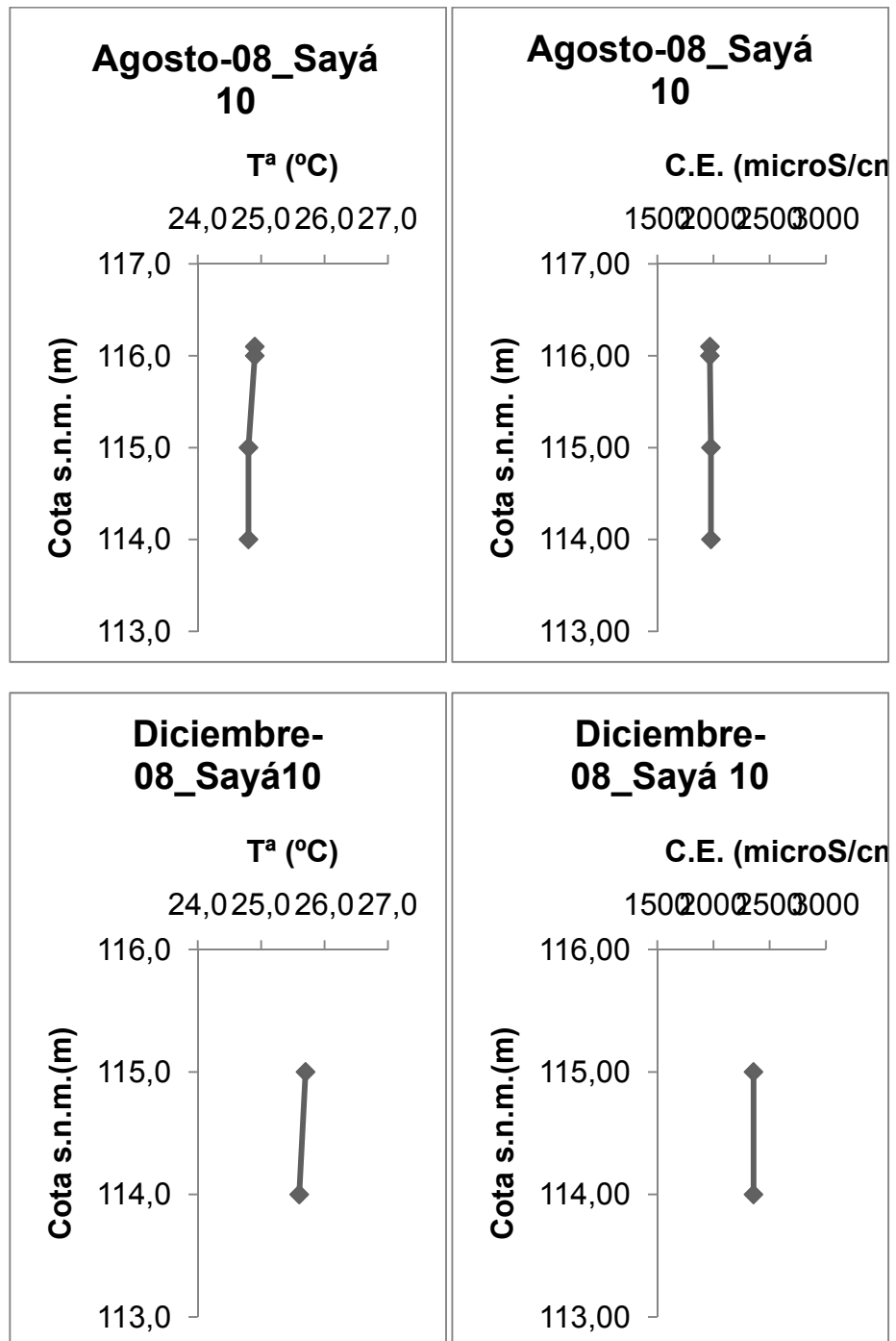
Figura A3.18. Perfiles de temperatura y conductividad eléctrica en el interior de los sondeos pozó Sayá 10.
