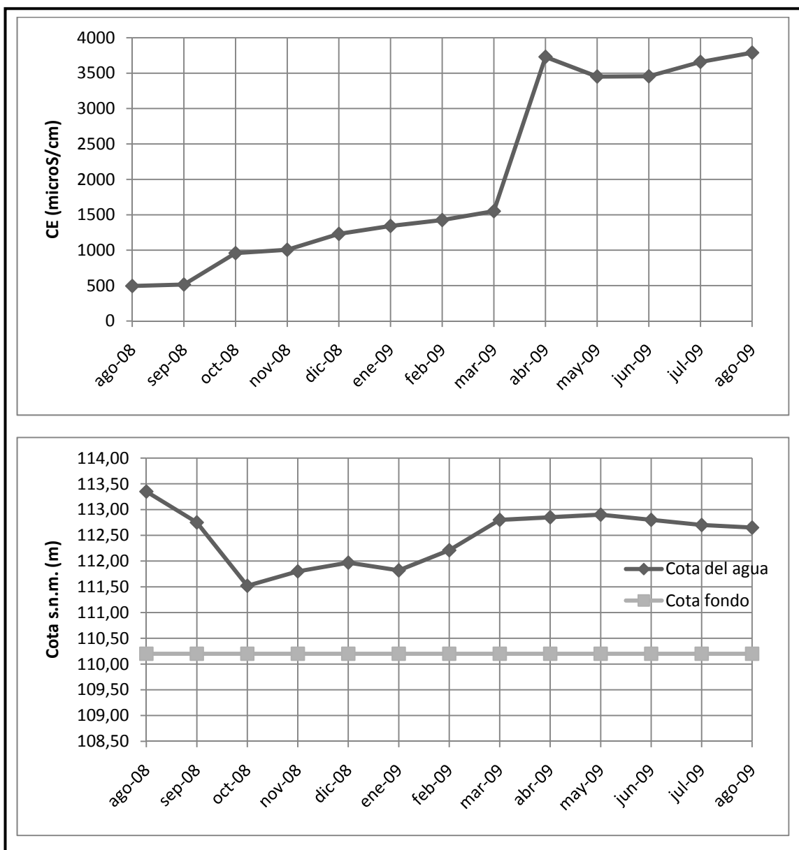
Figura A2.6. Evolución temporal del nivel piezométrico, profundidad, y conductividad eléctrica en el pozo Sayà 6.
