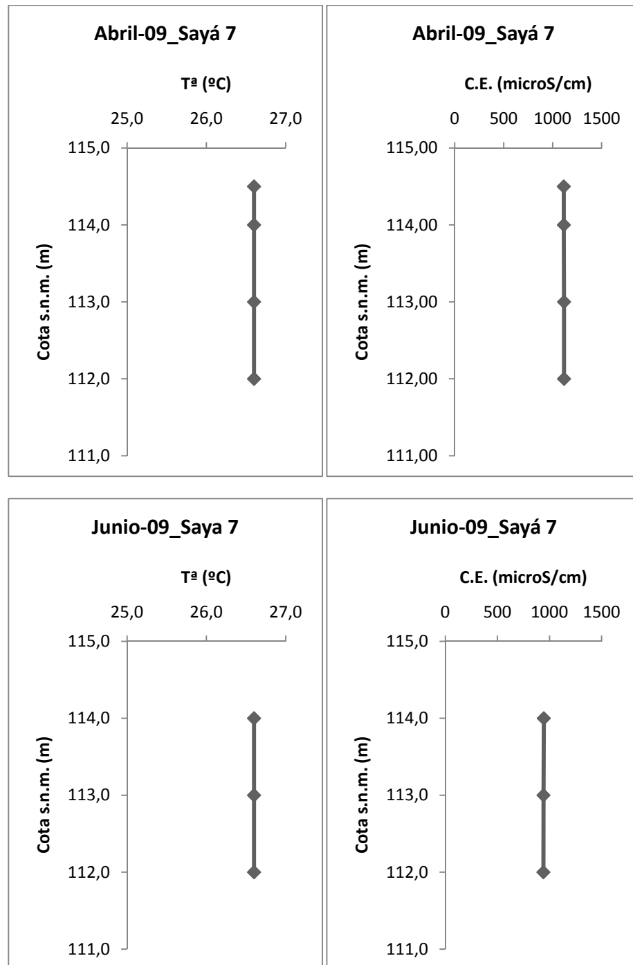
Figura A3.14. Perfiles de temperatura y conductividad eléctrica en el interior de los sondeos pozó Sayá 7.
