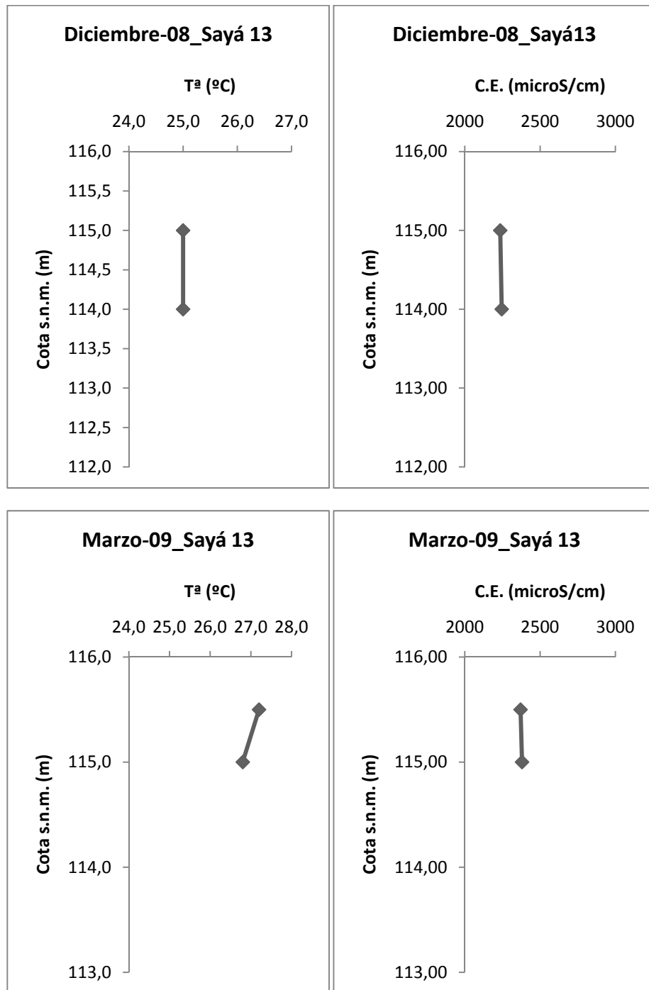
Figura A3.23. Perfiles de temperatura y conductividad eléctrica en el interior de los sondeos pozó Sayá 13.
