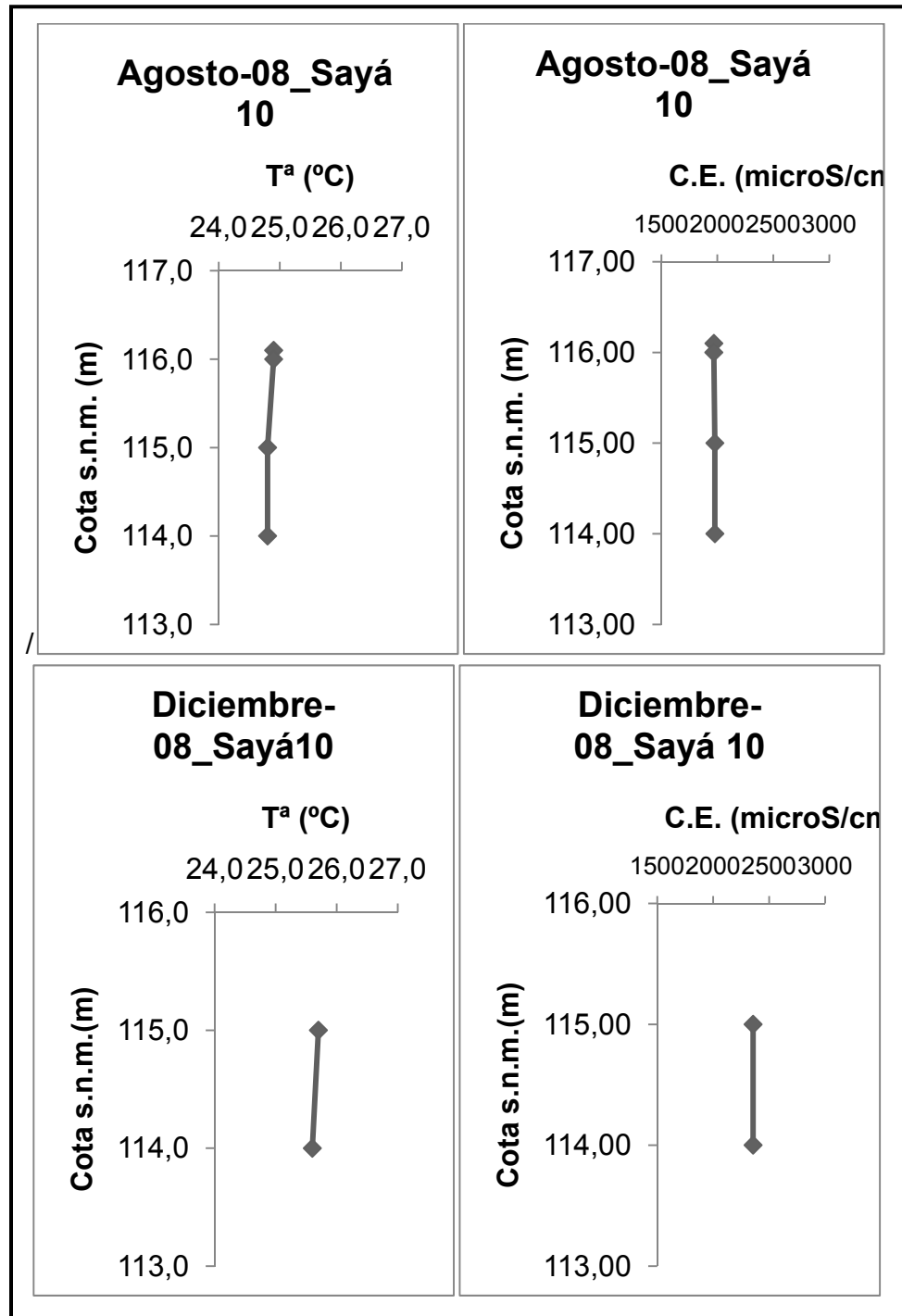
Figura A3.18. Perfiles de temperatura y conductividad eléctrica en el Sayá10.
