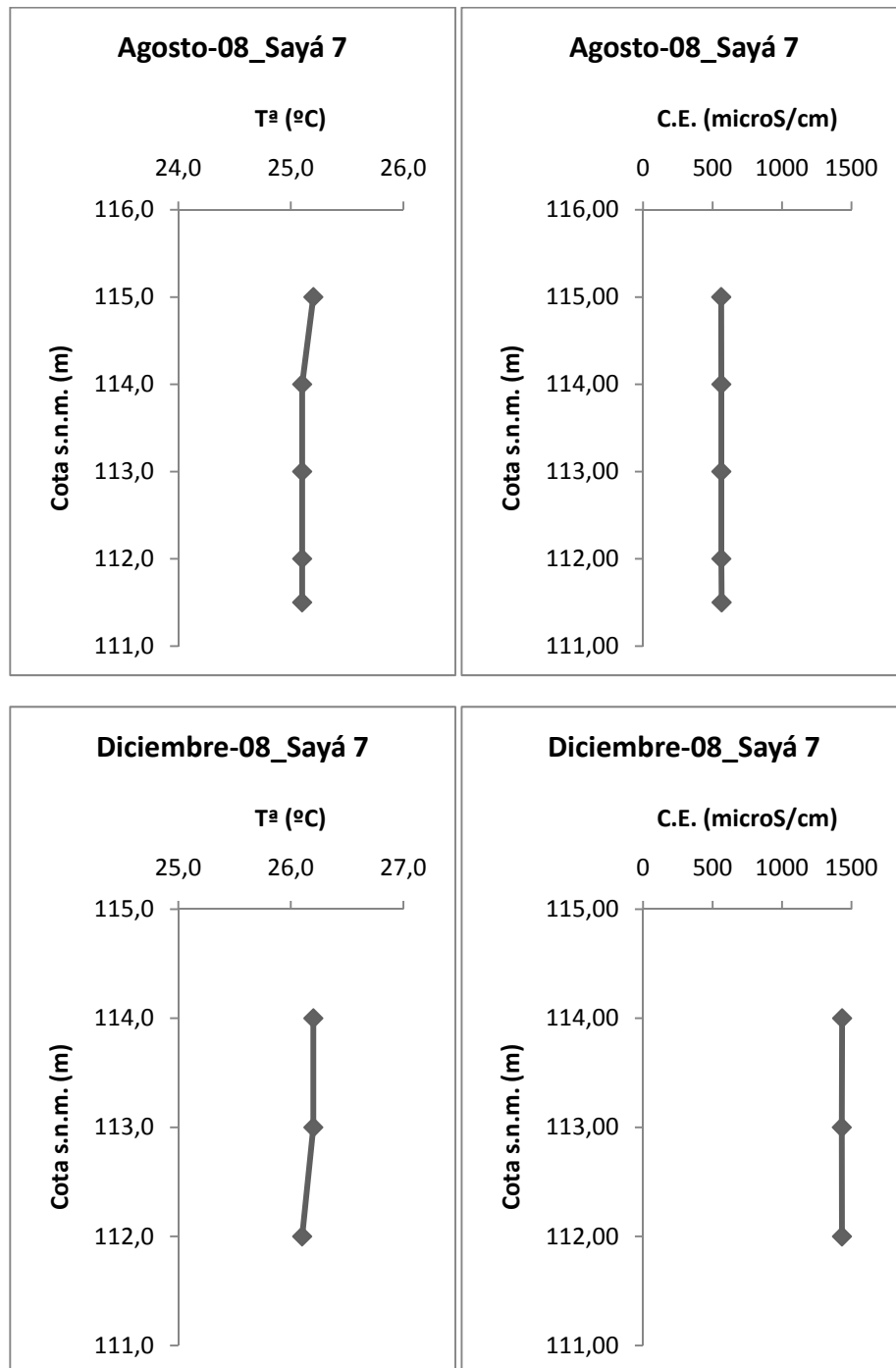
Figura A3.13. Perfiles de temperatura y conductividad eléctrica en el interior de los sondeos pozó Sayá 7.
