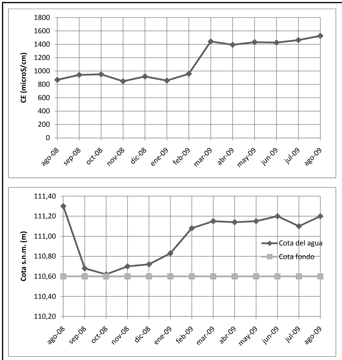
Figura A2.4. Evolución temporal del nivel piezométrico, profundidad, y conductividad eléctrica en el pozo Sayá 4.
