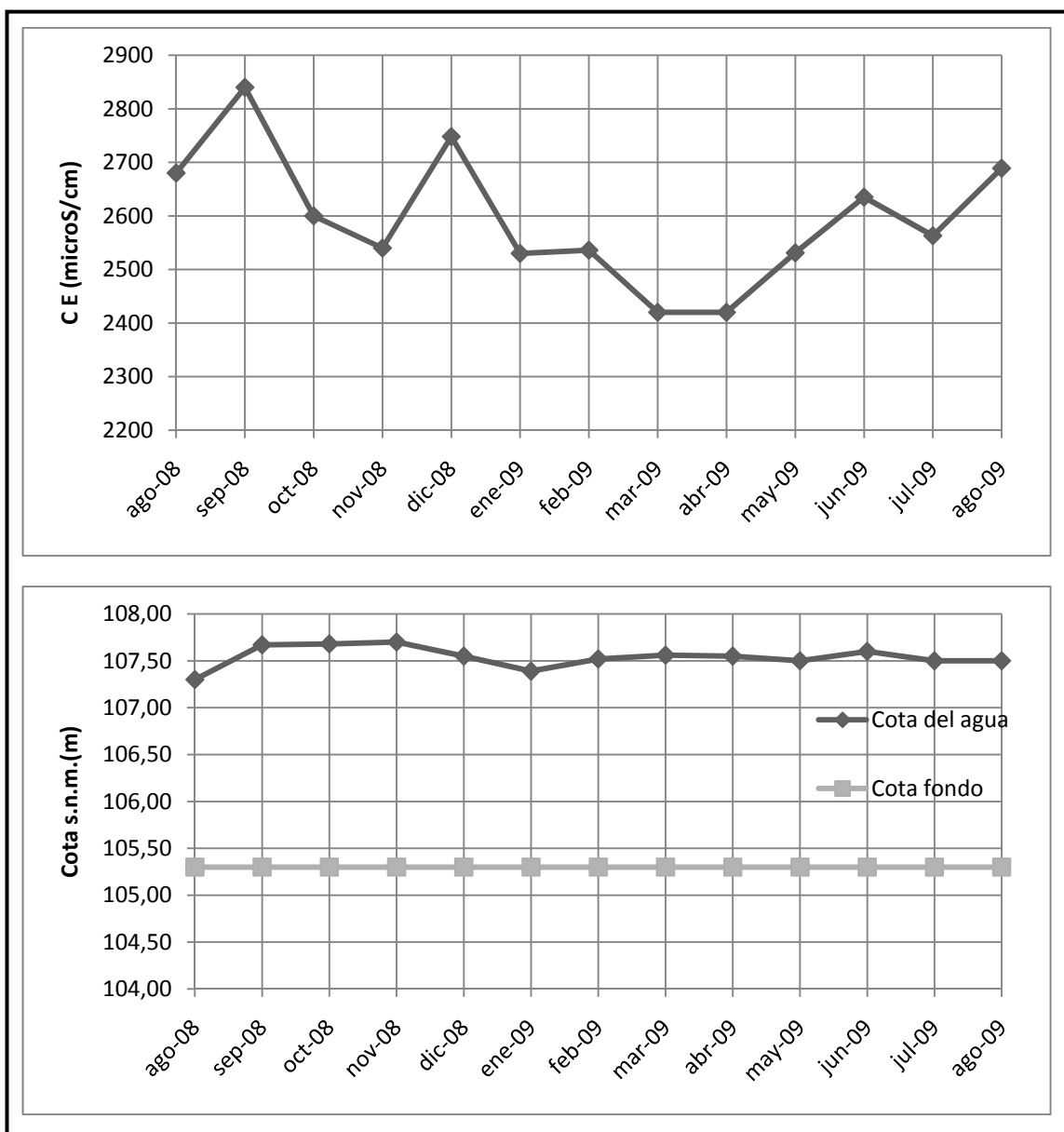
Figura A2.1. Evolución temporal del nivel piezométrico, profundidad, y conductividad eléctrica en el pozo Sayá 1.
