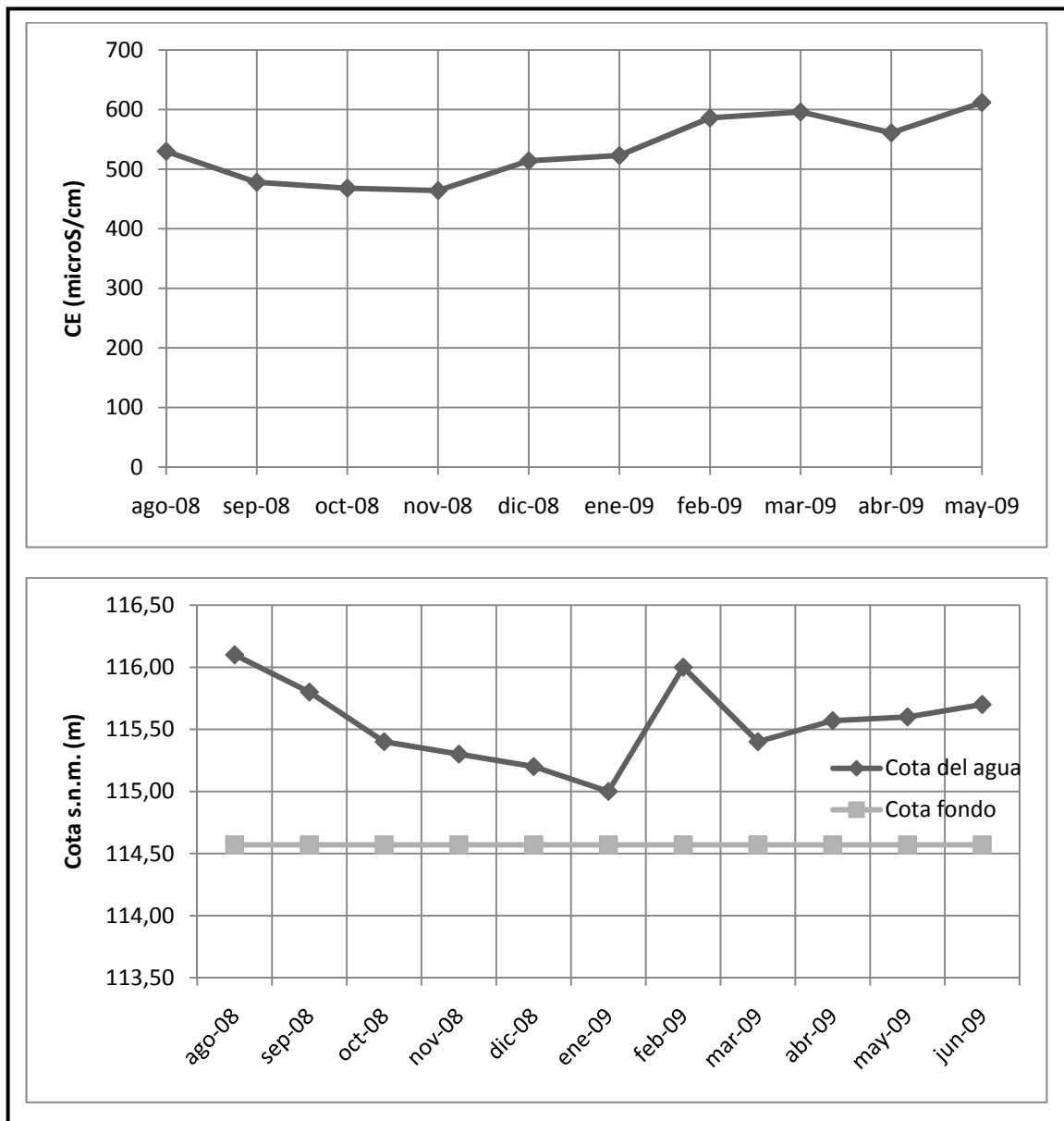
Figura A2.12. Evolución temporal del nivel piezométrico, profundidad, y conductividad eléctrica en el pozo 12.
