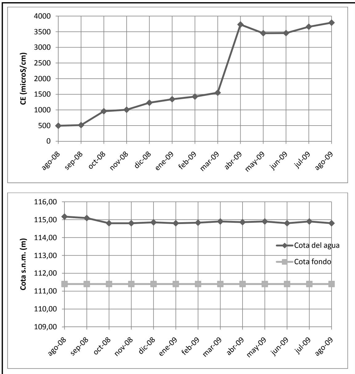
Figura A2.7. Evolución temporal del nivel piezométrico, profundidad, y conductividad eléctrica en el pozo Sayá 7
