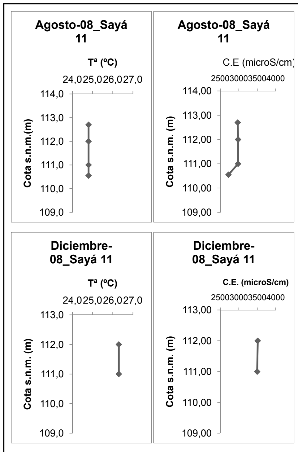
Figura A3.20. Perfiles de temperatura y conductividad eléctrica pozo Sayá 11.
