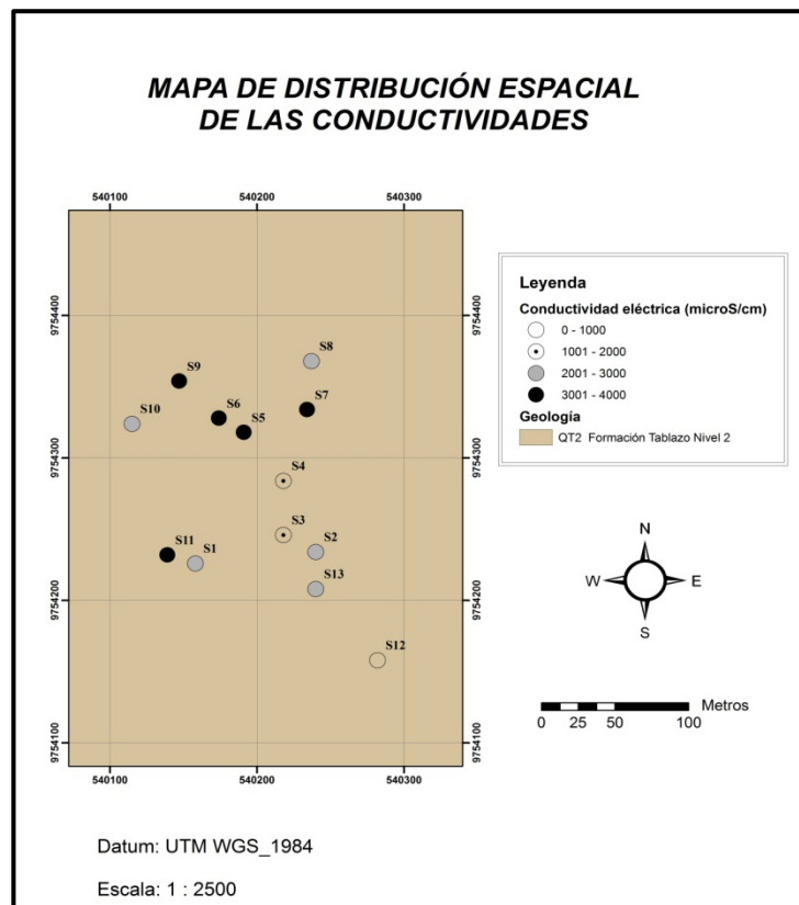
Figura 3.8 Distribución de las conductividades eléctricas máximas ( \mu\text{S}/\text{cm} ) alcanzadas en las captaciones de la red de control en el área de la población de Sayá.
