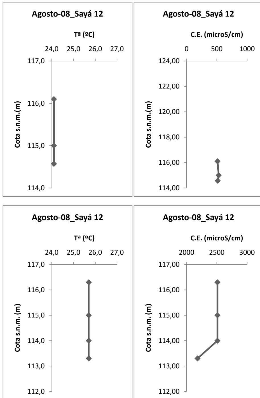
Figura A3.22. Perfiles de temperatura y conductividad eléctrica en el interior de los sondeos pozó Sayá 12.
