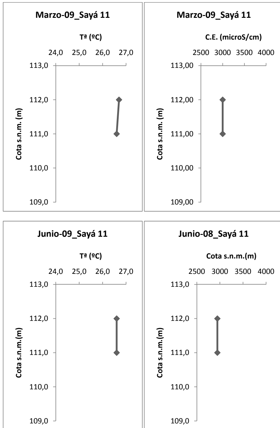
Figura A3.21. Perfiles de temperatura y conductividad eléctrica en el interior de los sondeos pozó Sayá 11.
