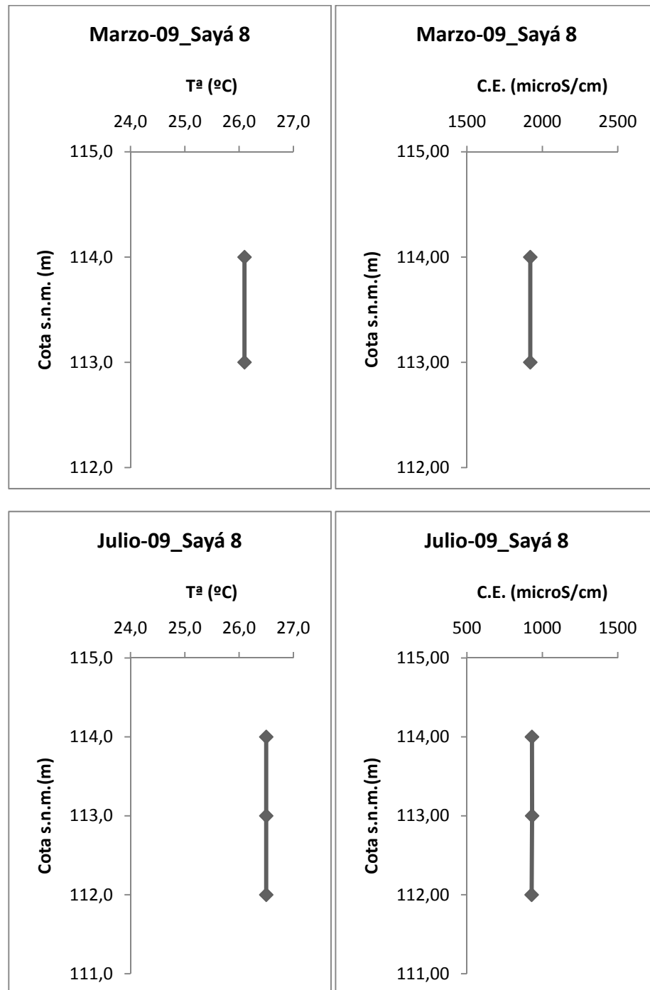
Figura A3.16. Perfiles de temperatura y conductividad eléctrica en el interior de los sondeos pozó Sayá 8.
