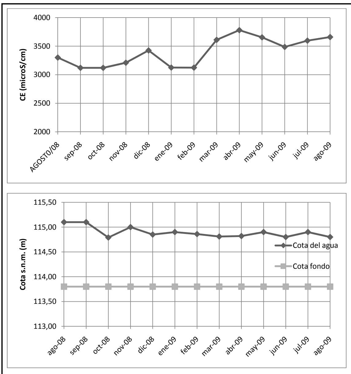
Figura A2.9. Evolución temporal del nivel piezométrico, profundidad, y conductividad eléctrica en el pozo Sayá 9.
