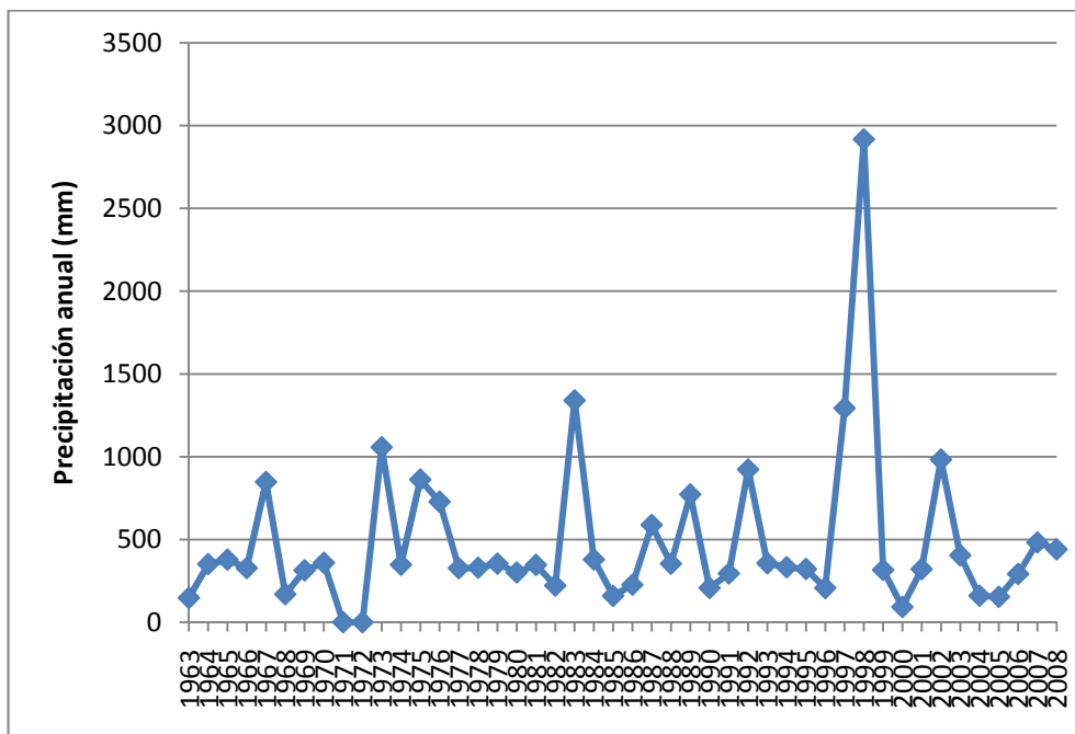
Figura. 3.4. Precipitaciones Anuales en el Área de la estación Manglaralto. (ESPOL-OIEA, 2006, ECU/8/026)
