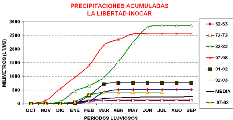
Figura. 3.5. Precipitaciones Acumuladas La Libertad – INOCAR. (Gálvez H., Regalado J., 2010)
