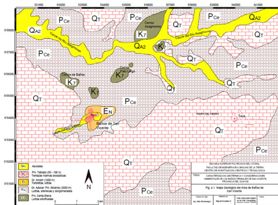
Figura 2.2. Mapa geológico de la comunidad de Sayá. (Gonzales M., 2003)
