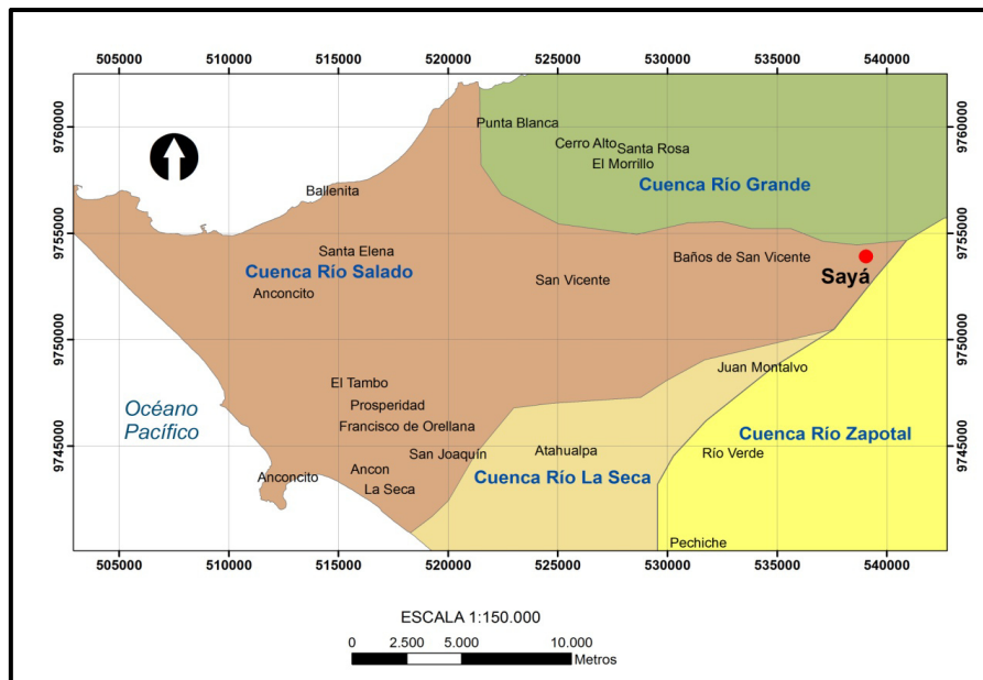
Figura 1.3. Delimitación de las principales cuencas hidrográficas de la zona de estudio. (ESPOL-OIEA, 2006, ECU/8/026)
