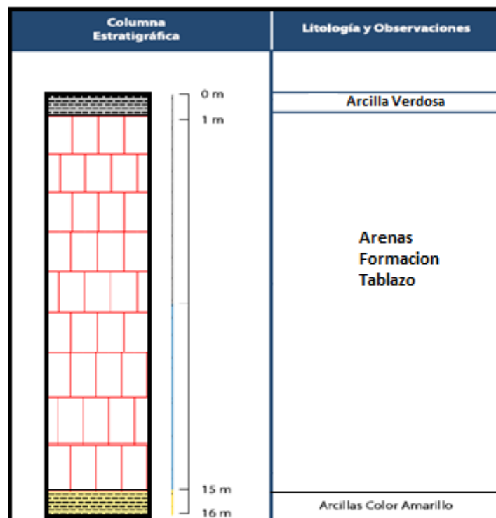
Figura 3.2. Columna Litológica pozo de observación de Sayá. (ESPOL-OIEA, 2006, ECU/8/026)
