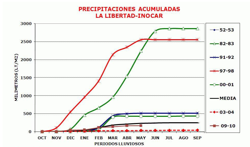
Figura. 3.6. Precipitaciones Acumuladas La Libertad – INOCAR. (Gálvez H., Regalado J., 2010)
