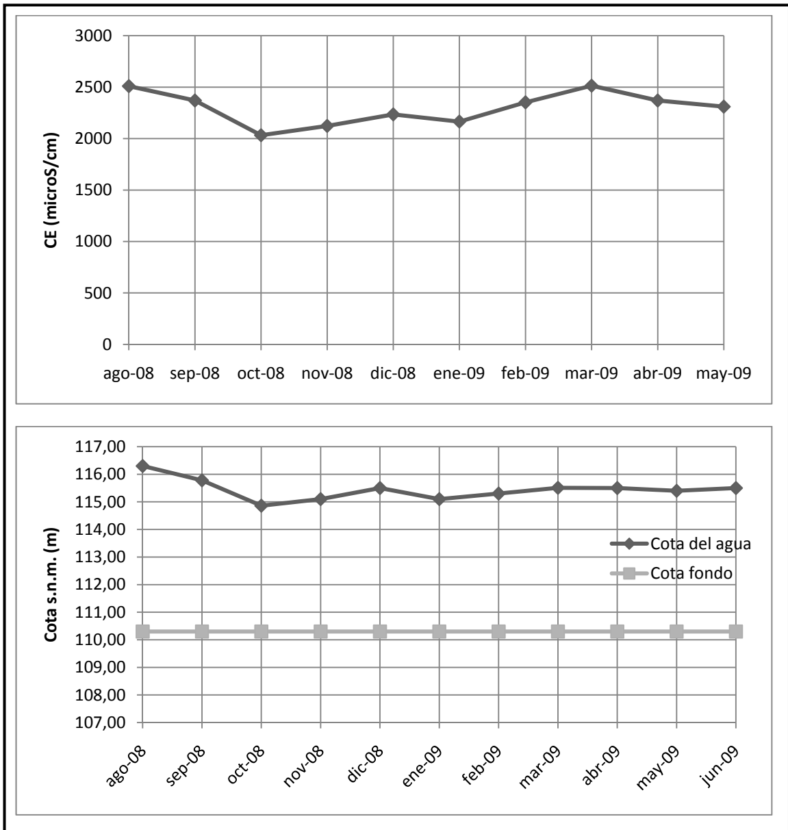
Figura A2.13. Evolución temporal del nivel piezométrico, profundidad, y conductividad eléctrica en el pozo Sayá 13.
