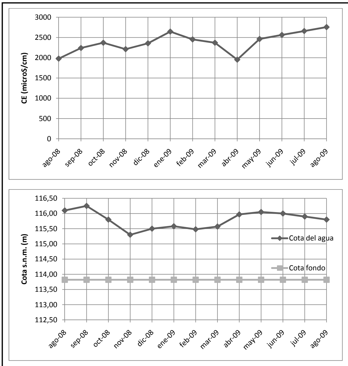
Figura A2.10. Evolución temporal del nivel piezométrico, profundidad, y conductividad eléctrica en el pozo Sayá 10.
