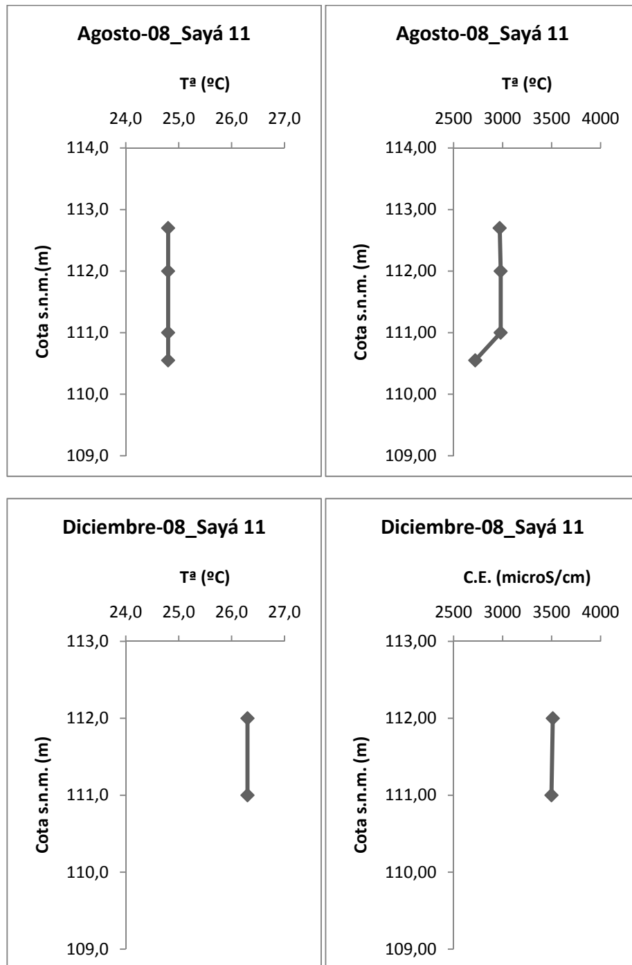
Figura A3.20. Perfiles de temperatura y conductividad eléctrica en el interior de los sondeos pozó Sayá 11.
