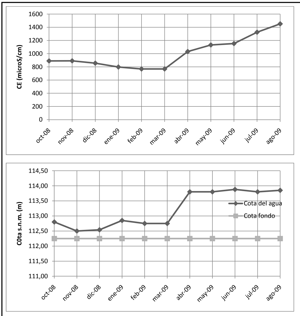
Figura A2.3. Evolución temporal del nivel piezométrico, profundidad, y conductividad eléctrica en el pozo Sayá 3.
