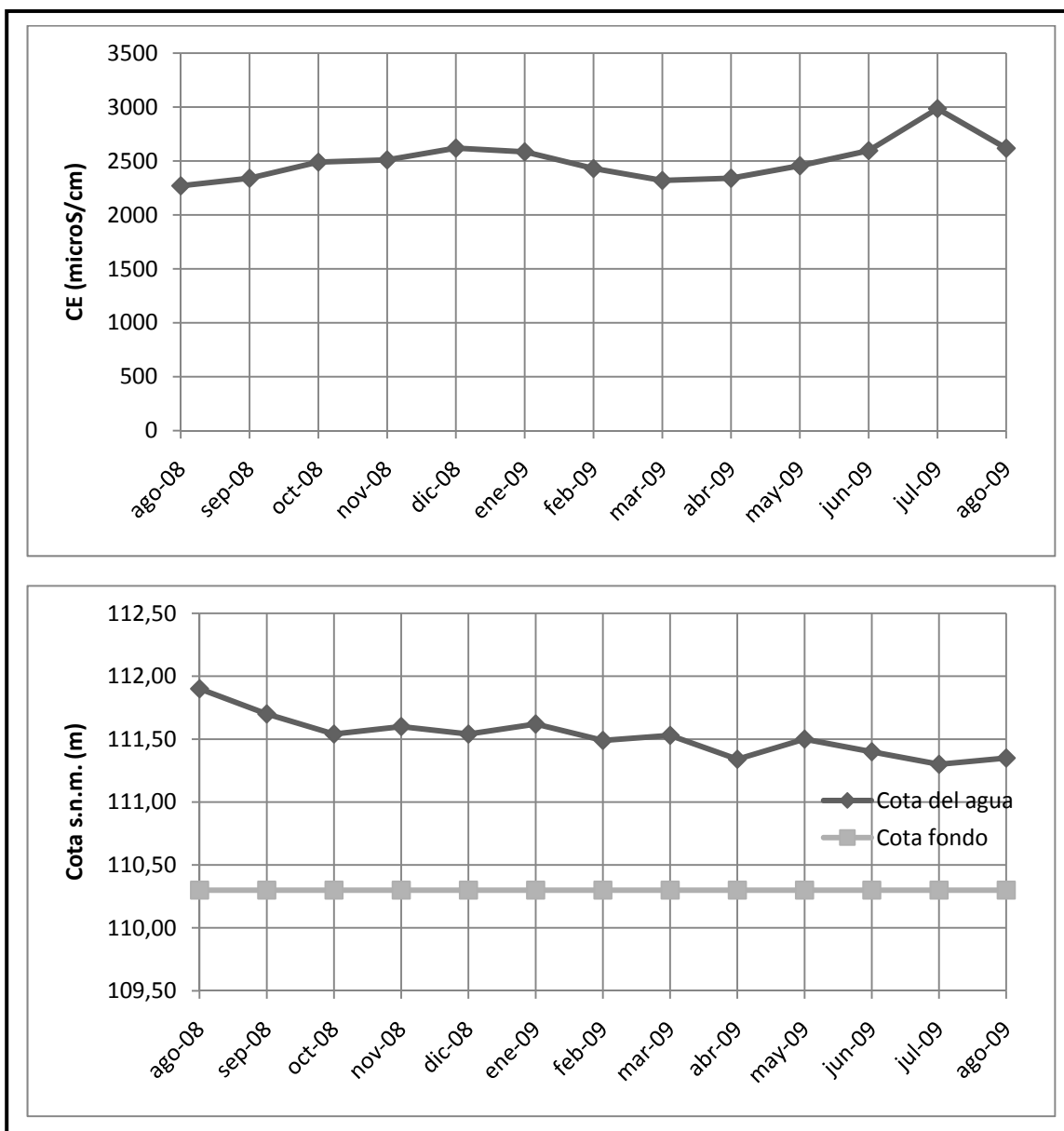
Figura A2.2. Evolución temporal del nivel piezométrico, profundidad, y conductividad eléctrica en el pozo Sayá 2.
