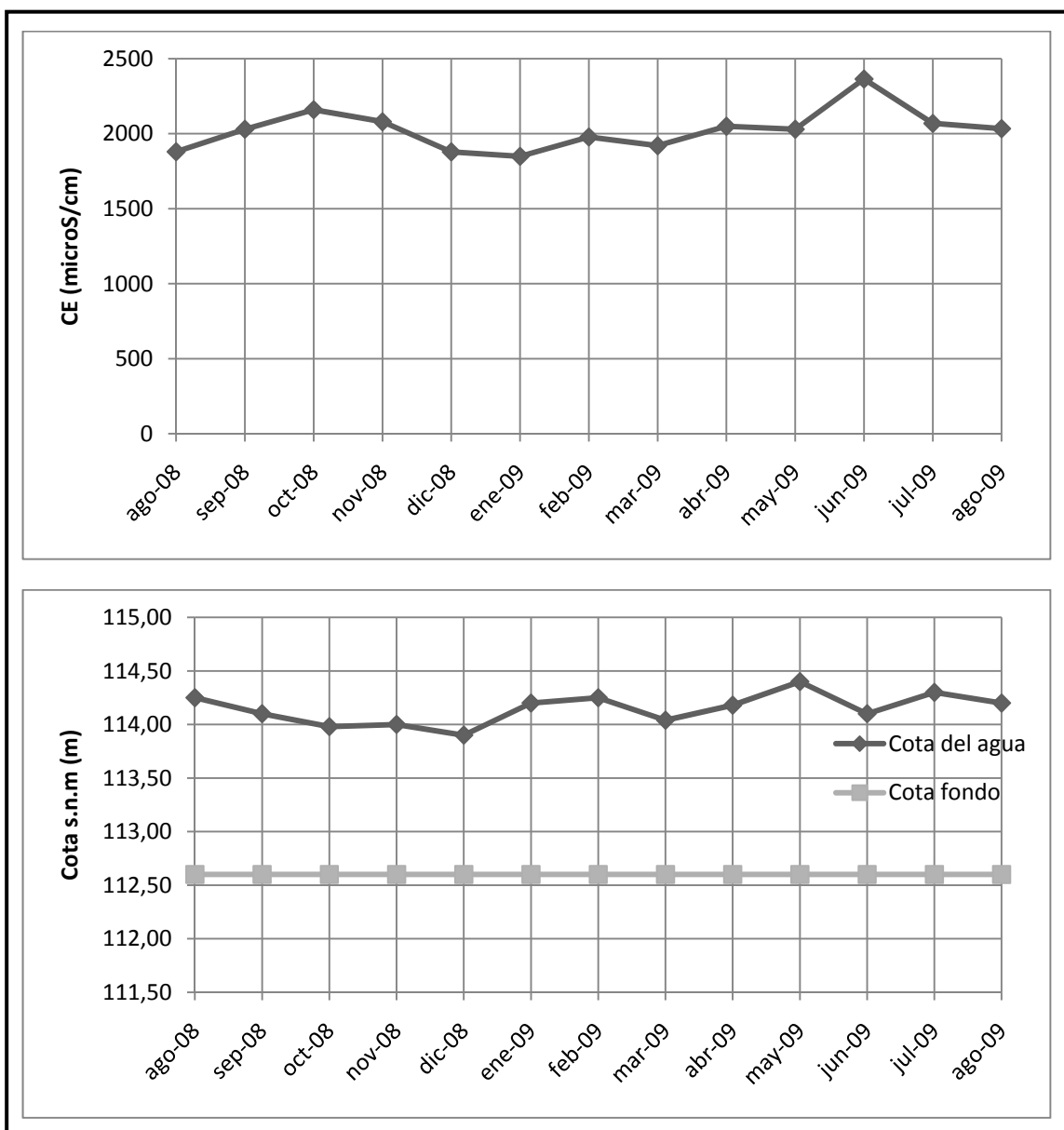
Figura A2.8. Evolución temporal del nivel piezométrico, profundidad, y conductividad eléctrica en el pozo Sayá 8.
