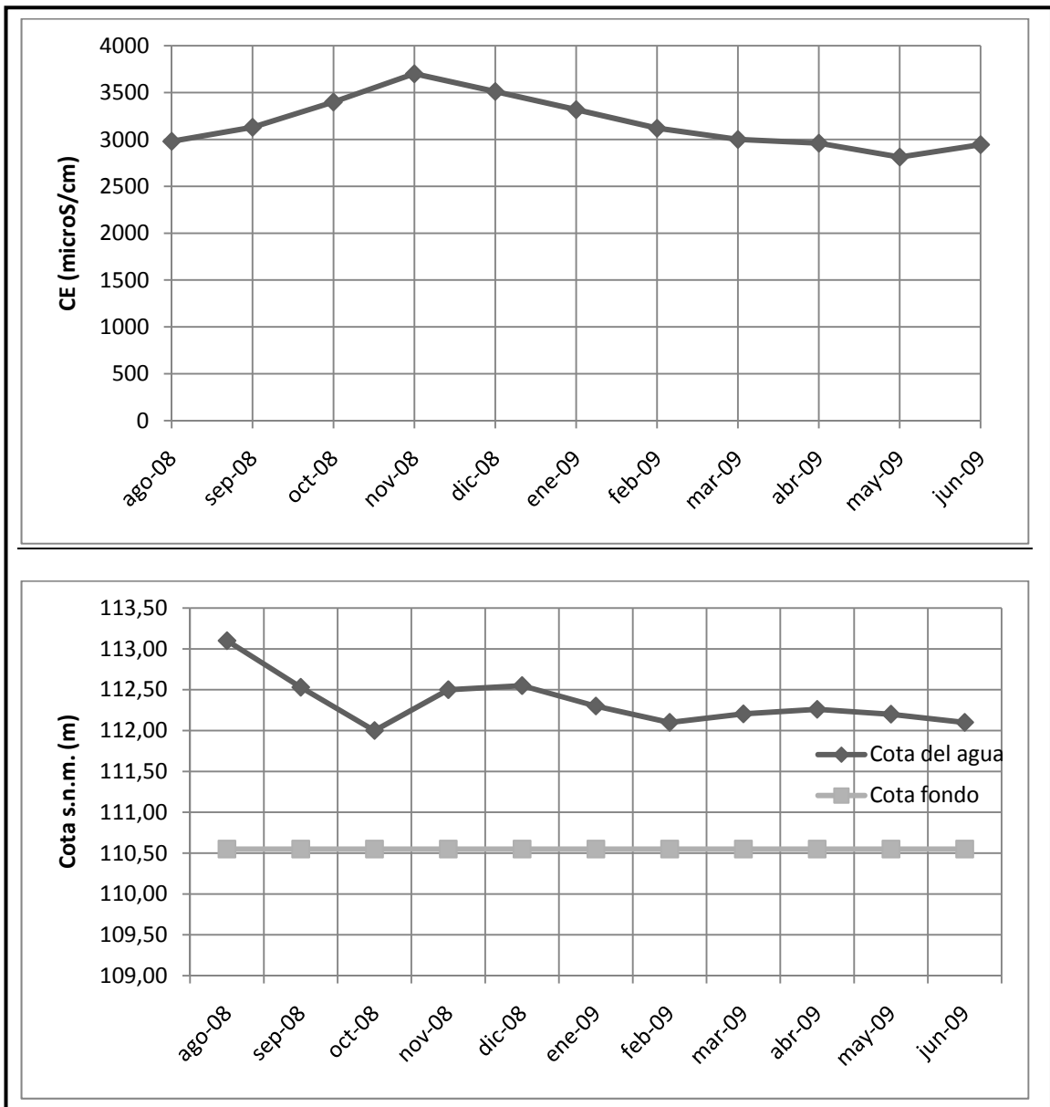
Figura A2.11. Evolución temporal del nivel piezométrico, profundidad, y conductividad eléctrica en el pozo Sayá 11.
