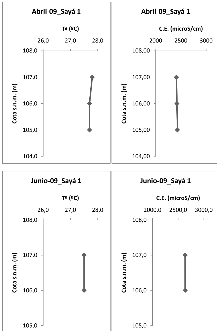
Figura A3.3. Perfiles de temperatura y conductividad eléctrica en el interior de los sondeos pozó Sayá 1.
