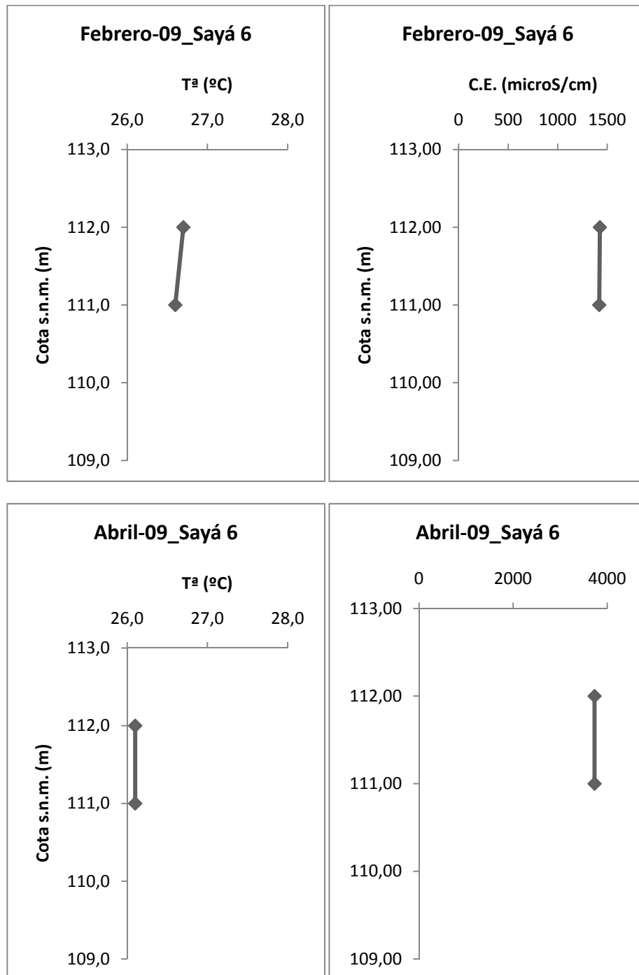
Figura A3.11. Perfiles de temperatura y conductividad eléctrica en el interior de los sondeos pozó Sayá 6.
