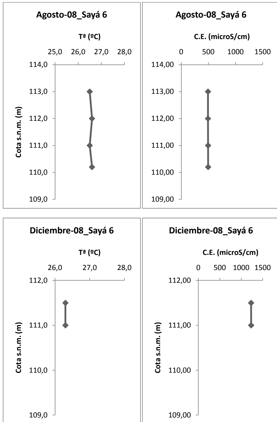
Figura A3.10. Perfiles de temperatura y conductividad eléctrica en el interior de los sondeos pozó Sayá 6.
