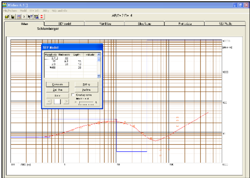
Figura A4.4. Interpretación de SEV Sayá-04, utilizando WINSEV 6.1.
