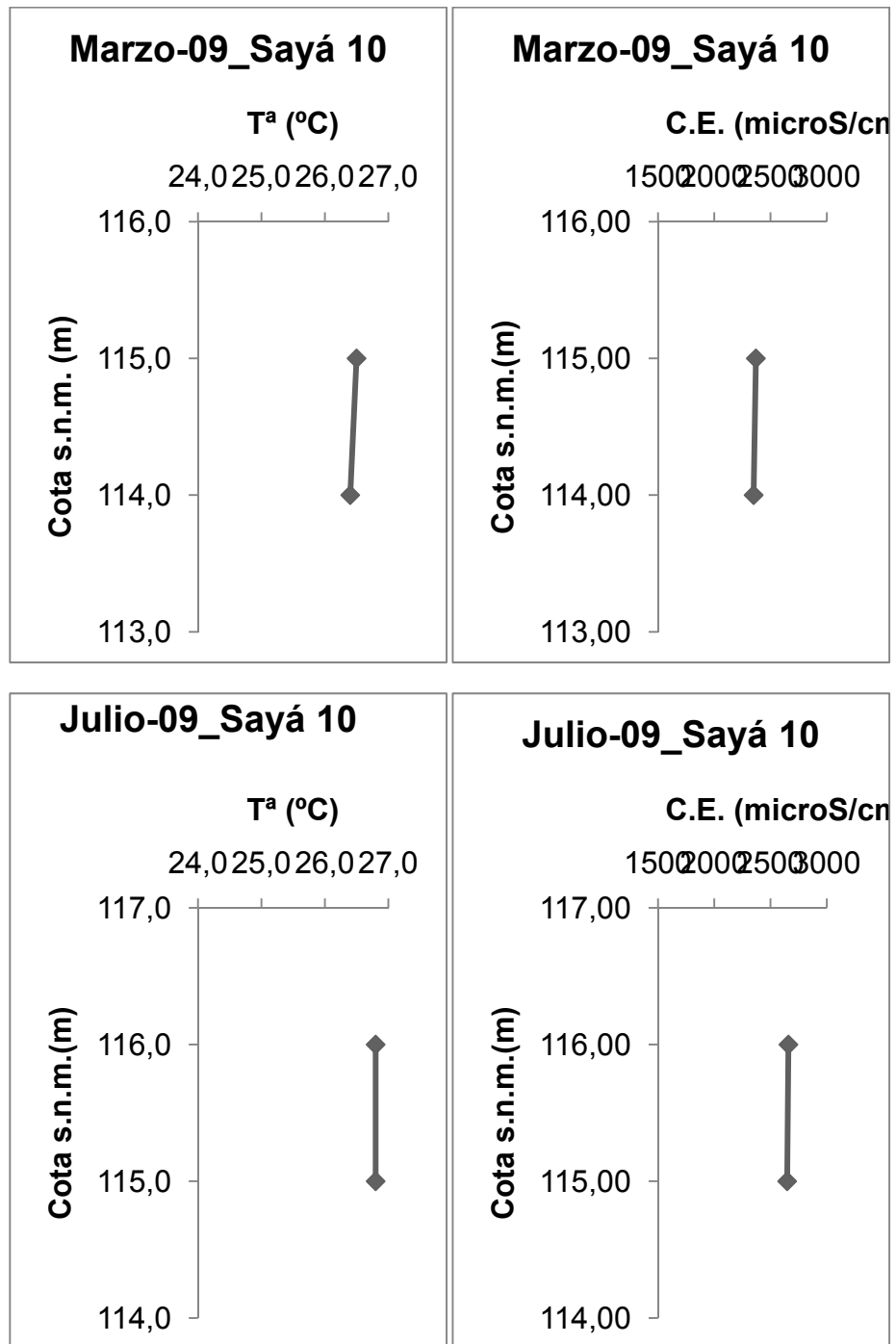
Figura A3.19. Perfiles de temperatura y conductividad eléctrica en el interior de los sondeos pozó Sayá 10.
