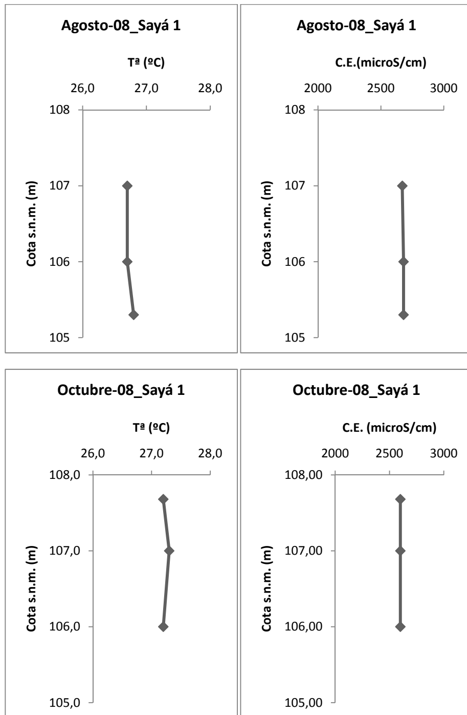
Figura A3. 1. Perfiles de temperatura y conductividad eléctrica en el interior de los sondeos pozo Sayá 1.
