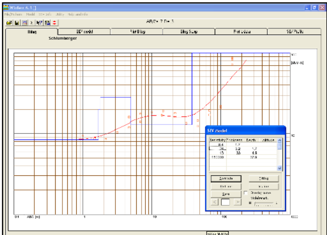
Figura A4.3. Interpretación de SEV Sayá-03, utilizando WINSEV 6.1.
