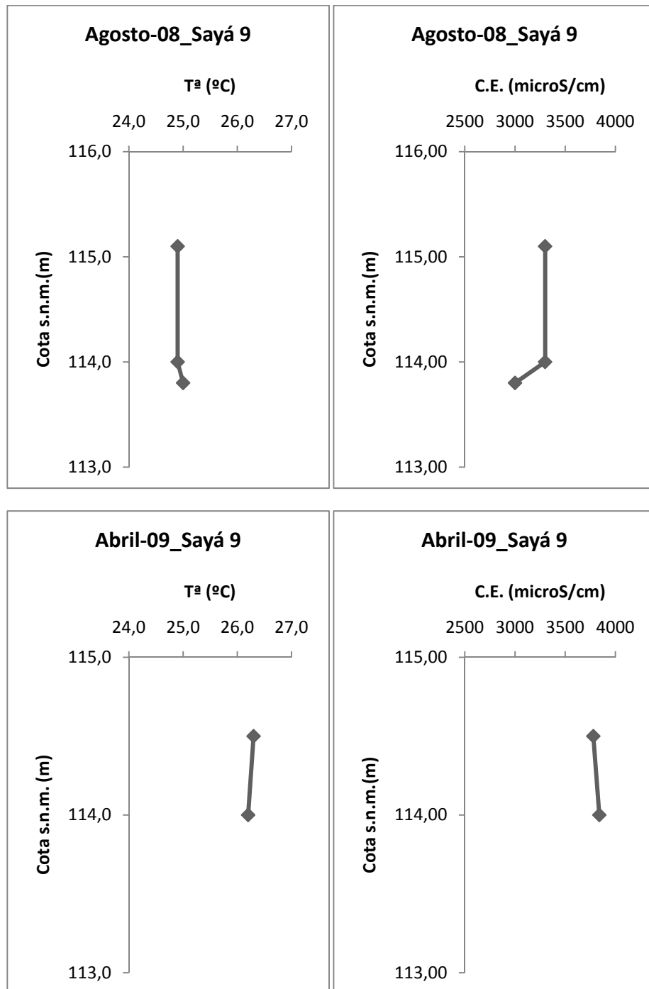
Figura A3.17. Perfiles de temperatura y conductividad eléctrica en el interior de los sondeos pozó Sayá 9.
