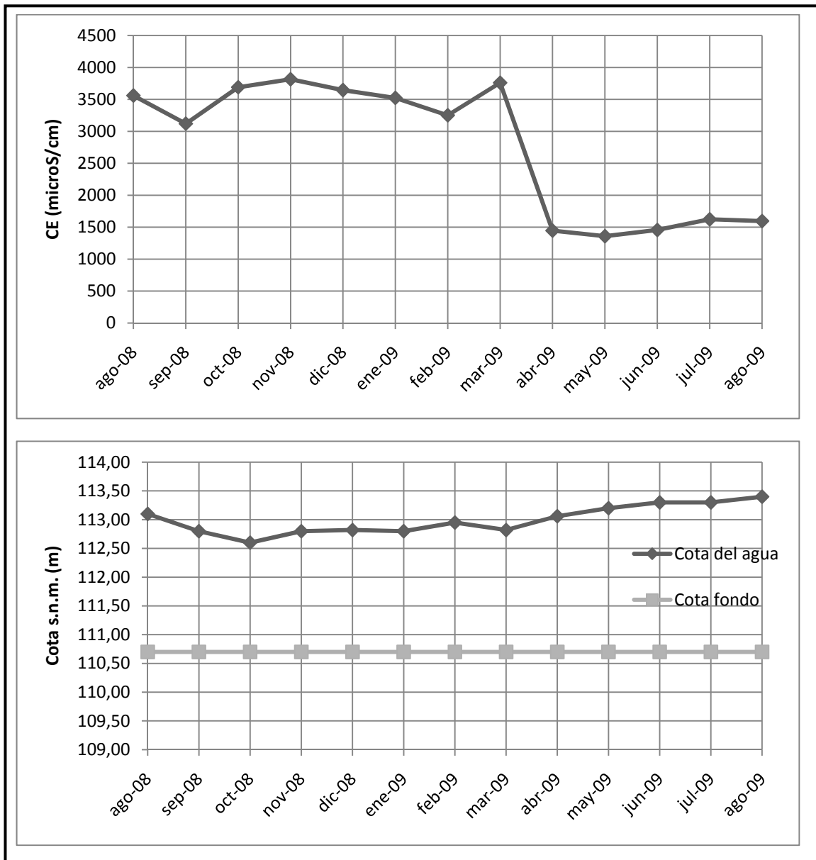
Figura A2.5. Evolución temporal del nivel piezométrico, profundidad, y conductividad eléctrica en el pozo Sayá 5.
