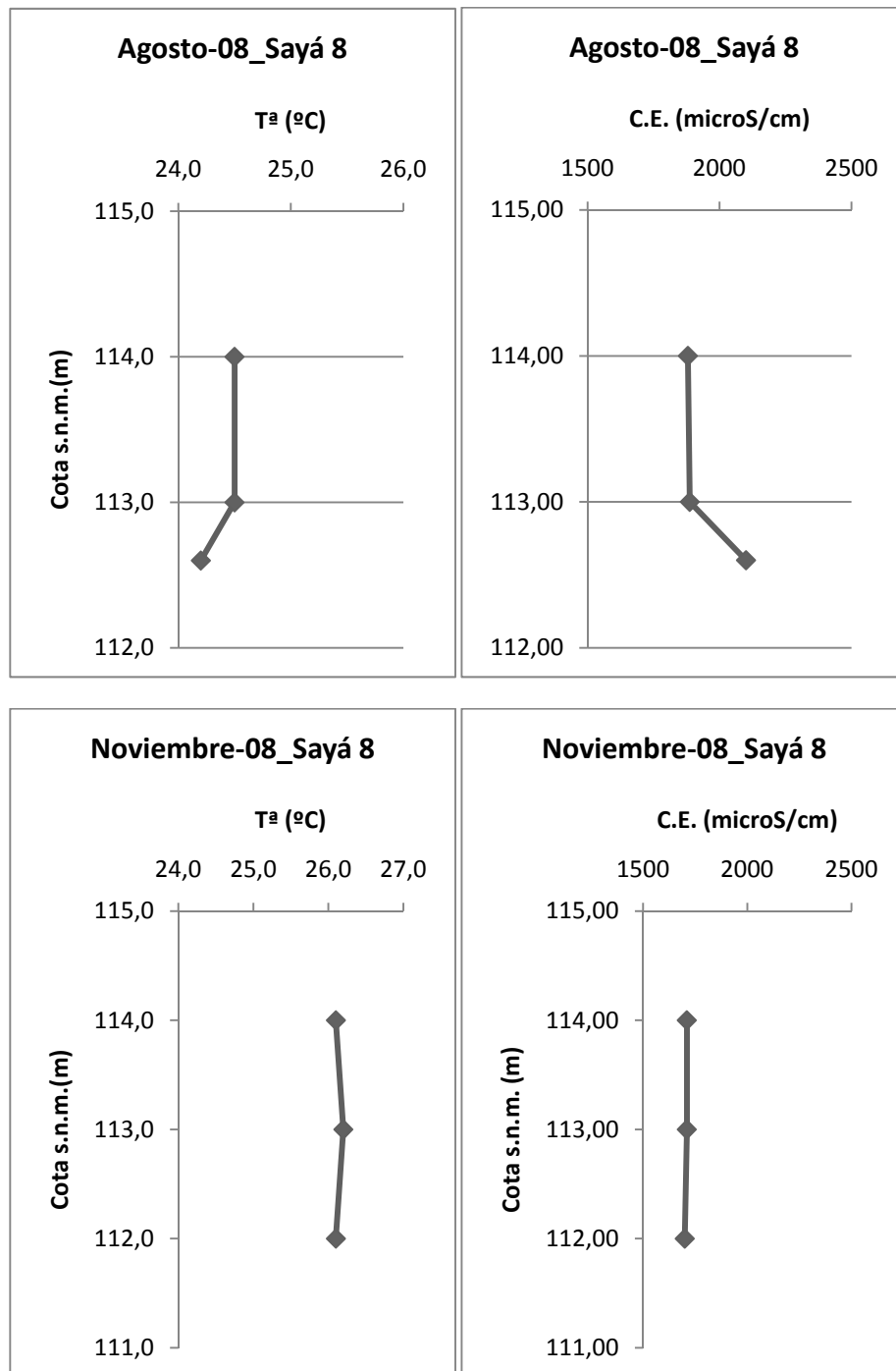
Figura A3.15. Perfiles de temperatura y conductividad eléctrica en el interior de los sondeos pozó Sayá 8.
