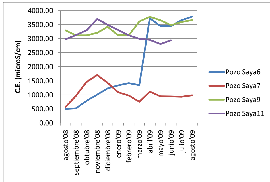
Figura 4.4.b. Evolución temporal de la conductividad eléctrica de los pozos de Sayá
