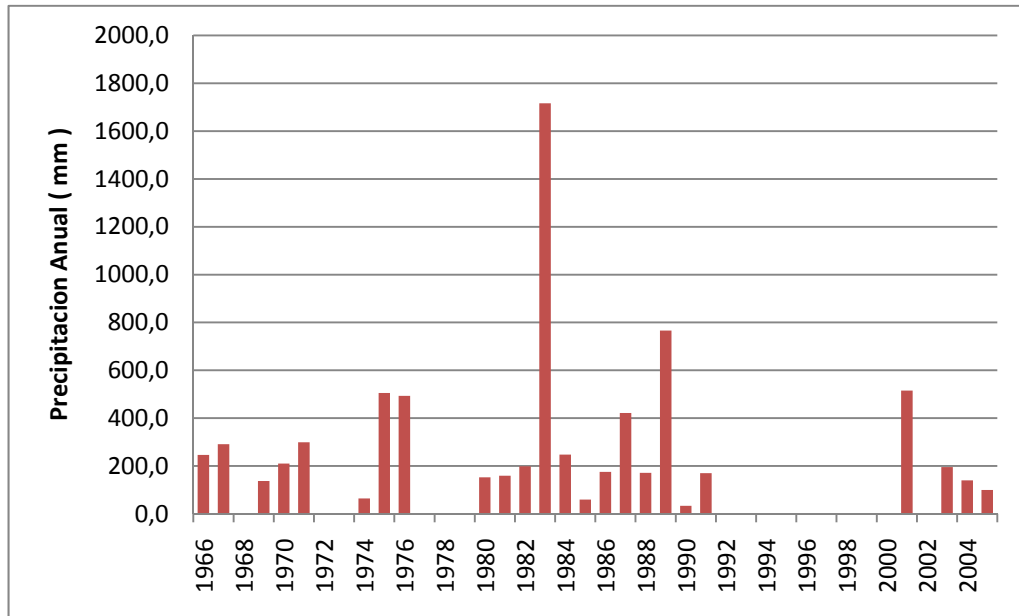
Figura. 3.3. Precipitaciones Anuales en el Área de la estación La Azúcar.
