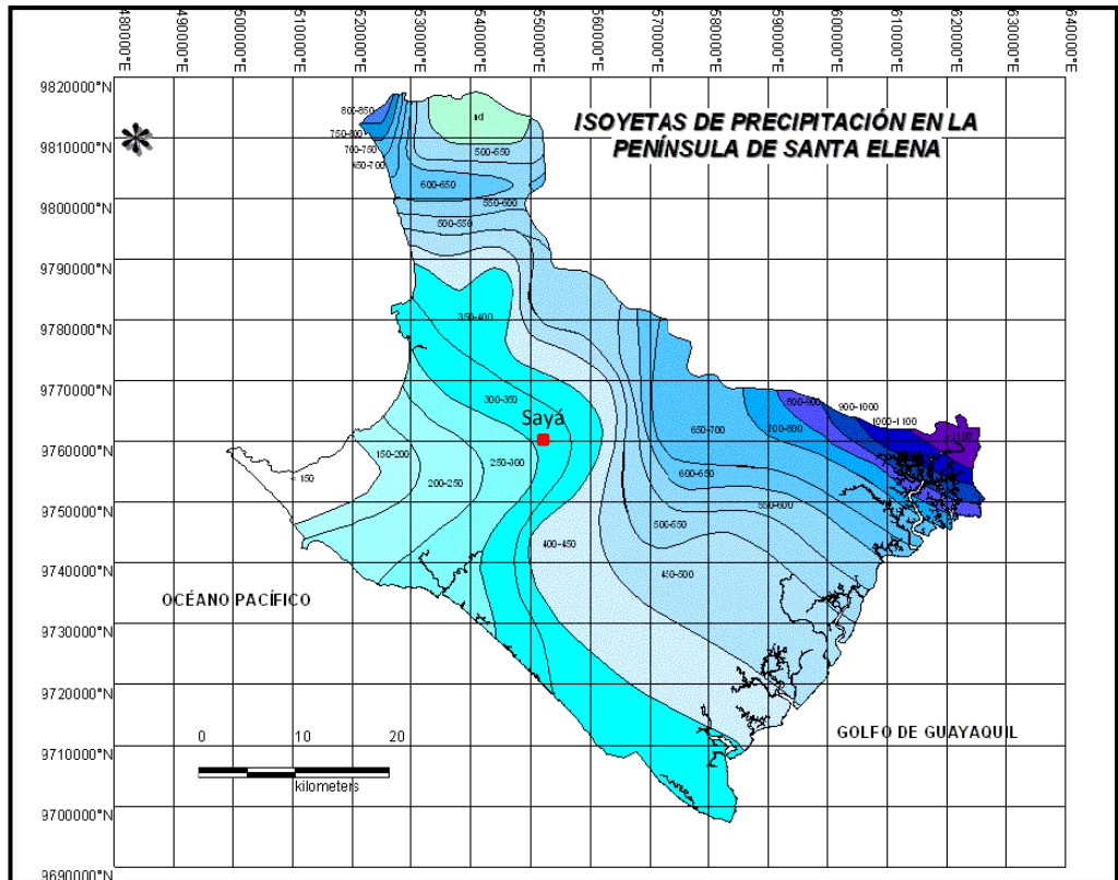
Figura 1.4 Mapa de ISO yetas de la Península de Santa Elena.
