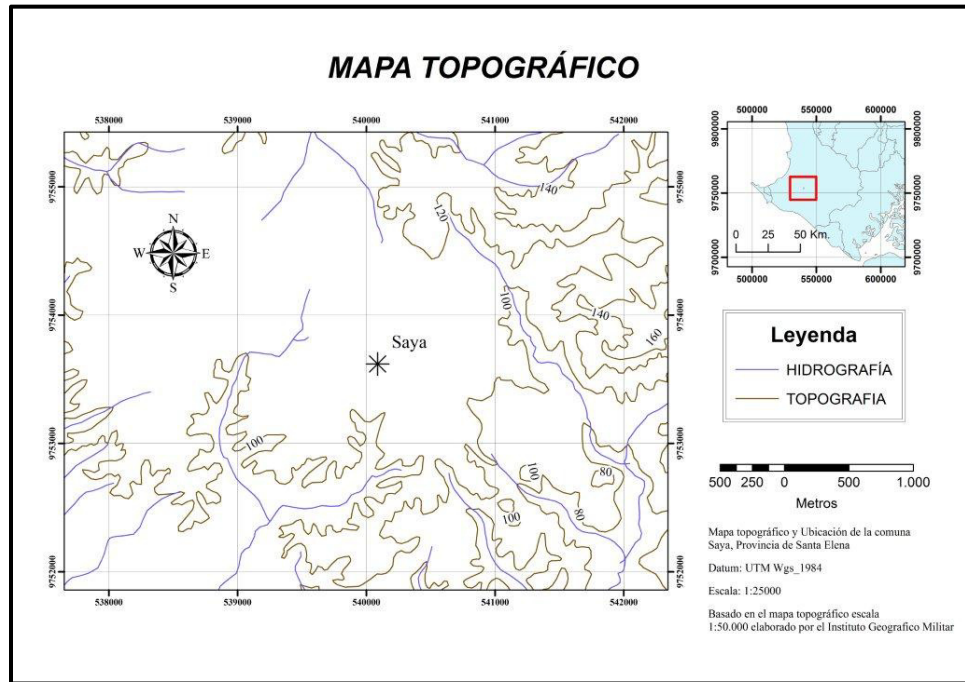
Figura 1.2. Mapa Topográfico de la zona de estudio. (ESPOL-OIEA, 2006, ECU/8/026)
