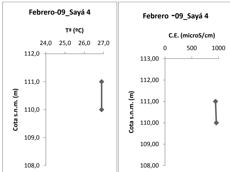
Figura A3.7. Perfiles de temperatura y conductividad eléctrica en el interior de los sondeos pozó Sayá 4.
