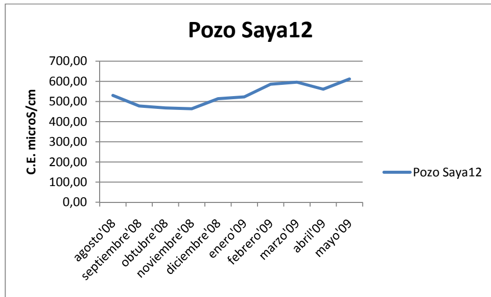
Figura 4.4.d Evolución temporal de la conductividad eléctrica de los pozos de sayá
