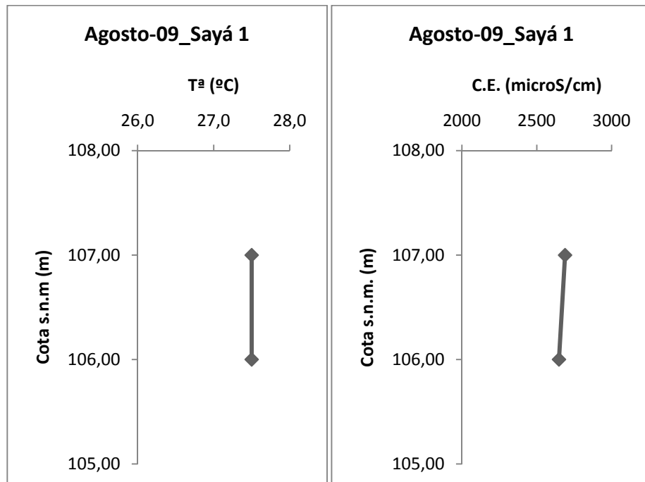
Figura A3.4. Perfiles de temperatura y conductividad eléctrica en el interior de los sondeos pozó Sayá 1.
