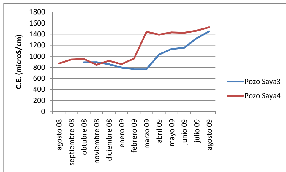
Figura 4.4.c Evolución temporal de la conductividad eléctrica de los pozos de Sayá
