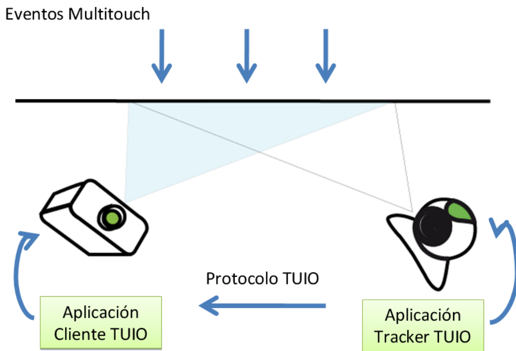
Figura 16. Esquema de Funcionamiento de la Pantalla Multitouch
