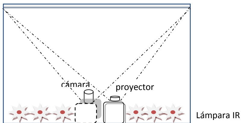
Figura 23. Esquema de una mesa Rear DI
