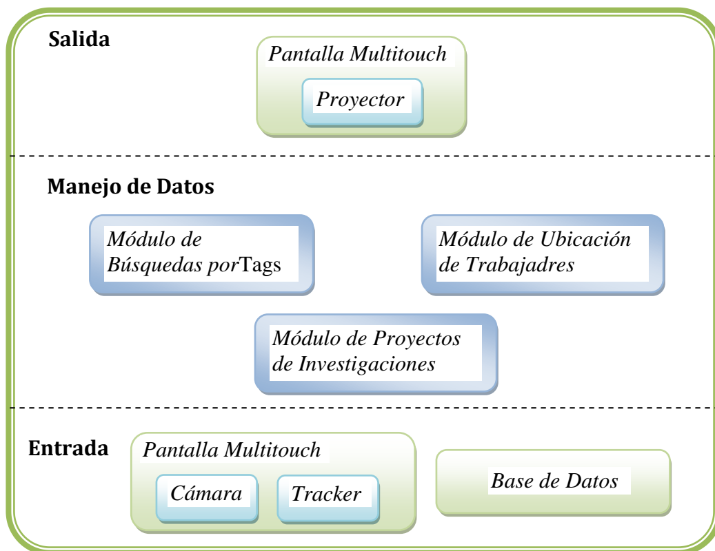
Figura 17. Arquitectura del Sistema
