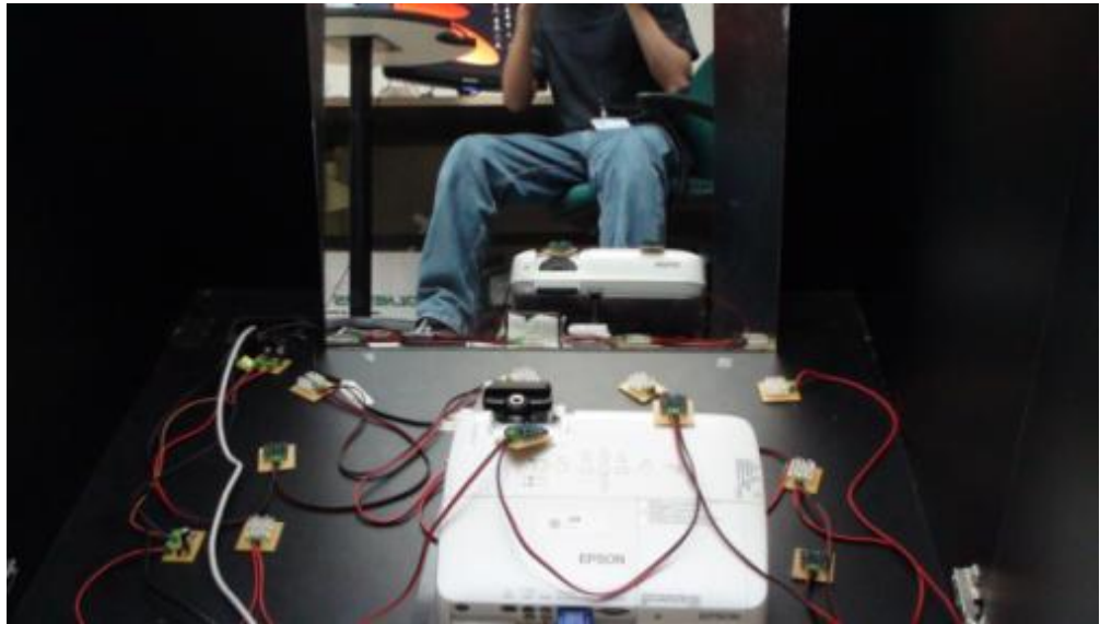
Figura 38. Vista interior de la Mesa Multitouch
