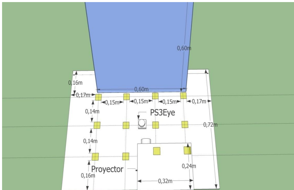
Figura 39. Medidas de los elementos internos de la mesa multitouch
