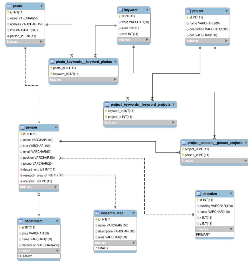
Figura 34. Diseño Estructural de la Base de Datos
