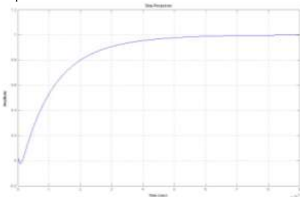
Figura 11. Respuesta de la planta en lazo cerrado con controlador.
