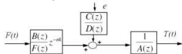
Figura 5. Diagrama de bloques modelo error predicción.
