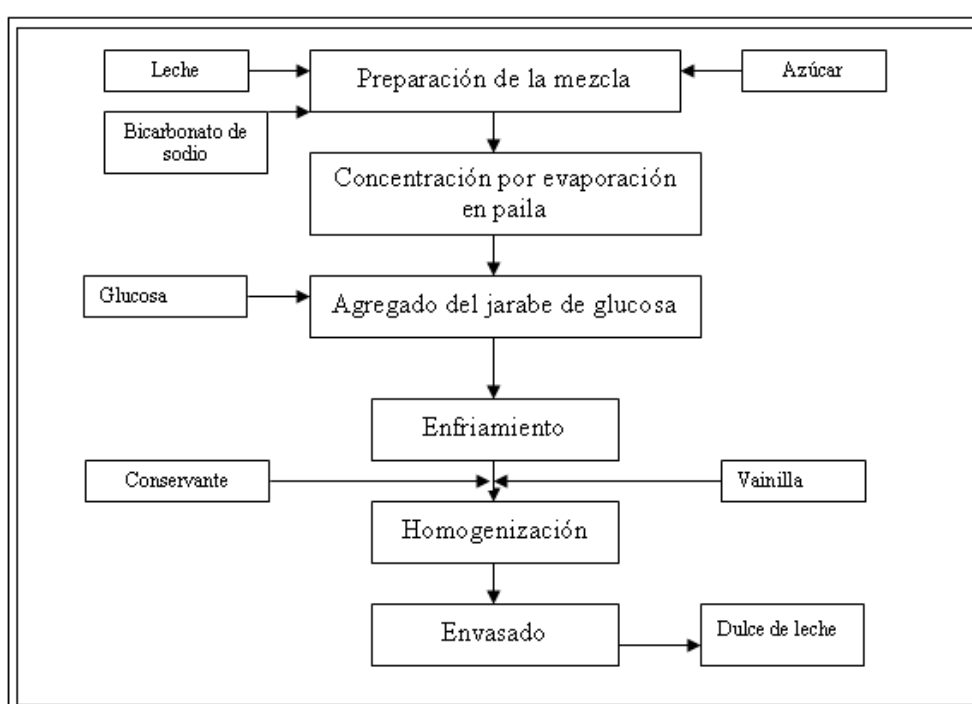
FIGURA 2.3 Diagrama de flujo del sistema en paila para la elaboración del dulce de leche.
