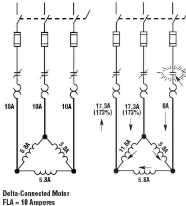
Fig. 3.8. Operación del motor bajo falla monofásica.
