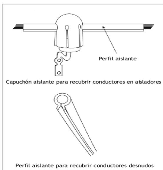
Fig. 5.13. Materiales utilizados en el método de trabajo en contacto. (Fuente: Guía Técnica para la Evaluación y Prevención de Riesgo Eléctrico)
