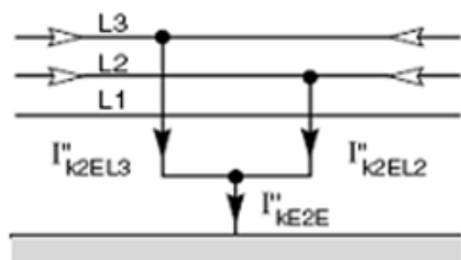
Fig. 2.2b. Cortocircuito bifásico a tierra. (Fuente: Schneider Electric – Cuaderno Técnico n 158)
