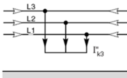
Fig. 2.1. Cortocircuito Trifásico. (Fuente: Schneider Electric – Cuaderno Técnico n 158)
