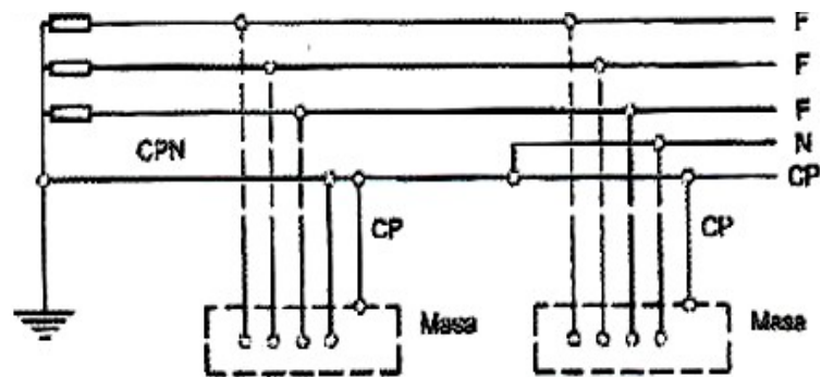
Fig. 2.9. Esquema TN-C-S. (Fuente: http://www.coitiab.es/reglamentos/electricidad/reglamentos/itc_bt/itc-bt-08.htm )
