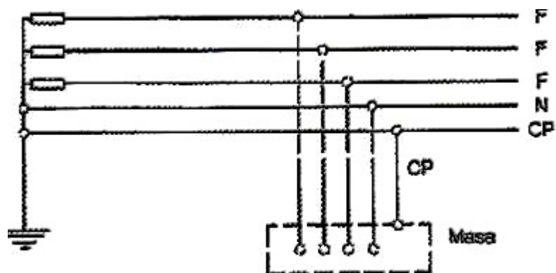
Fig. 2.7. Esquema TN-S. (Fuente: http://www.coitiab.es/reglamentos/electricidad/reglamentos/itc_bt/itc-bt-08.htm )
