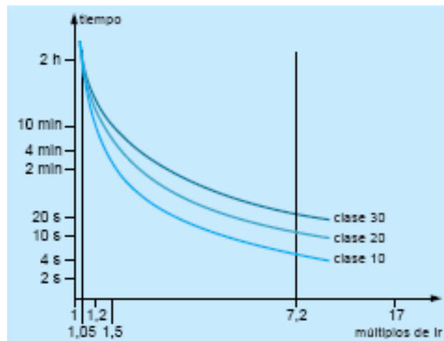
Fig. 3.11. Curvas de las clases de Relé térmico.
