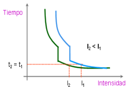
Fig. 3.6. Selectividad Amperimétrica. (Fuente: http://www.tuveras.com/aparamenta/magnetotermico.htm )
