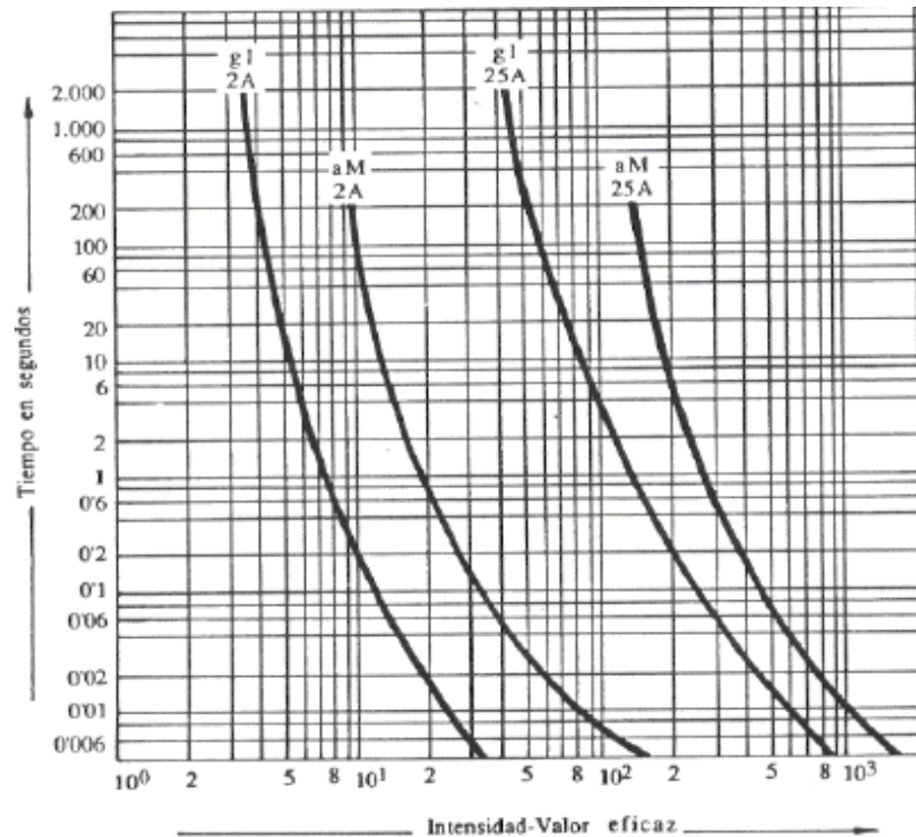
Fig. 3.2. Curvas características de fusibles. Fuente: Escuela Universitaria de Ingeniería Técnica Agrícola de Ciudad Real
