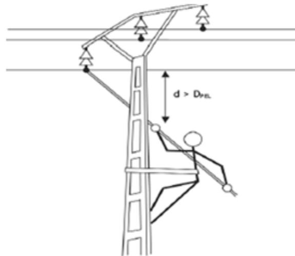
Fig. 5.12. Método de trabajo a distancia. (Fuente: Guía Técnica para la Evaluación y Prevención de Riesgo Eléctrico)
