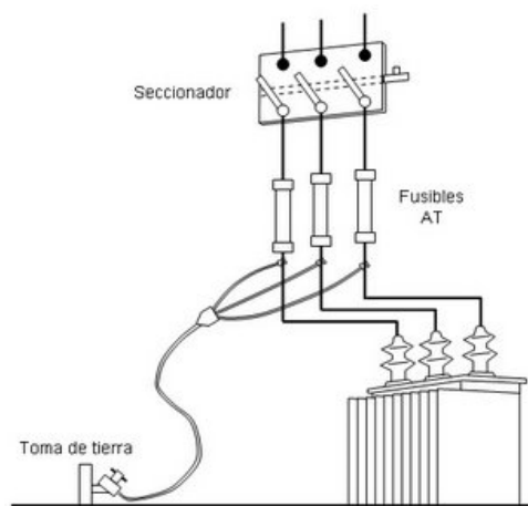
Fig. 5.9. Puesta a tierra de un circuito de alta tensión. (Fuente: Guía Técnica para la Evaluación y Prevención de Riesgo Eléctrico)
