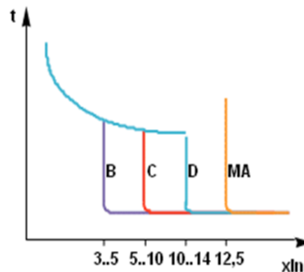
Fig. 3.5. Curvas características de disparo para las diversas clases de disyuntores magnetotérmicos. (Fuente: http://www.tuveras.com/aparamenta/magnetotermico.htm )
