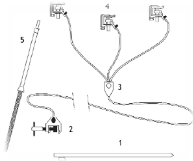
Fig. 5.7. Elementos de un equipo portátil de puesta a tierra. (Fuente: Guía Técnica para la Evaluación y Prevención de Riesgo Eléctrico)
