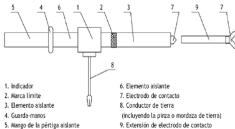
Fig. 5.5b. Detector de tensión tipo resistivo para AT. (Fuente: Guía Técnica para la Evaluación y Prevención de Riesgo Eléctrico)
