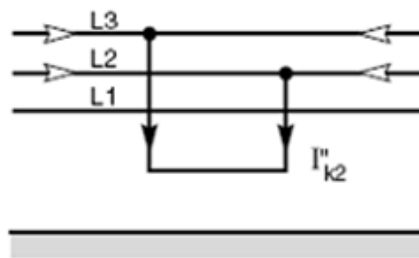
Fig. 2.2a. Cortocircuito bifásico aislado. (Fuente: Schneider Electric – Cuaderno Técnico n 158)
