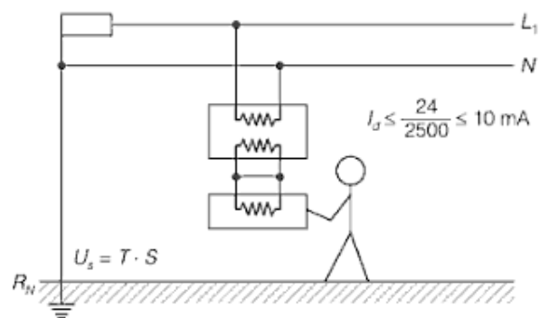
Fig. 4.5. Empleos de pequeñas tensiones de Seguridad (Fuente: http://www.sprl.upv.es/IOP_ELEC_05.htm )
