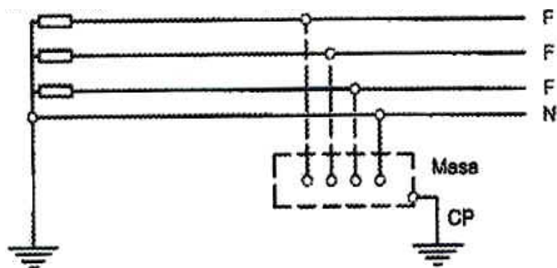
Fig. 2.10. Esquema TT. (Fuente: http://www.coitiab.es/reglamentos/electricidad/reglamentos/itc_bt/itc-bt-08.htm )
