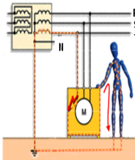
Fig. 2.6. Contacto eléctrico frente a una falla de aislamiento.
