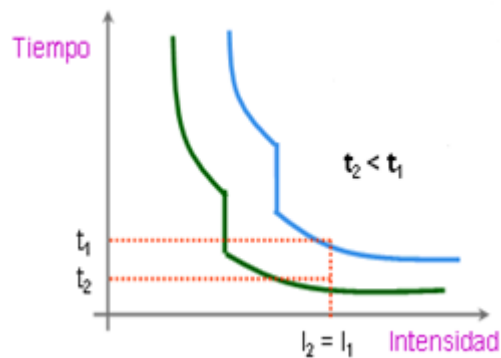
Fig. 3.7. Selectividad Cronométrica. (Fuente: http://www.tuveras.com/aparamenta/magnetotermico.htm )
