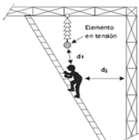
Fig. 5.11. Método de trabajo a potencial. (Fuente: Guía Técnica para la Evaluación y Prevención de Riesgo Eléctrico)
