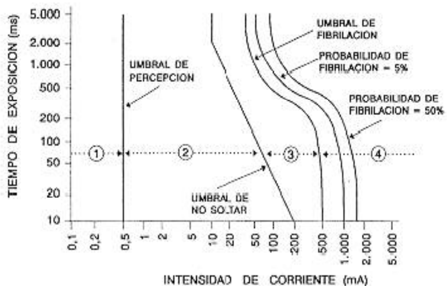
Fig. 1.3. Curvas de seguridad (I vs t) para corriente alterna (50-60Hz) trayectoria mano izquierda - pies. (Fuente: Instituto Nacional de Seguridad e Higiene en el Trabajo)
