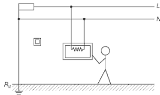
Fig. 4.6. Separación de las partes activas. (Fuente: http://www.spri.upv.es/IOP_ELEC_05.htm )
