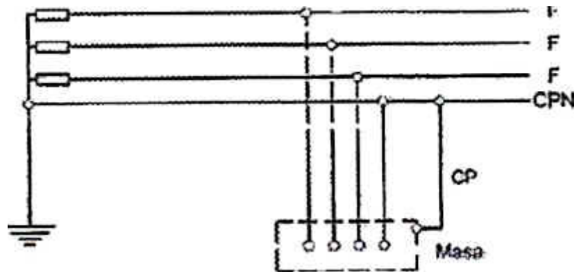
Fig. 2.8. Esquema TN-C. (Fuente: http://www.coitiab.es/reglamentos/electricidad/reglamentos/itc_bt/itc-bt-08.htm )
