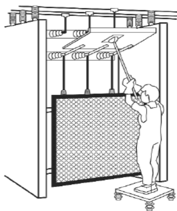
Fig. 5.4. Colocación de láminas aislantes. (Fuente: Guía Técnica para la Evaluación y Prevención de Riesgo Eléctrico)
