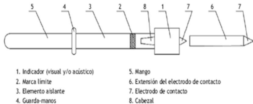
Fig. 5.5a. Detector de tensión tipo capacitivo para AT. (Fuente: Guía Técnica para la Evaluación y Prevención de Riesgo Eléctrico)
