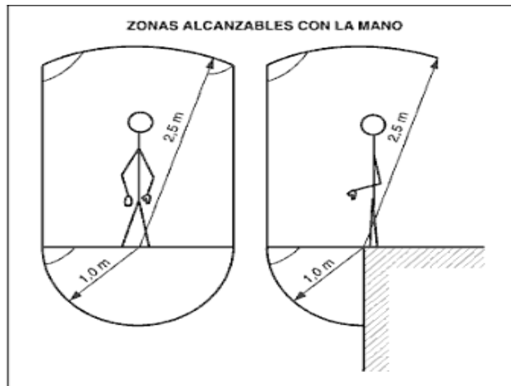
Fig. 4.3. Zonas de alejamiento de las partes activas. (Fuente: http://www.sprl.upv.es/IOP_ELEC_04.htm )
