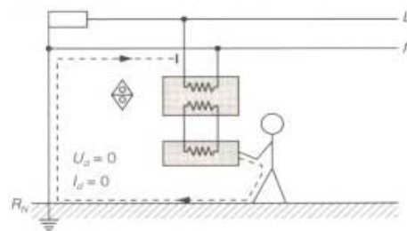
Fig. 4.4. Separación de circuitos. (Fuente: http://www.sprl.upv.es/IOP_ELEC_05.htm )
