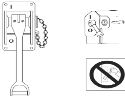
Fig. 5.2. Inmovilización del aparato de maniobra. (Cortesía: Guía Técnica para la Evaluación y Prevención de Riesgo Eléctrico)
