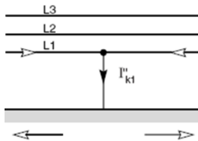
Fig. 2.3. Cortocircuito fase-tierra. (Fuente: Schneider Electric – Cuaderno Técnico n 158)
