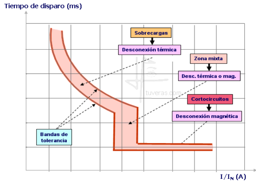
Fig. 3.4. Curva de disparo.
