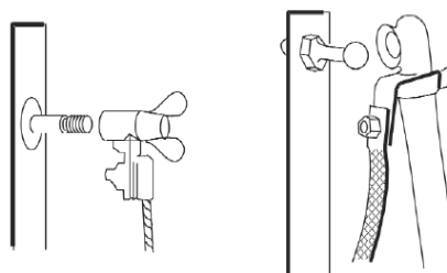
Fig. 5.8. Puntos fijos de puesta a tierra. (Fuente: Guía Técnica para la Evaluación y Prevención de Riesgo Eléctrico)
