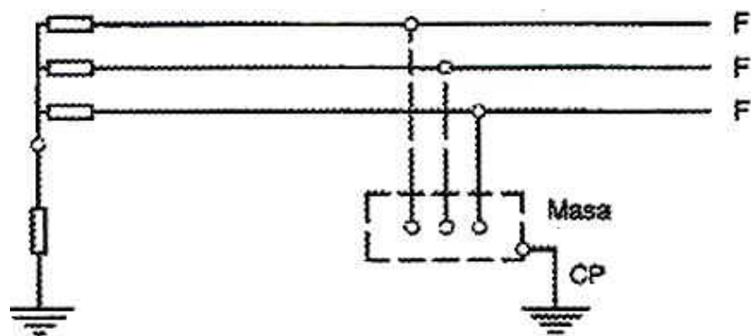
Fig. 2.11. Esquema IT. (Fuente: http://www.coitiab.es/reglamentos/electricidad/reglamentos/itc_bt/itc-bt-08.htm )
