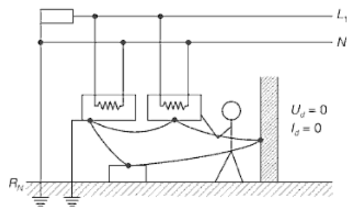
Fig. 4.7. Conexión equipotencial de las masas. (Fuente: Universidad Politécnica de Valencia)
