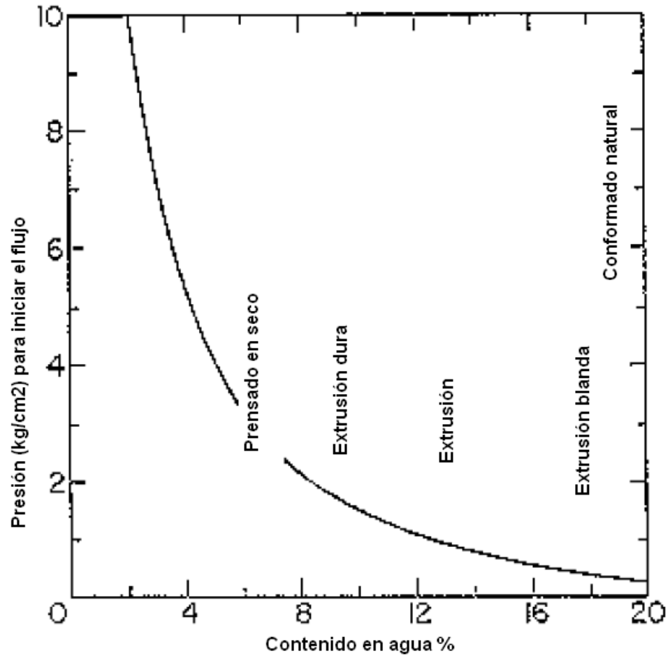
FIGURA 2.5. SISTEMAS DE MOLDEO EN BASE AL CONTENIDO DE AGUA Y PRESIÓN INICIAL
