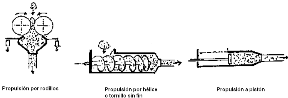
FIGURA 2.3. PRENSAS DE EXTRUSIÓN
