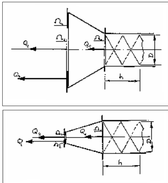
FIGURA 2.6. CONICIDAD DE BOCA
