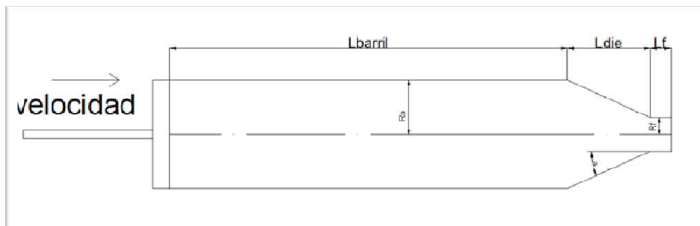
FIGURA 4.1. Vista de prototipo de extrusora
