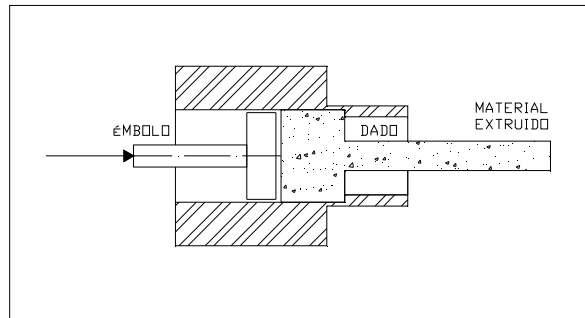
FIGURA 2.2. ESQUEMA DE EXTRUSORA
