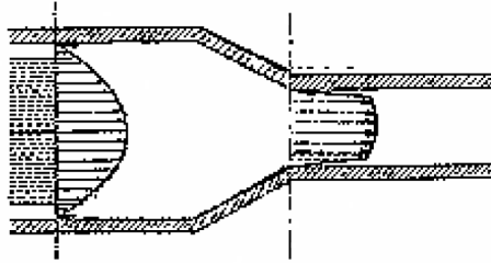
FIGURA 2.4. DISTRIBUCIÓN DE VELOCIDADES DE SALIDA
