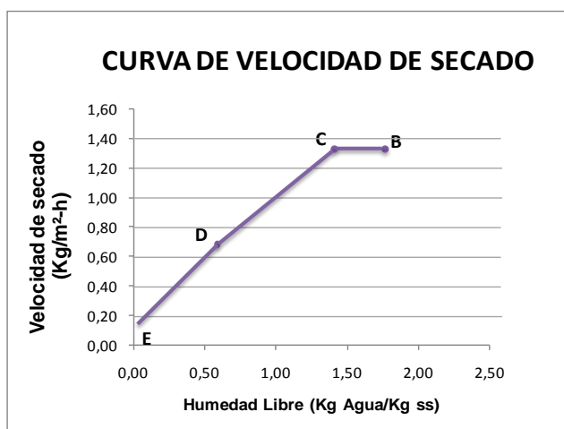
FIGURA 2.8- CURVA DE VELOCIDAD DE SECADO
