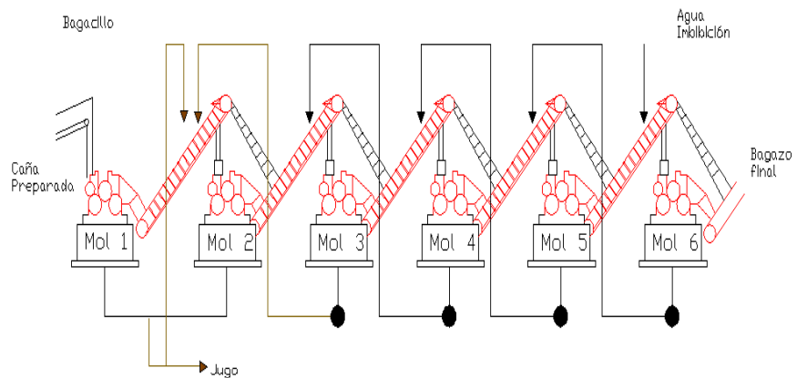
Figura 1.2 TÁNDEM DE MOLINOS
