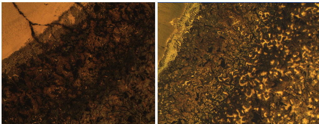
Figura 2.24 ZAT 50X producto A-1
