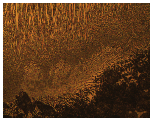
Figura 2.20 ZF 400X producto B-2
