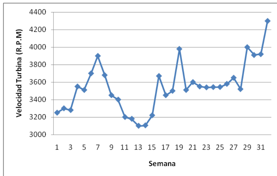
Figura 3.1 GRÁFICO VELOCIDAD TURBINAS VERSUS SEMANAS DE OPERACIÓN
