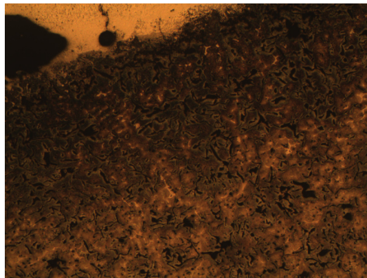
Figura 2.31 ZAT 50X producto B-2
