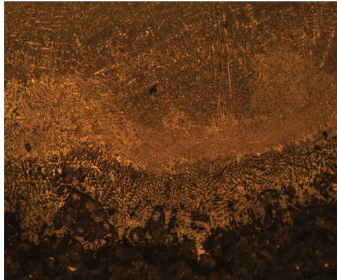
Figura 2.11 ZF 100X Producto A-1
