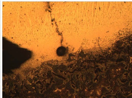
Figura 2.18 ZF 100X producto B-2
