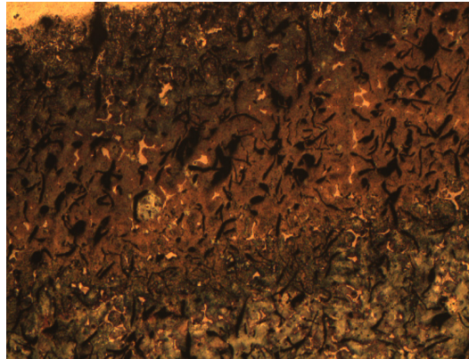
Figura 2.30 ZAT 50X producto B-1
