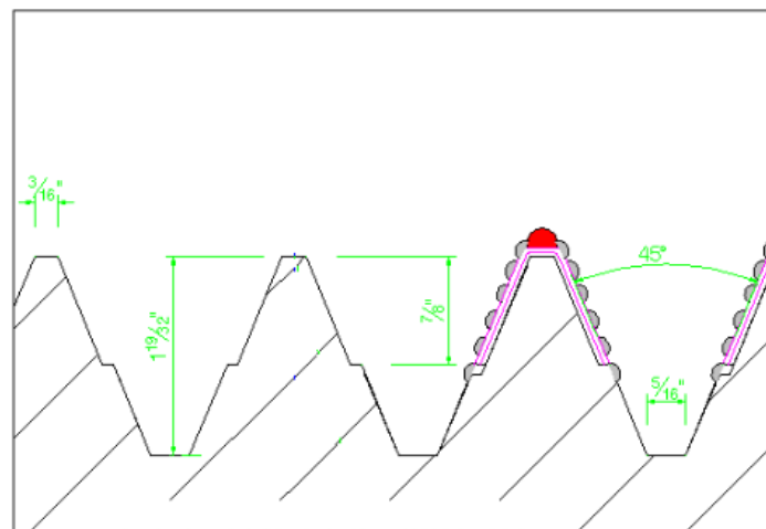
Figura 1.12 DETALLE DE APLICACIÓN RECUBRIMIENTO
