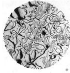
Figura 1.10 MICROESTRUCTURA DEL HIERRO GRIS (FERRITA Y PERLITA)
