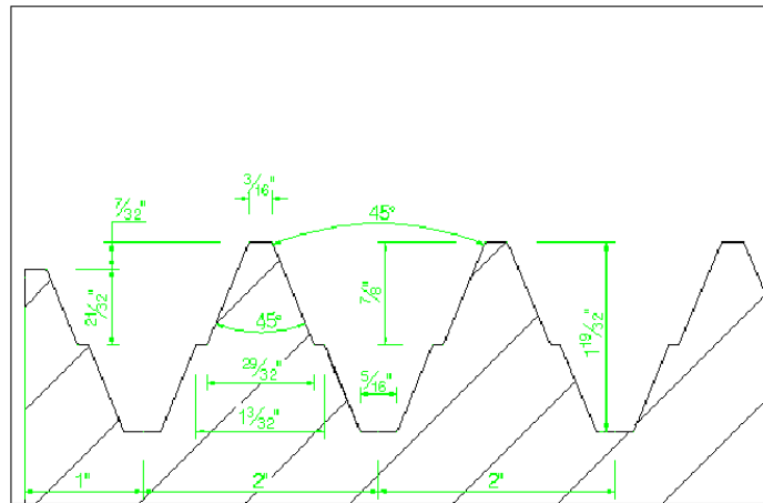
Figura 1.11 DETALLE DIENTES PREVIO A BLINDAJE
