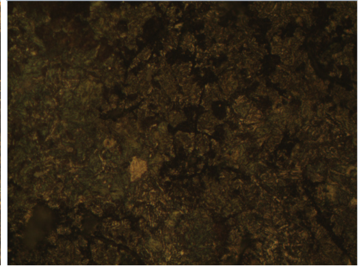
Figura 2.37 ZAT 500X producto C
