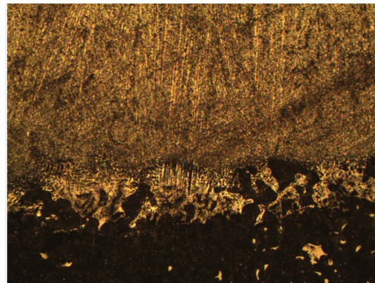
Figura 2.22 ZF 100X producto C
