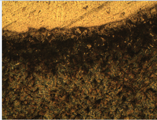
Figura 2.36 ZAT 50X producto C
