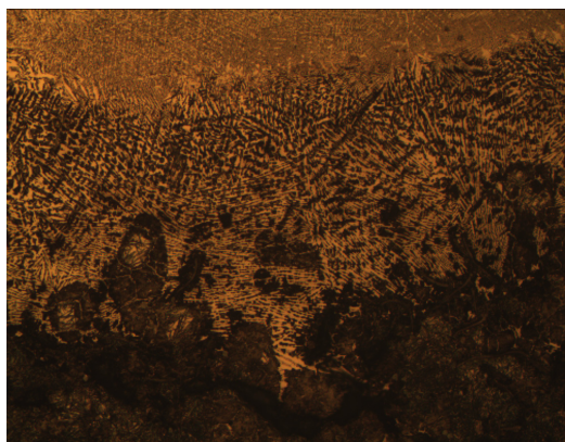
Figura 2.13 ZF 400X Producto A-1
