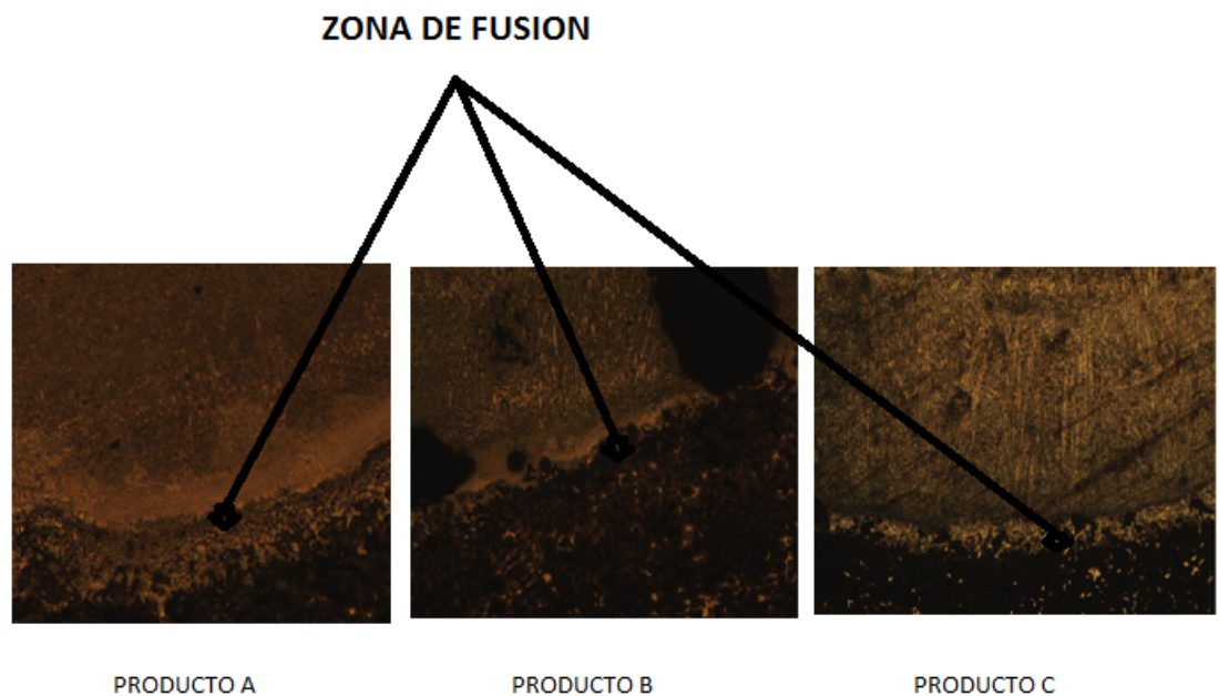
Figura 3.2 ZONA DE FUSIÓN DE LOS RECUBRIMIENTOS UTILIZADOS.
