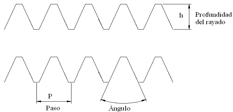
Figura 1.6 DESCRIPCIÓN DE LOS DIENTES DE LAS MAZAS
