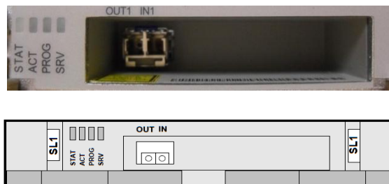
Figura 4.11 Vista frontal de la tarjeta R1SL1 [13].
