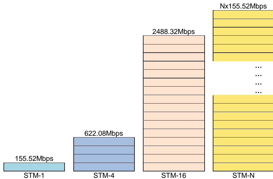
Figura 1.14 Señales en SDH.
