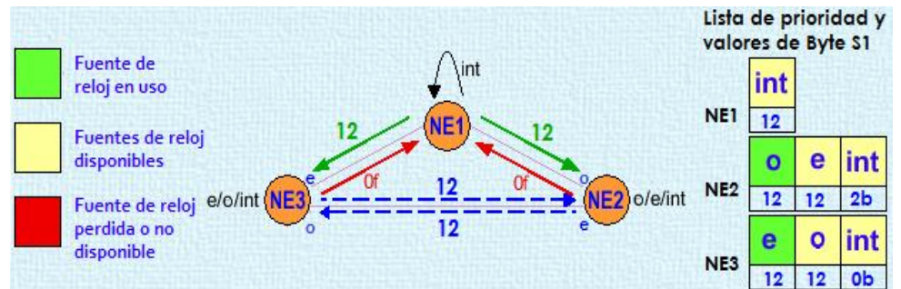
Figura 5.12 Representación de las características de sincronización a configurar.
