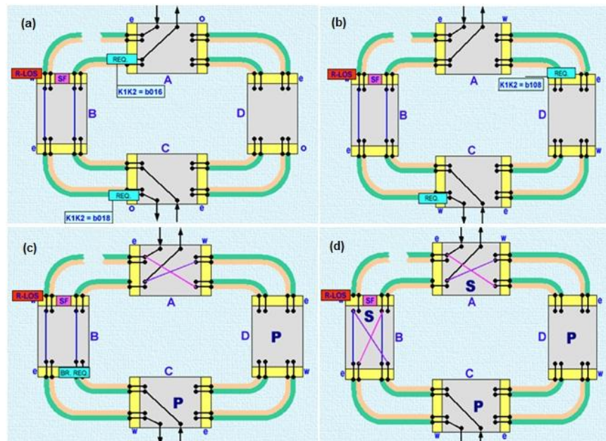
Figura 3.10 Anillo MSP unidireccional en condiciones de falla.
