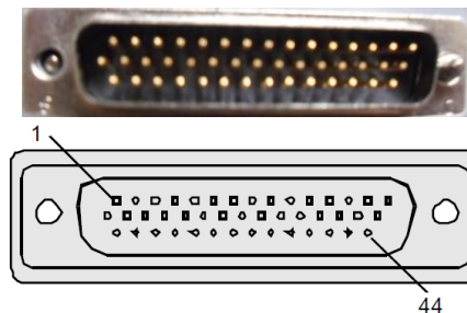
Figura 4.37 Conector hembra DB-44 [13].
