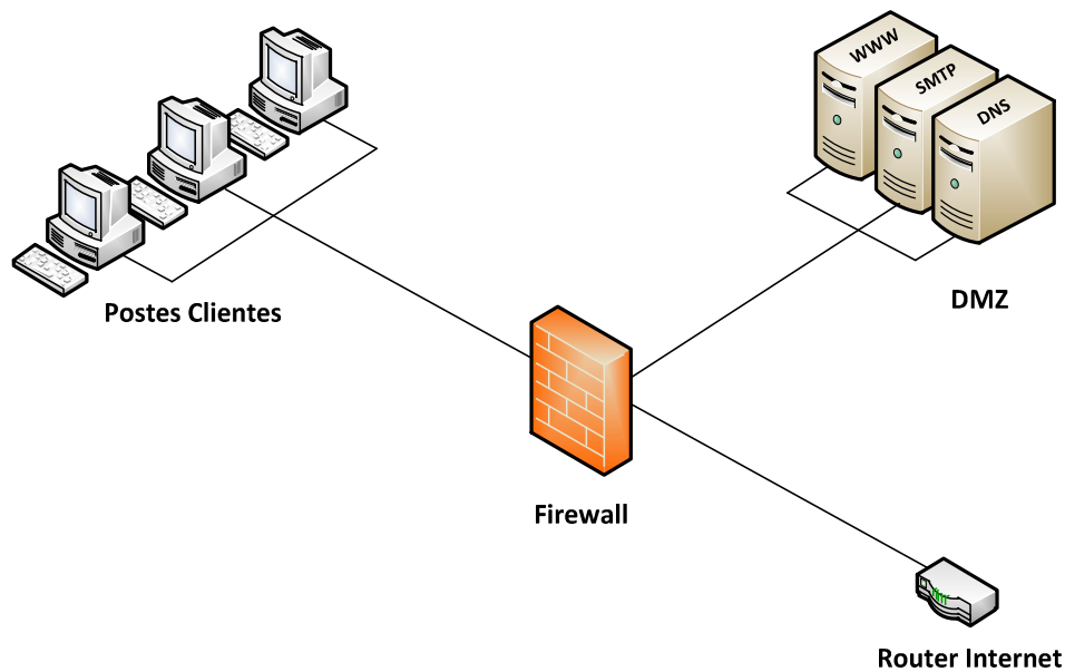
Fig. 1 1 Diagrama de una red típica que usa una DMZ con un cortafuegos de tres patas (three-legged).
