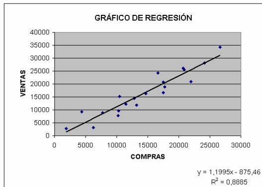
Gráfico 3: Regresión lineal
