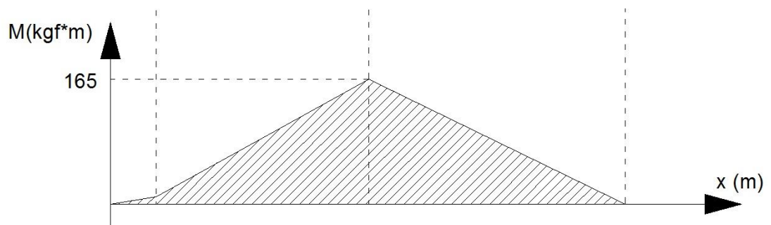
Figura 4-10 GRÁFICA DEL MOMENTO FLECTOR EN BARRA 2
