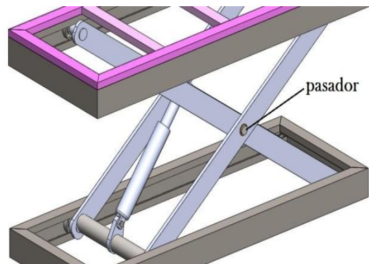
Figura 4-25 PASADOR EN TIJERAS
