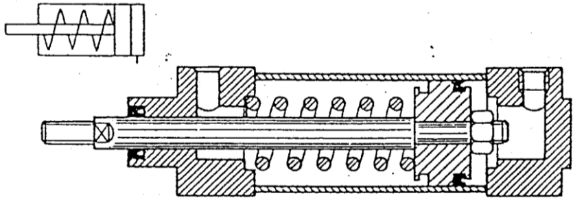
Figura 3-7 CILINDRO NEUMÁTICO DE SIMPLE ACCIÓN
