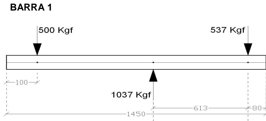
Figura 4-14 FUERZAS EN BARRA 1
