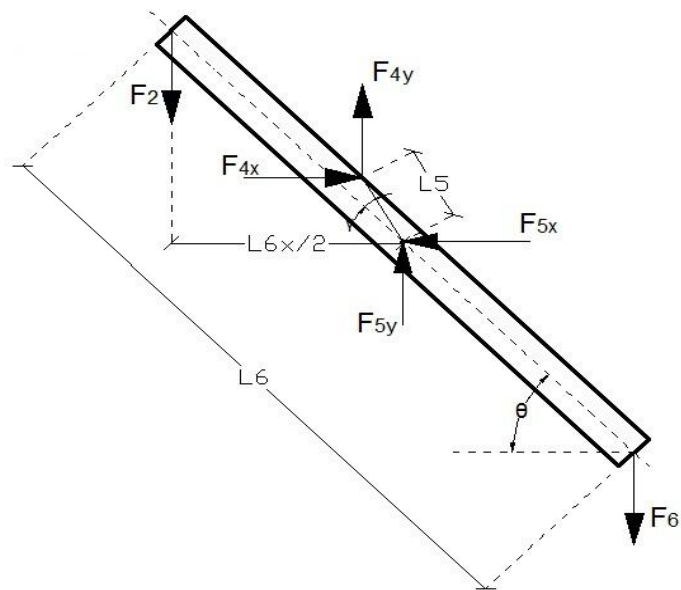
Figura 4-5 FUERZAS QUE ACTÚAN SOBRE LA BARRA 3
