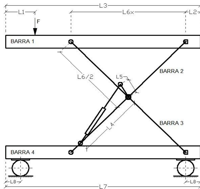
Figura 4-2 GEOMETRÍA DE LA PLATAFORMA.
