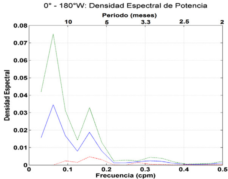
Figura 9. Densidad de Energía Espectral para el punto de grilla 0°-180°W (datos mensuales). La densidad espectral está en m^2/cpm . La línea azul es el espectro. Los límites de confianza del 95% están representados por las líneas verde y roja.
