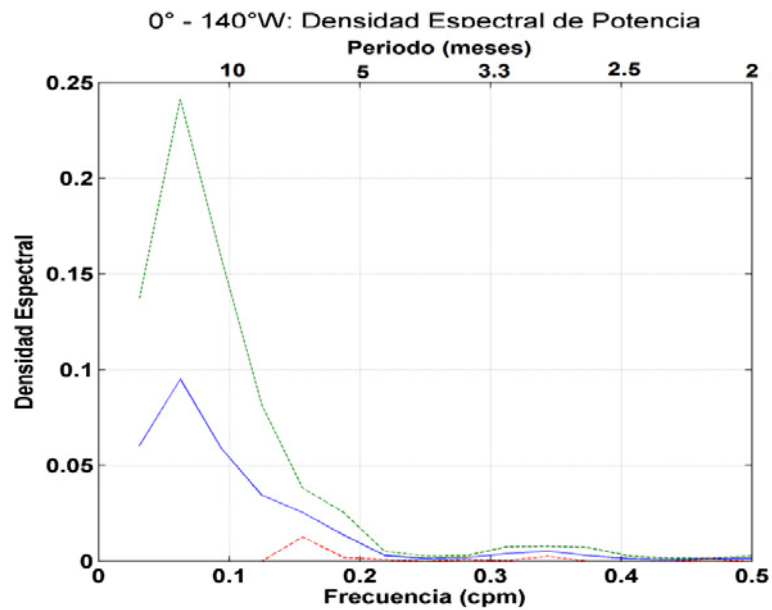
Figura 8. Densidad de Energía Espectral para el punto de grilla 0^{\circ} - 140^{\circ} W (datos mensuales). La densidad espectral está en m^2/cpm . La línea azul es el espectro. Los límites de confianza del 95% están representados por las líneas verde y roja.
