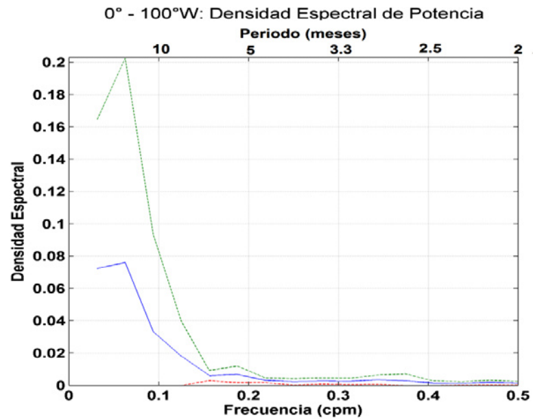
Figura 7. Densidad de Energía Espectral para el punto de grilla 0^{\circ} - 100^{\circ} W (datos mensuales). La densidad espectral está en m^2/cpm . La línea azul es el espectro. Los límites de confianza del 95% están representados por las líneas verde y roja.
