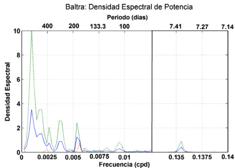
Figura 10. Densidad de Energía Espectral para la estación de Baltra (datos diarios). La densidad espectral está en m^2/cpd . La línea azul es el espectro. Los límites de confianza del 95% están representados por las líneas verde y roja.
