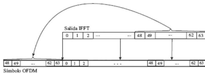
Inserción del prefijo Cíclico.
