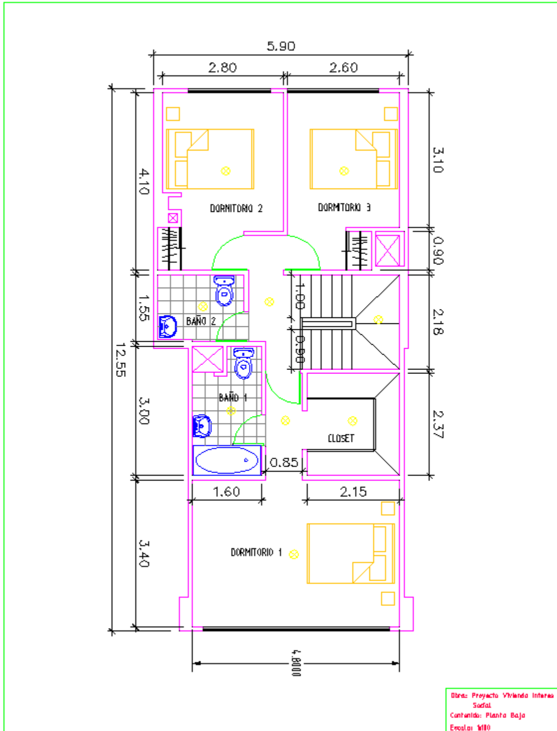
Figura 22.- Planta Alta
