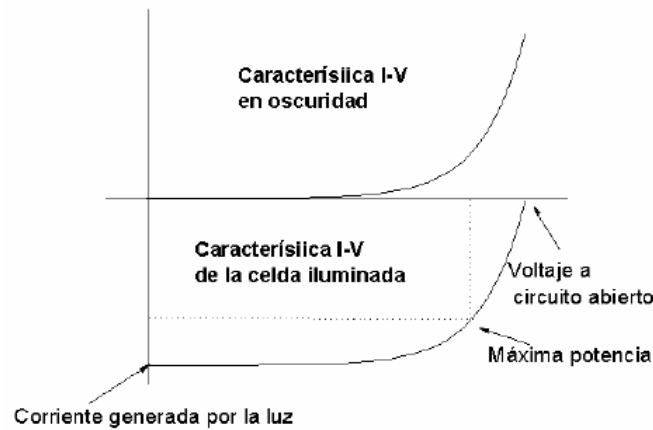
Figura 29.- Dependencia I-V de una celda solar en oscuridad y bajo iluminación
