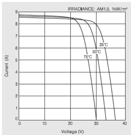
Figura 33.- Intensidad vs Voltaje a varias temperaturas de la celda.
