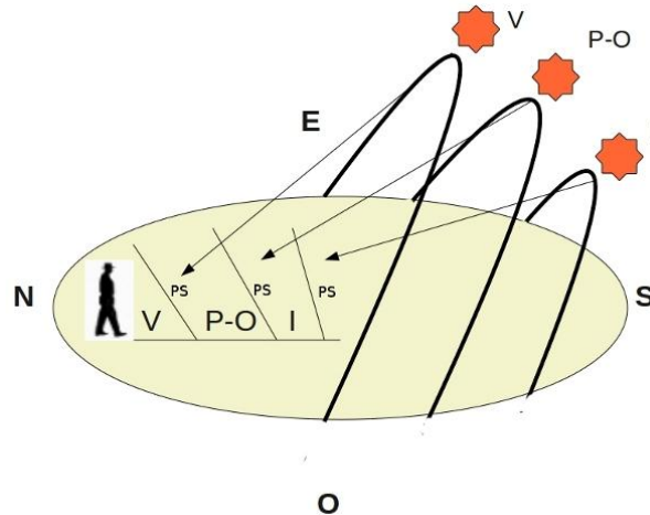
Figura 30.- Diferentes inclinaciones del panel dependiendo de la estación
