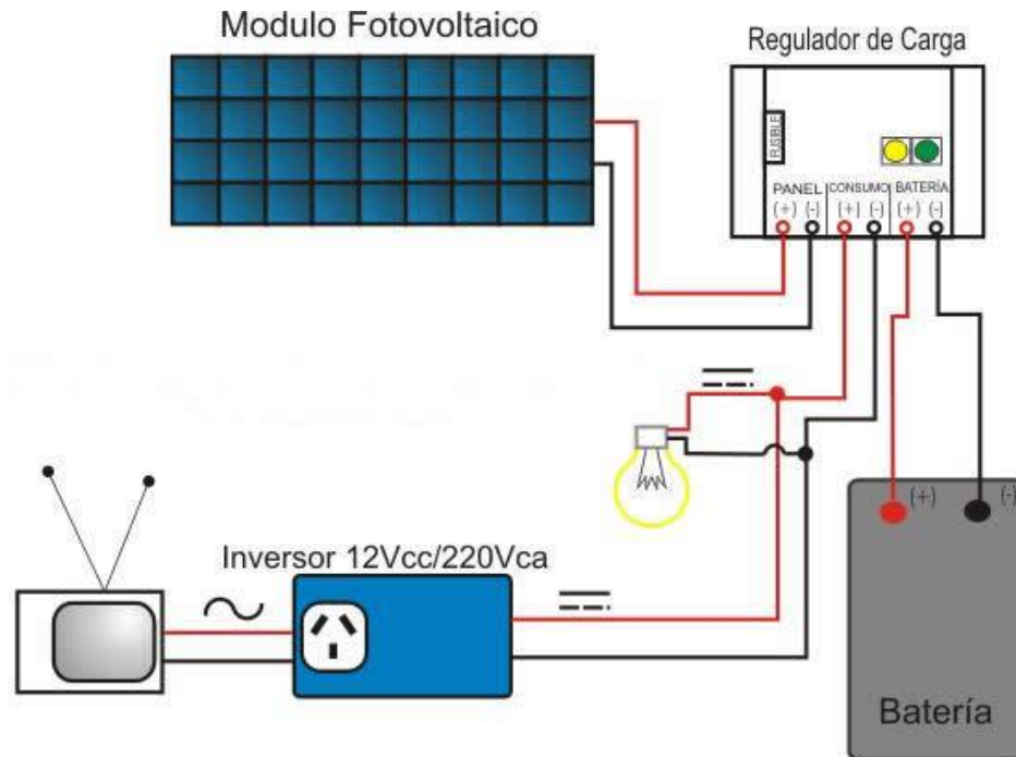
Figura 32.- Sistema solar fotovoltaico
