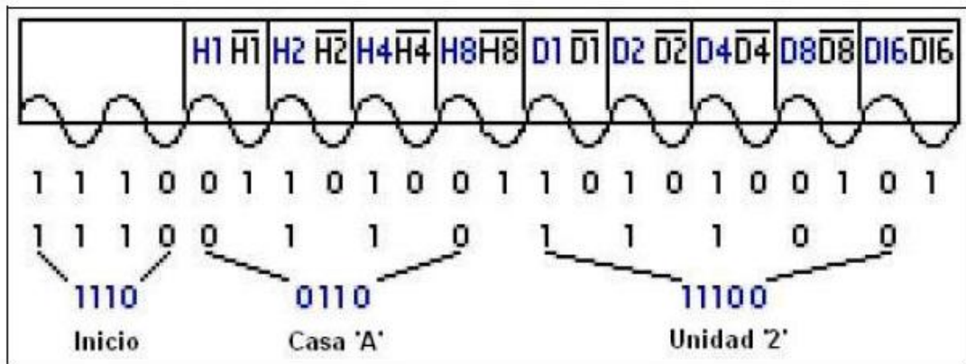
Figura 14.- Trama de X-10
