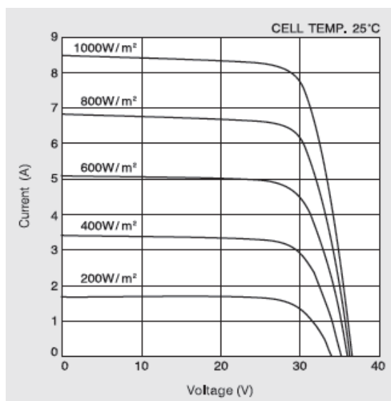
Figura 34.- Intensidad vs Voltaje a varios niveles de irradiancia.
