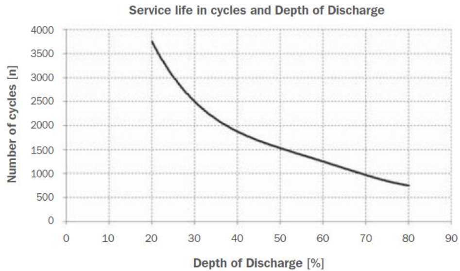
Figura 38.- Curva de profundidad de descarga y tiempo de vida en ciclos
