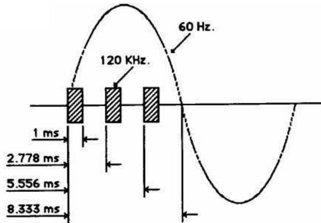
Figura 13.- Relación entre los pulsos y el punto cero de la corriente alterna
