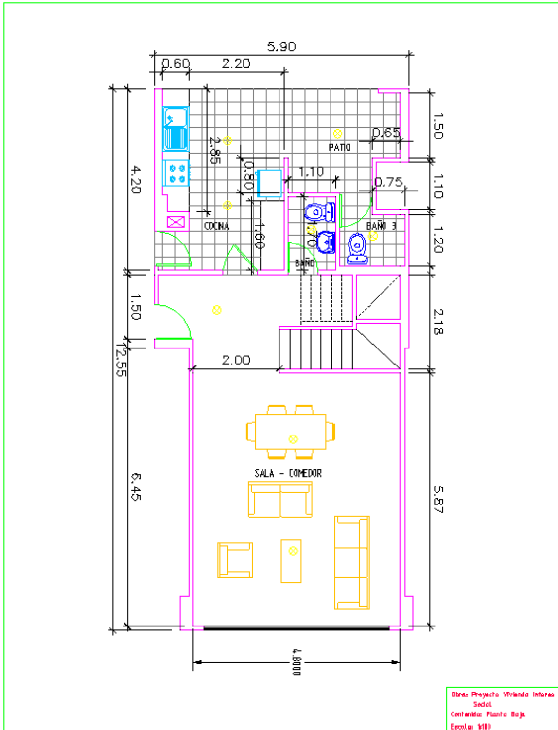
Figura 21.- Planta Baja
