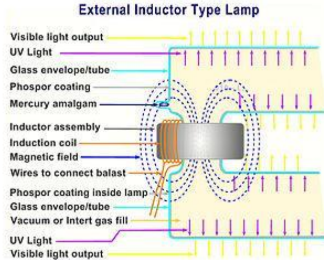
Figura 2.- Lámpara de Inducción Externa
