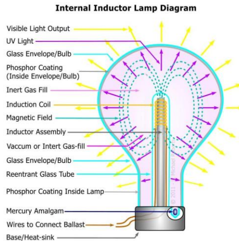
Figura 1.- Lámpara de Inducción Interna
