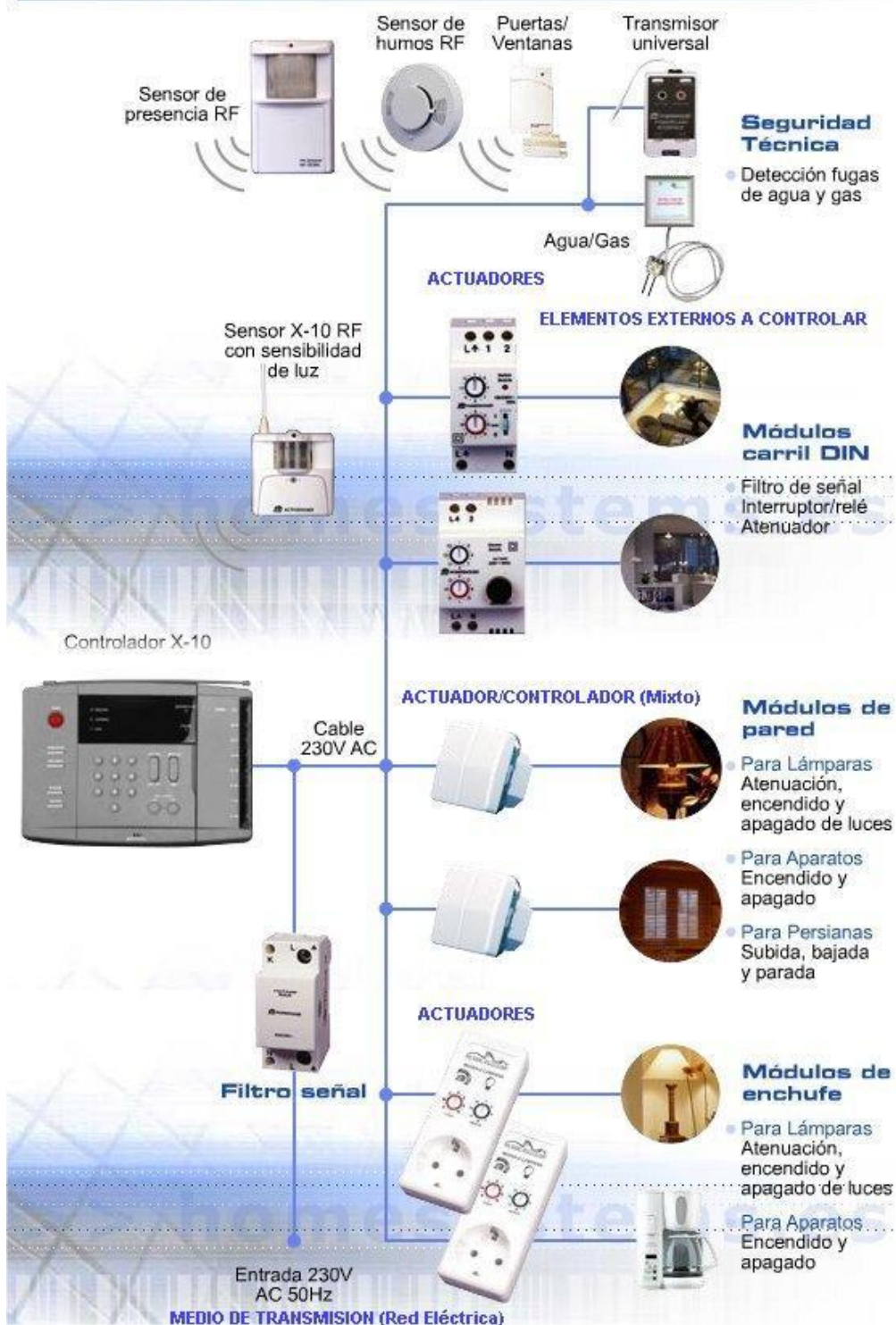
Figura 15.- Estructura de un sistema doméstico X-10
