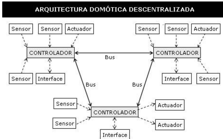
Figura 7.- Arquitectura descentralizada
