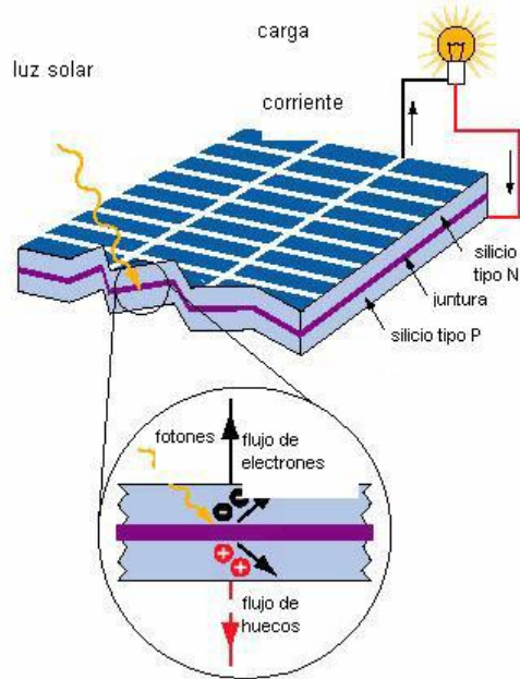
Figura 28.- Estructura de una celda solar de silicio
