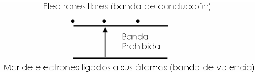
Figura 26.- Representación esquemática del diagrama de bandas de un semiconductor
