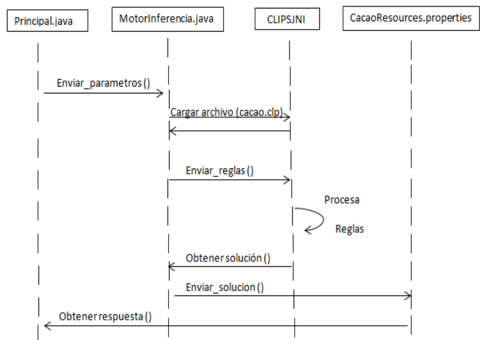
Figura 2.5: Mecanismo de Inferencia
