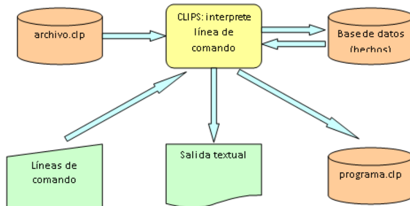
Figura 2.2: Estructura General de CLIPS
