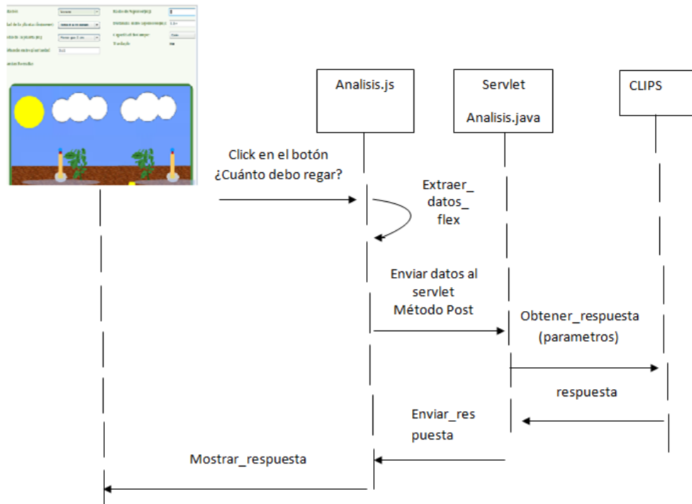
Figura 2.9: Funcionamiento de la Página de Análisis de EXPCAC
