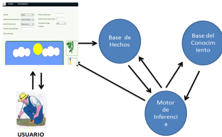
Figura 2.4: Estructura General del Sistema Experto EXPCAC
