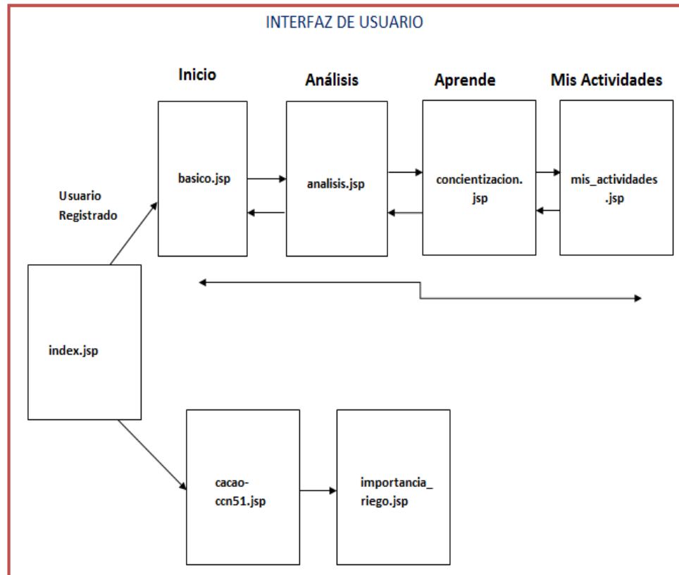
Figura 2.6: Diseño General de la Interfaz de Usuario
