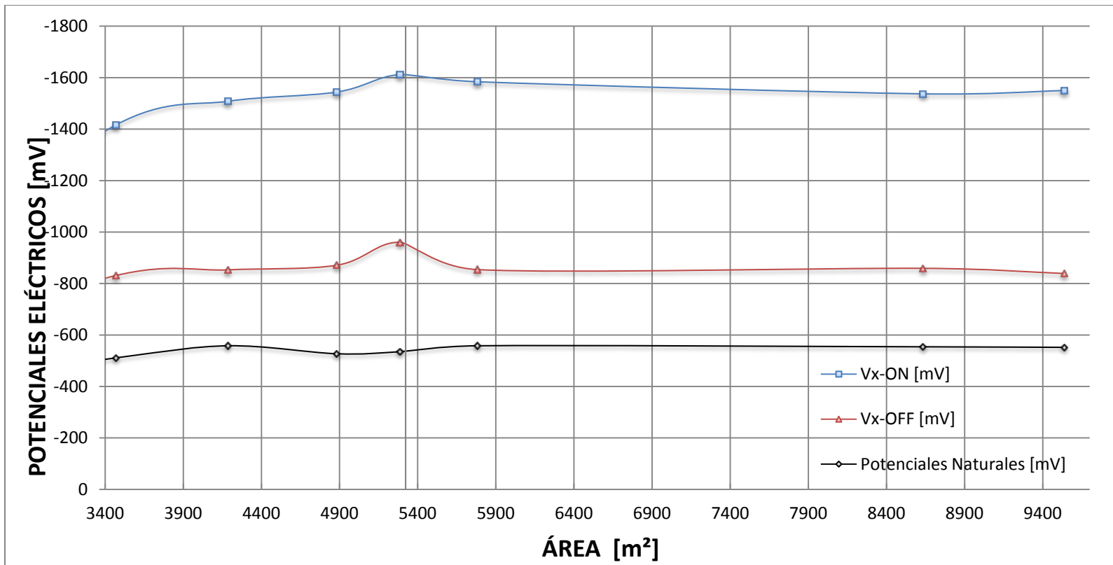
FIG. 3.4. DISTRIBUCIÓN DE POTENCIALES EN PRUEBA DE CONDUCTANCIA ELÉCTRICA DEL RECUBRIMIENTO EN FUNCIÓN DEL ÁREA SUPERFICIAL
