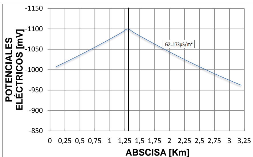
FIG. 3.11. DISTRIBUCIÓN DE POTENCIALES ELÉCTRICOS CON ALIMENTACIÓN EN ABSCISA SELECCIONADA
