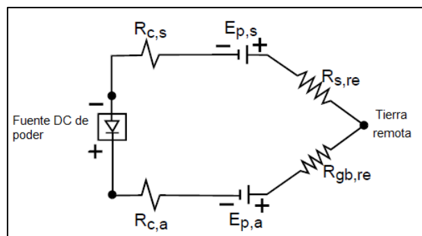
FIG. 2.8. CIRCUITO DEL SISTEMA DE PROTECCIÓN CATÓDICA PARA TUBERÍAS ENTERRADAS
