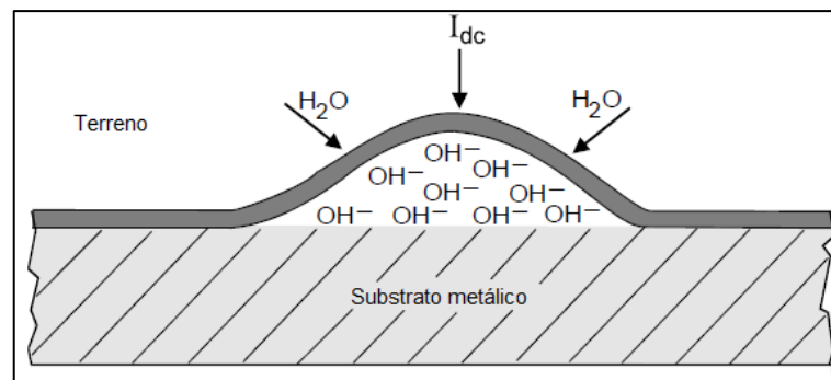
FIG. 1.9. AMPOLLAMIENTO DEL RECUBRIMIENTO
