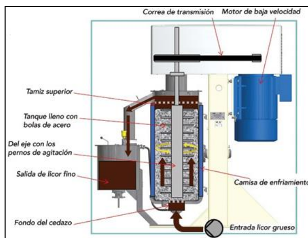
FIGURA 1.18 MOLINO DE BOLAS HORIZONTAL
