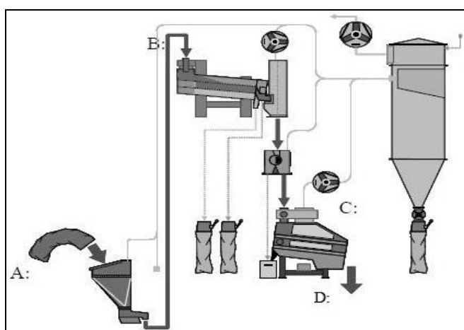
FIGURA 1.12 PROCESO DE LIMPIEZA DE CACAO
