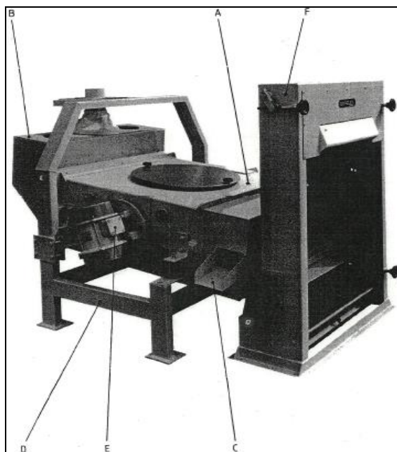
FIGURA 1.13 CLASIFICADORA DE HABAS DE CACAO FUENTE: (Buhler Barth AG, 1986)
