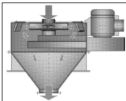
FIGURA 1.16 DESCASCARADO, MARTILLO ROMPEDOR FUENTE: (Buhler Barth AG, 1986)
