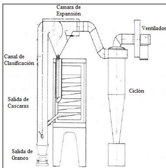
FIGURA 1.17 SISTEMA DE EXPANSIÓN
