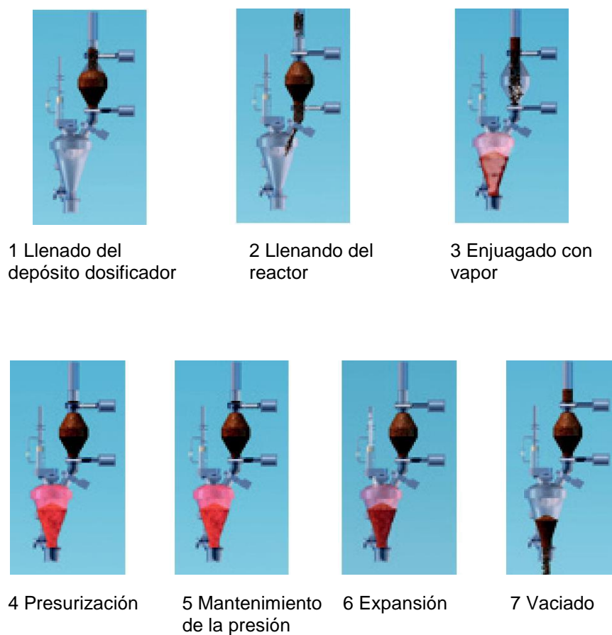
FIGURA 1.15 PROCESOS DE DESBACTERIZACIÓN
