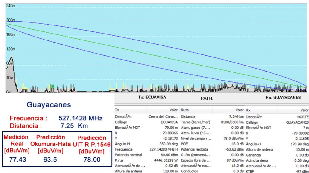
Figura 4.27:Medición punto fijo Ecuavisa – Guayacanes
