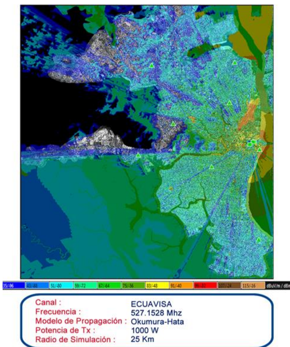
Figura 4.7.: Resultado predicción Okumura-Hata Ecuavisa
