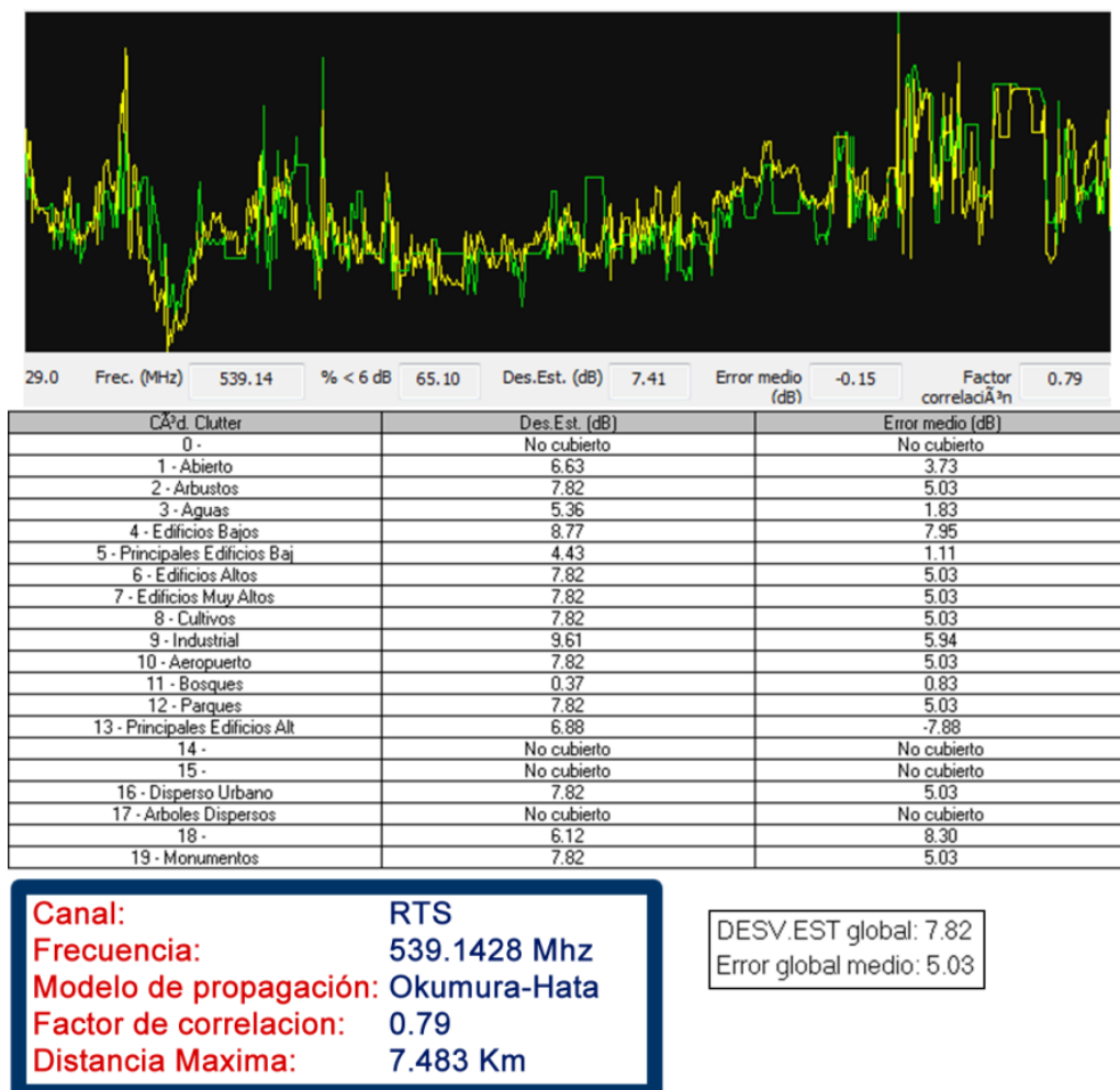
Figura 4.17: Correlación, medición real Vs Okumura Hata RTS recorrido 2
