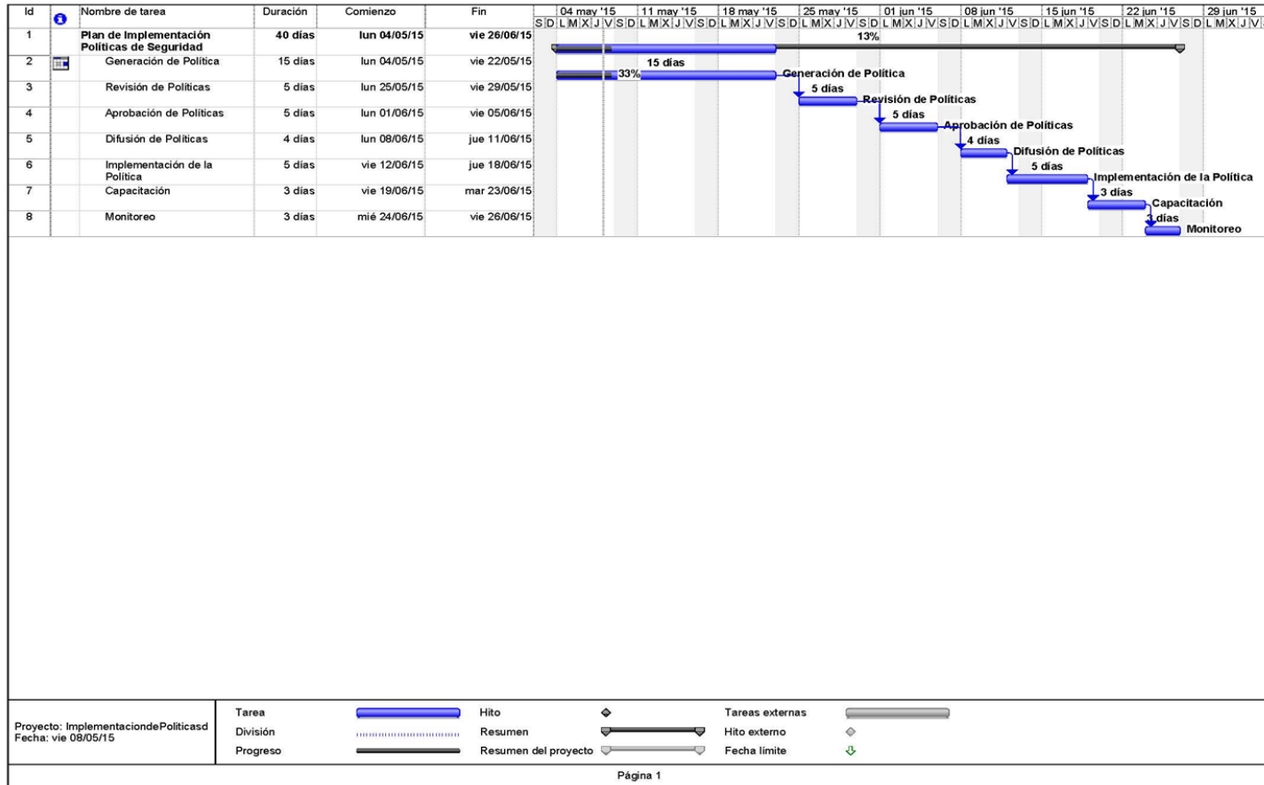
Figura 5-64. Diagrama GANTT
