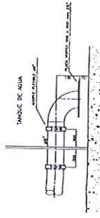
DETALLE PLACA VORTEX ESC. 1/4"
