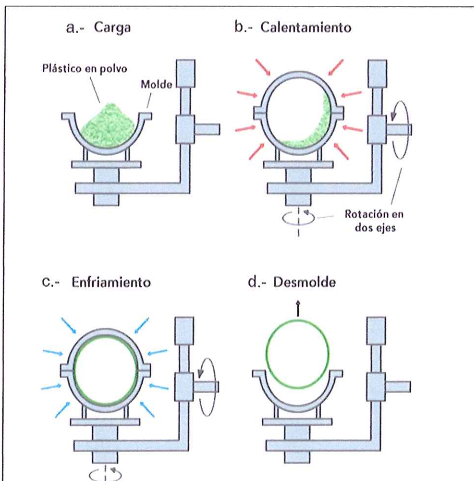
FIGURA 1.1 PASOS BÁSICOS DEL PROCESO DE ROTO-MOLDEO [1]
