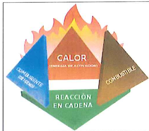
FIGURA 1.2. TETRAEDRO DEL FUEGO [3]
