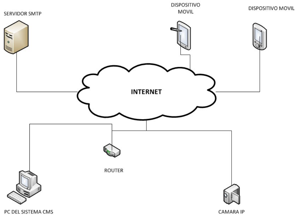
Fig. 3.5.4.1 Modulo de envío mediante SMTP
