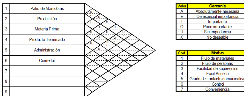
Figura 3.11 Diagrama de Relaciones Planta Puré de Banano.
