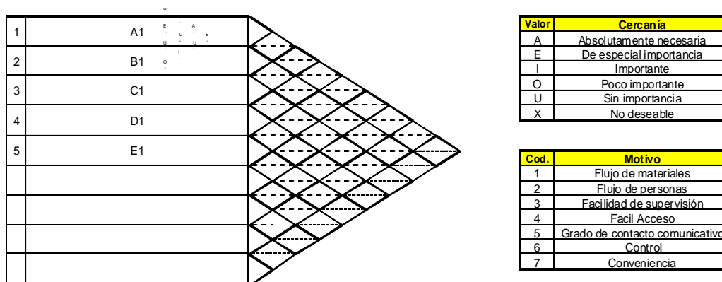
Figura 1.1 Diagrama de Relaciones de SPL.
