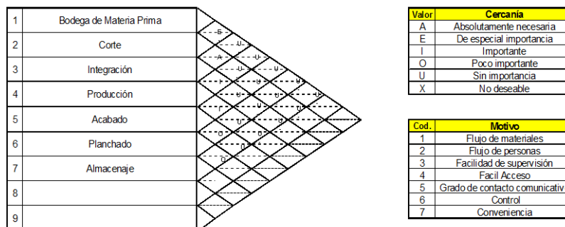
Figura 3.18 Diagrama de Relaciones Planta de Plásticos.
