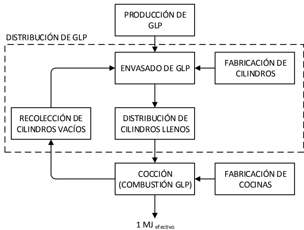
FIGURA 4.1 LÍMITES DEL SISTEMA DE COCCIÓN CON GLP
