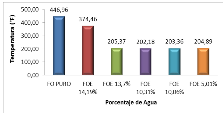
FIGURA 4.8 GRÁFICO COMPARACIÓN DE LAS TEMPERATURA DE GASES DE ESCAPE CON FO Y FOE.
