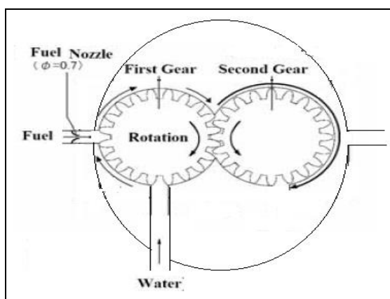
FIGURA 3.7 – DISPOSITIVO DIRECCION (JUEGO DOS ENGRANES) FUENTE [1]
