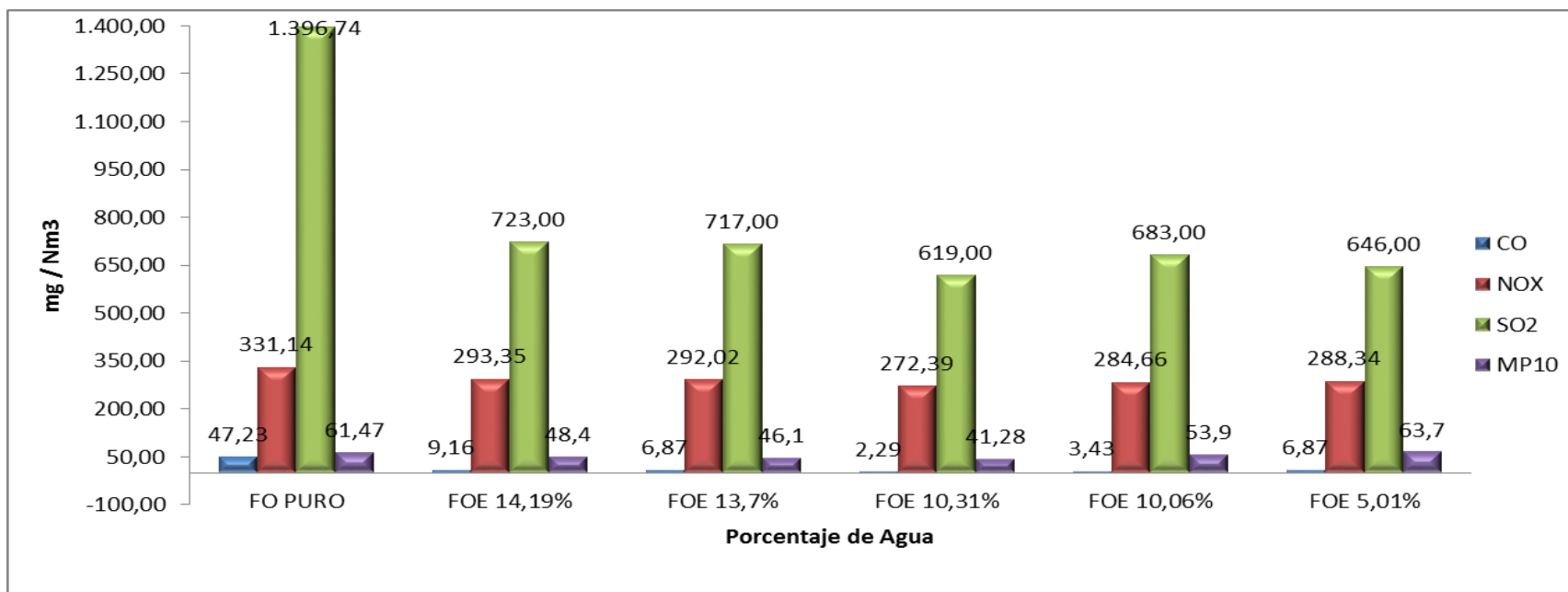
FIGURA 4.7 GRAFICO DE COMPARACIÓN DE LAS EMISIONES DE GASES Y MATERIAL PARTICULADO DEL FO Y FOE CON DIFERENTES PORCENTAJES DE AGUA.
