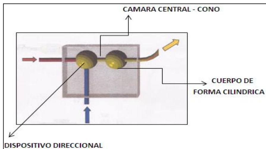
FIGURA 3.6 - CIRCUITO GENERAL EMULSOR ESTATICO O TURBOTRANSDUCTOR. FUENTE [1]
