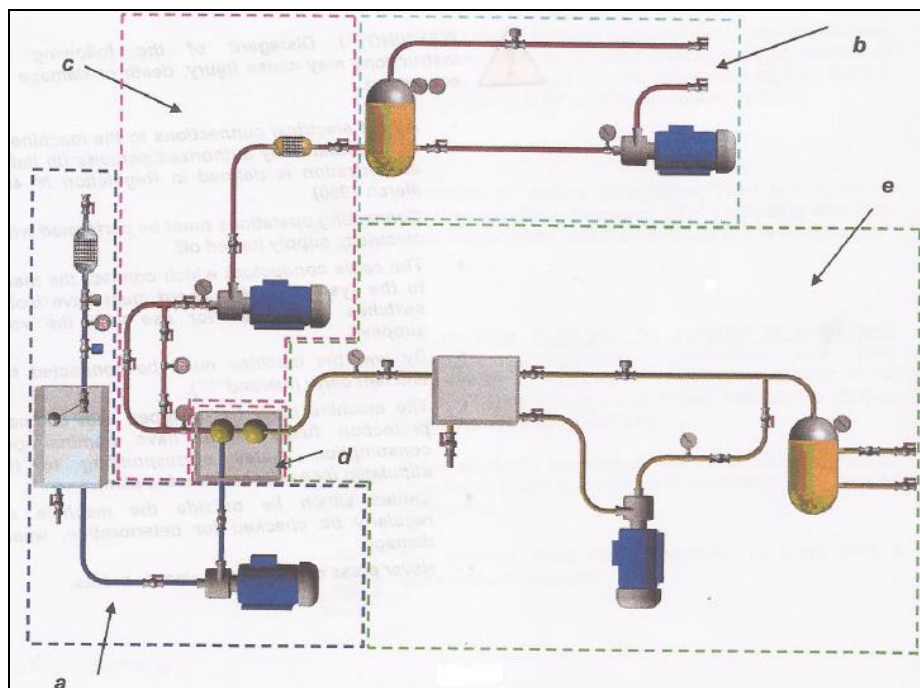
FIGURA 3.2 – CIRCUITO GENERAL DE PROCESO DE PRODUCCIÓN DE LA MICROEMULSIÓN. FUENTE [1]
