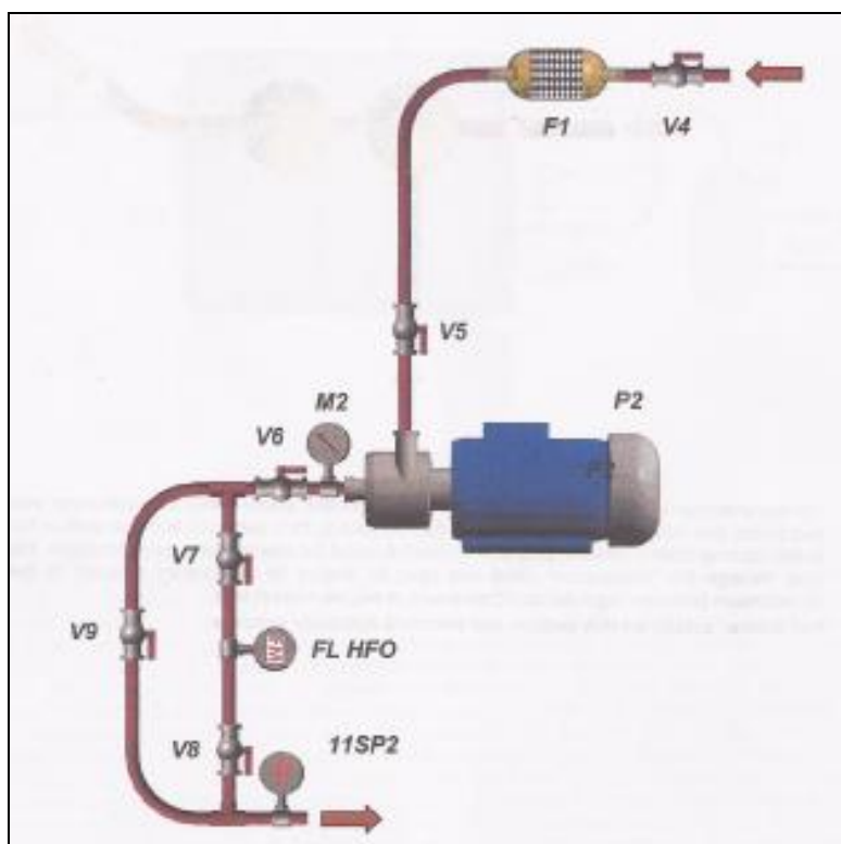
FIGURA 3.5 - CIRCUITO GENERAL PRESURIZADO DE COMBUSTIBLE (CIRCUITO REFORZADOR). FUENTE [1]
