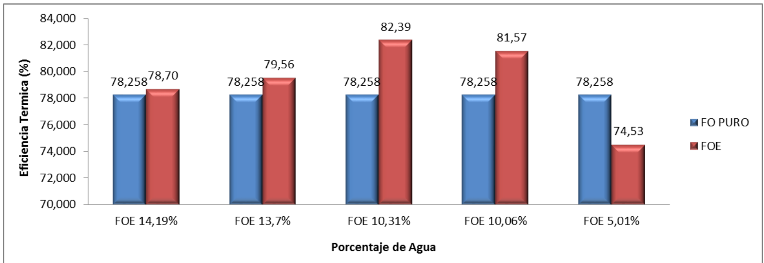
FIGURA 4.5 GRÁFICO DE COMPARACIÓN DE LA EFICIENCIA TÉRMICA – OPERATIVA DEL FO Y FOE CON DIFERENTES PORCENTAJES DE AGUA.
