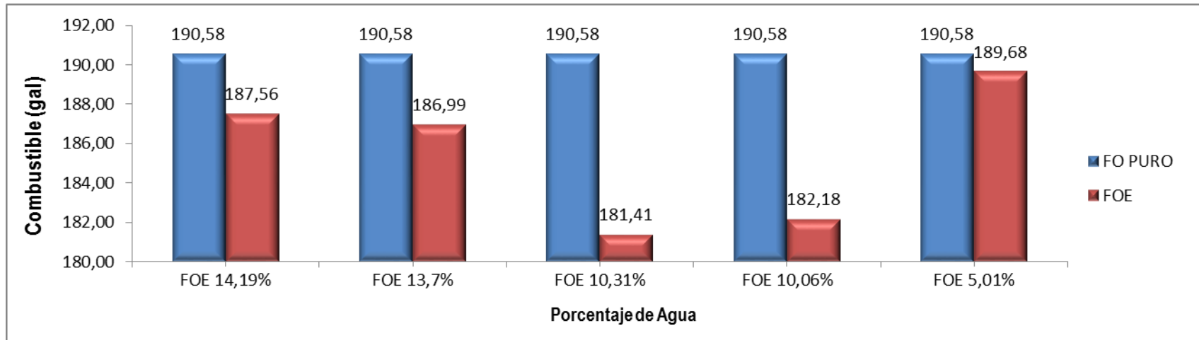
FIGURA 4.1 GRÁFICO DE COMPARACIÓN DEL CONSUMO PROMEDIO DEL FO Y FOE CON DIFERENTES PORCENTAJES DE AGUA.
