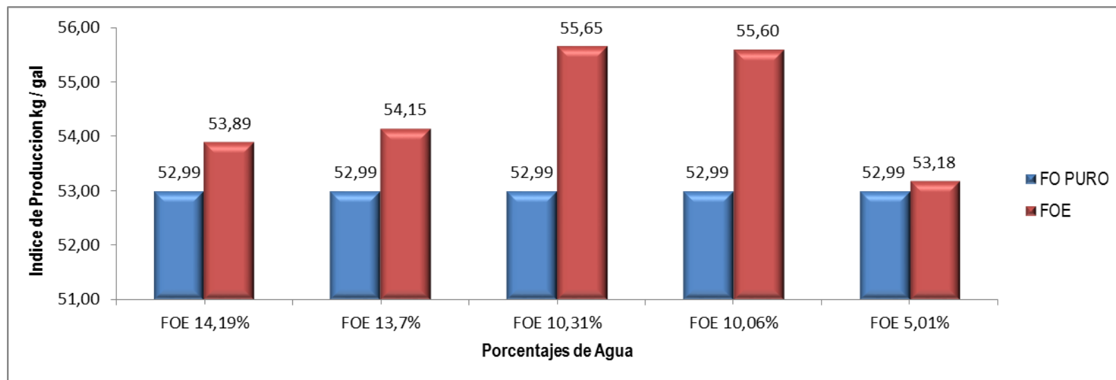
FIGURA 4.3 GRÁFICO DE COMPARACIÓN DEL ÍNDICE DE PRODUCCIÓN DEL FO Y FOE CON DIFERENTES PORCENTAJES DE AGUA.
