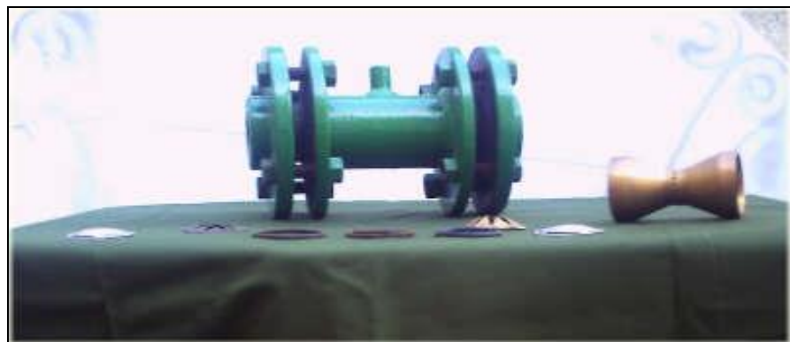
FIGURA 3.8 – CONO DE LA CAMARA CENTRAL DEL EMULSOR ESTATICO DE FLUJO LAMINAR. FUENTE [2]
