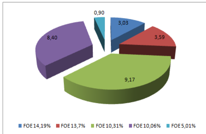
Ahorro de Fuel Oil N°4 en gal/h.
