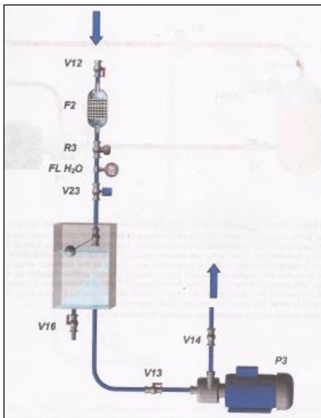
FIGURA 3.3 - CIRCUITO GENERAL DE AGUA DE ALIMENTACIÓN PRESURIZADO. FUENTE [1]
