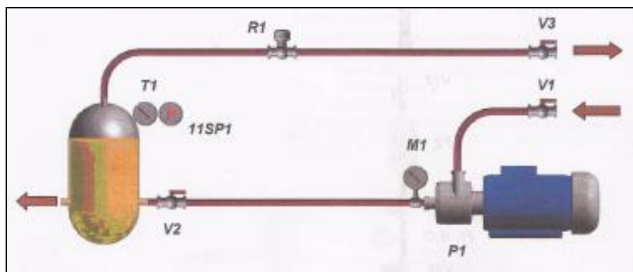
FIGURA 3.4 - CIRCUITO GENERAL DE ALIMENTACIÓN DEL FUEL OIL. FUENTE [1]
