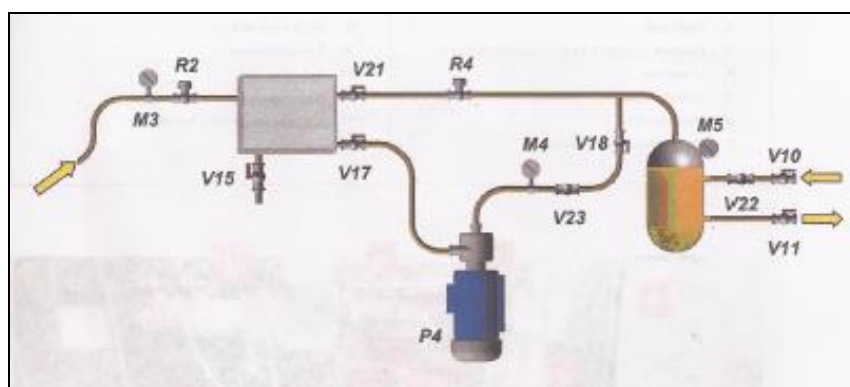
FIGURA 3.9 - CIRCUITO GENERAL DEL ANILLO QUEMADOR.
