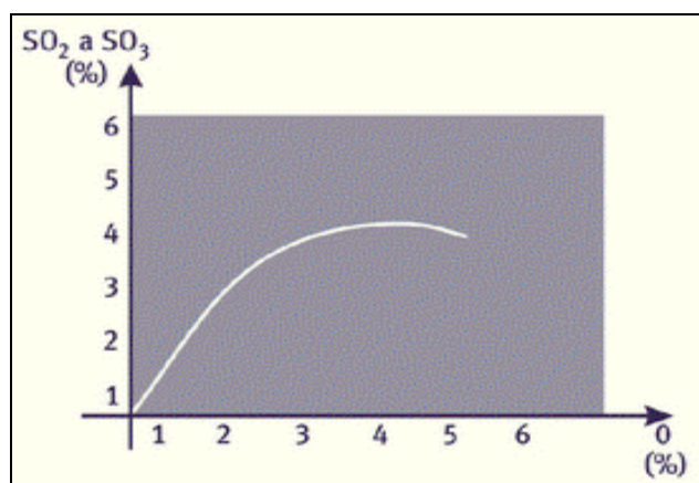
FIGURA 1.14 RELACIÓN ENTRE EL OXÍGENO Y LOS COMPUESTOS \text{SO}_2 Y \text{SO}_3 . FUENTE [2]
