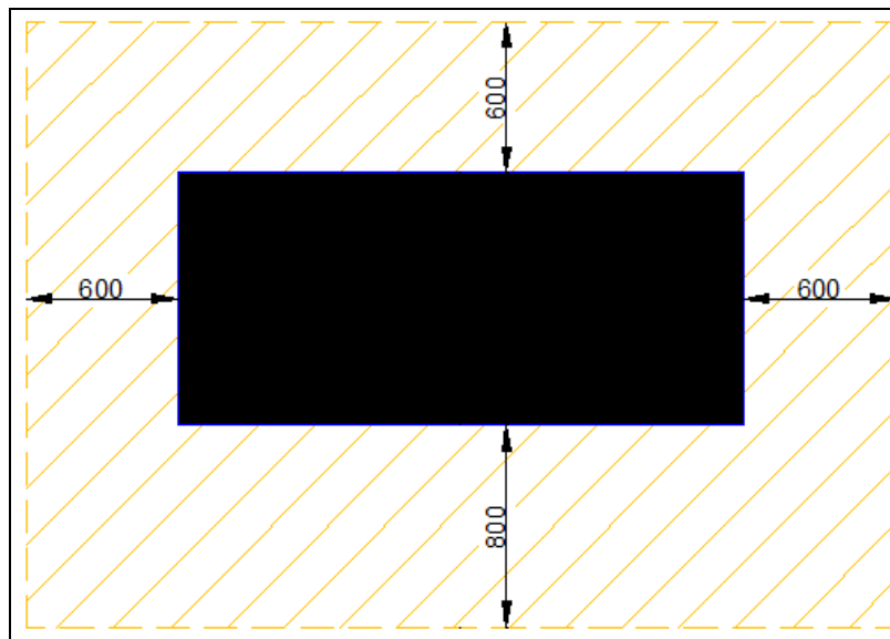
FIGURA 3.1 - ÁREA DE INSTALACIÓN (ESPACIOS LIBRES) DE LA UNIDAD MICRO – EMULSIFICADORA, UNIDADES EN MILÍMETROS. FUENTE [1]
