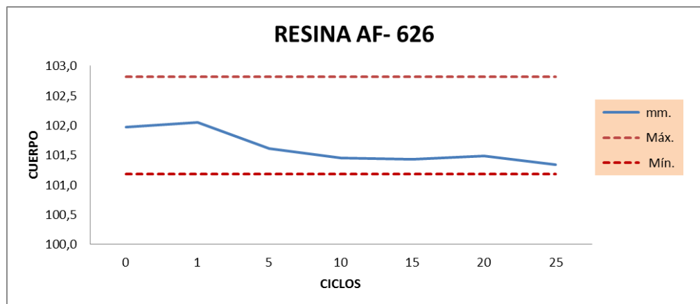
FIGURA 3.7 GRÁFICO COMPORTAMIENTO DE LA RESINA AF-626 SEGÚN EL CUERPO DEL ENVASE.
