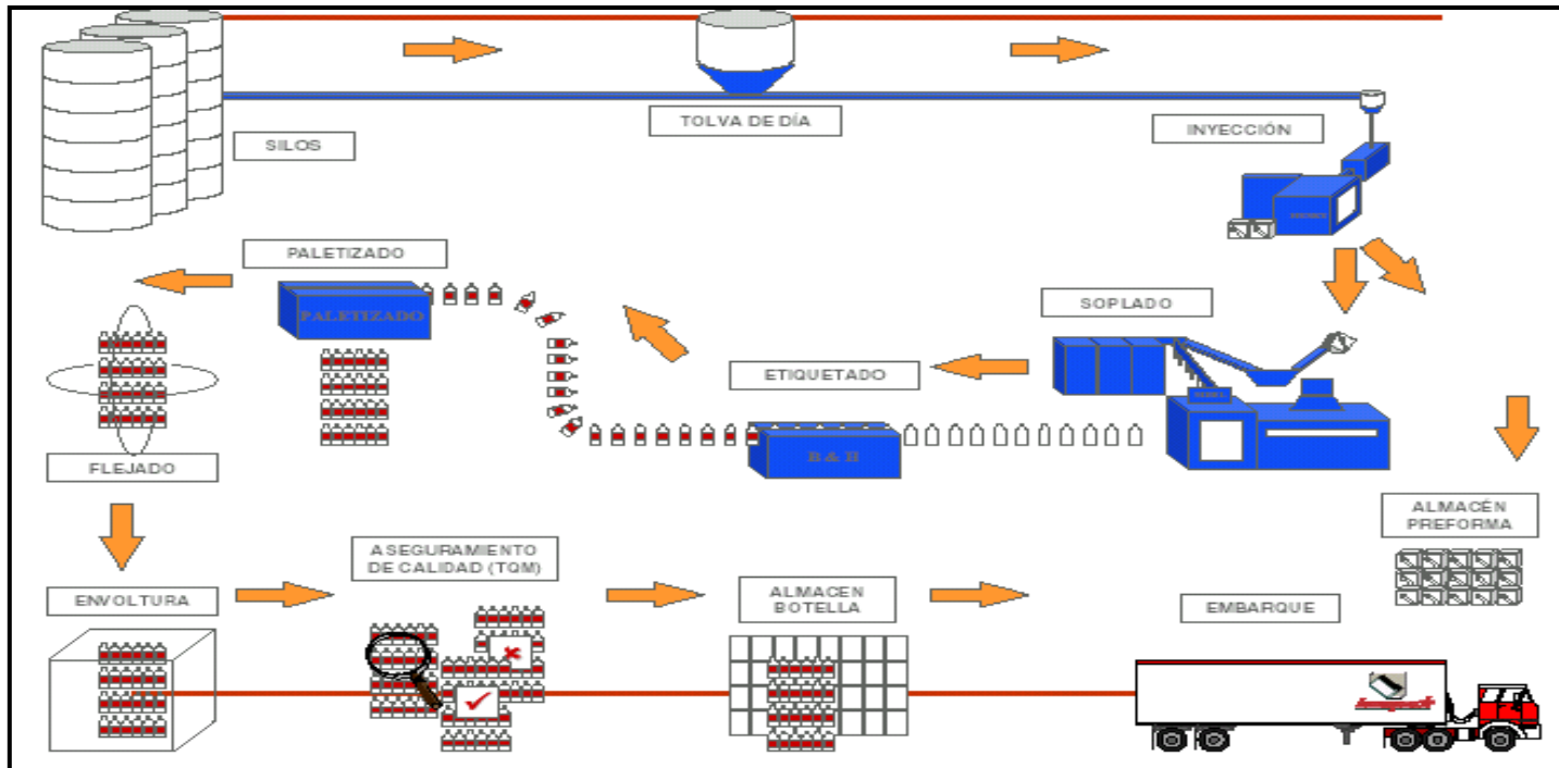
FIGURA 2.1. LAYOUT DEL PROCESO FABRICACIÓN DE BOTELLAS PET- RETORNABLE.
