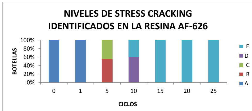
FIGURA 3.12 GRÁFICO NIVELES DE STRESS CRACKING EN LOS ENVASES DE LA RESINA AF-626.
