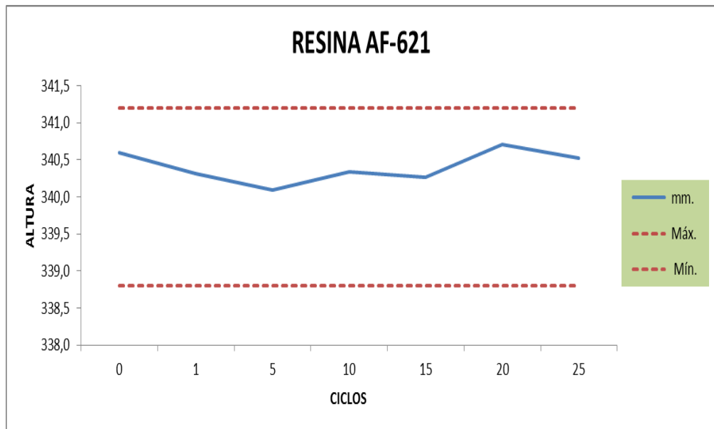
FIGURA 3.4 GRÁFICO COMPORTAMIENTO DE LA RESINA AF-621 SEGÚN LA ALTURA DEL ENVASE.
