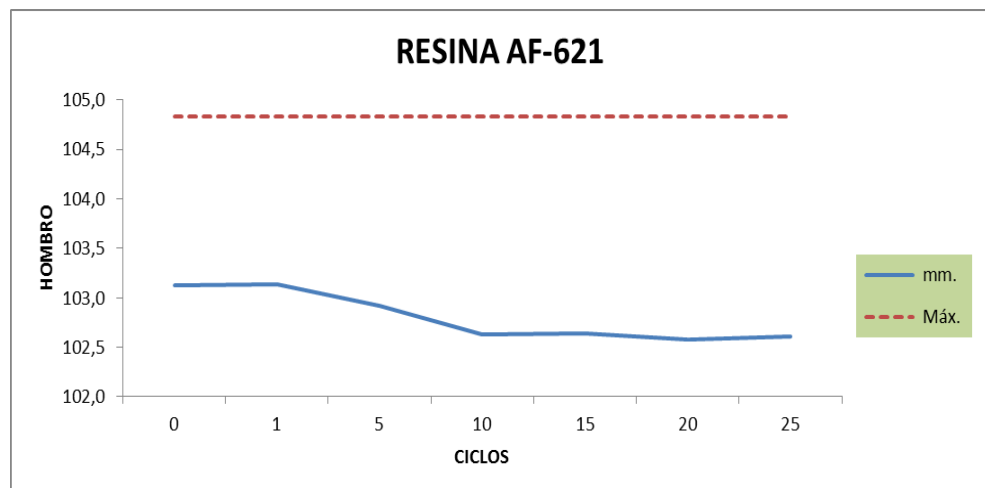
FIGURA 3.5 GRÁFICO COMPORTAMIENTO DE LA RESINA AF-621 SEGÚN EL HOMBRO DEL ENVASE.
