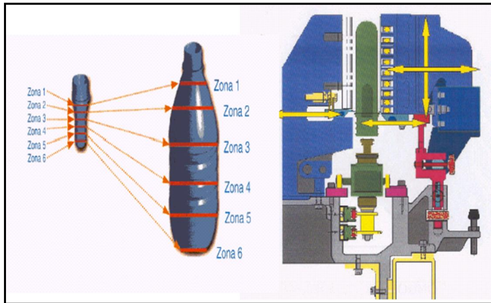
FIGURA 2.5. TRANSFORMACIÓN DE PREFORMA A BOTELLA MEDIANTE EL PROCESO DE SOPLADO DEL PET-RETORNABLE.
