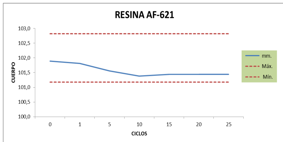
FIGURA 3.8 GRÁFICO COMPORTAMIENTO DE LA RESINA AF-621 SEGÚN EL CUERPO DEL ENVASE.
