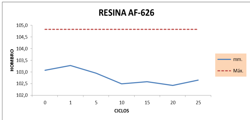
FIGURA 3.6 GRÁFICO COMPORTAMIENTO DE LA RESINA AF-626 SEGÚN EL HOMBRO DEL ENVASE.
