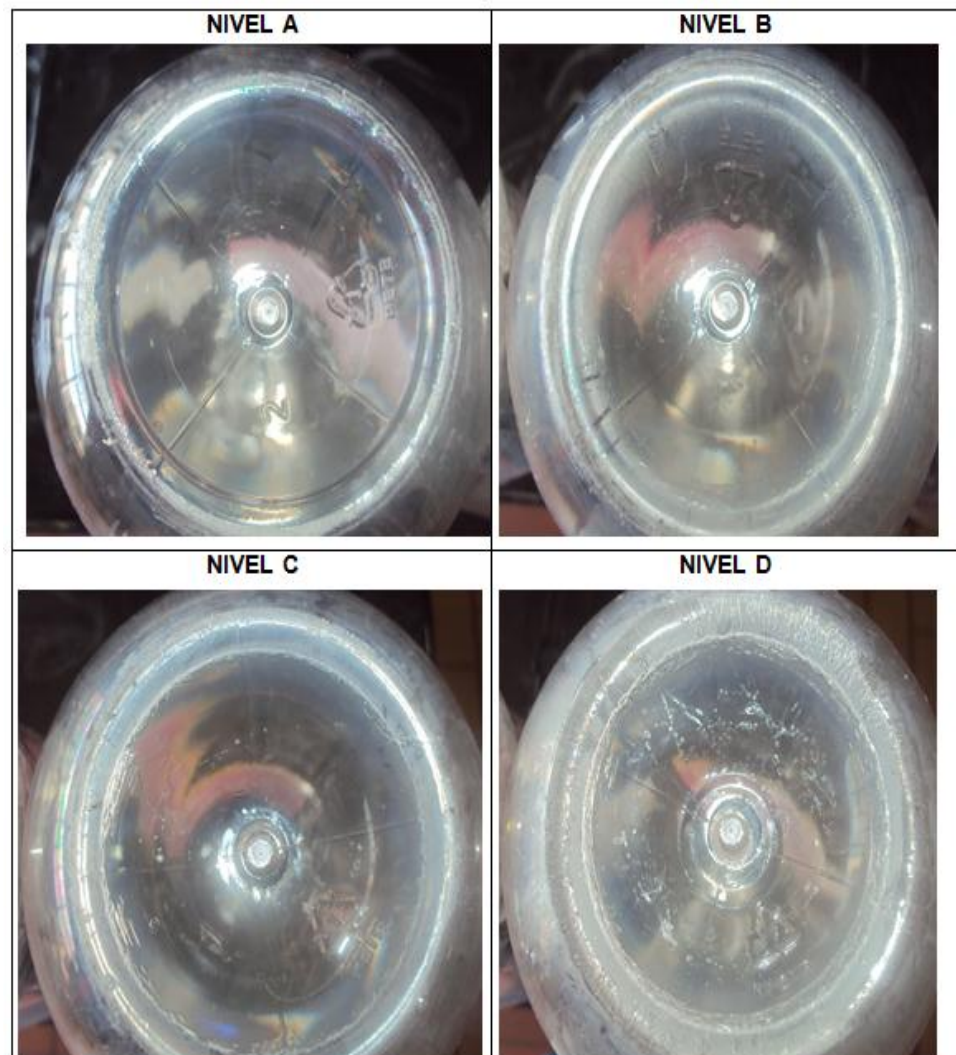
FIGURA 3.14. NIVELES DE STRESS CRACKING EN BOTELLAS PET RETORNABLES. RESINA AF- 626 Y AF-621.
