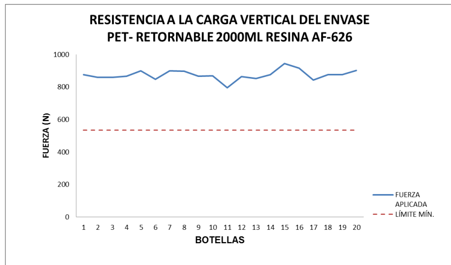
FIGURA 3.25 GRÁFICO RESISTENCIA A LA CARGA VERTICAL RESINA AF-626.
