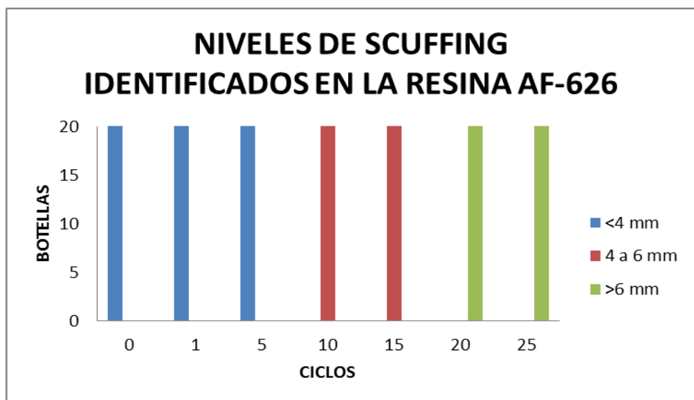
FIGURA 3.17 GRÁFICO PROCESO DE DESGASTE DEL ENVASE DE LA RESINA AF-626.
