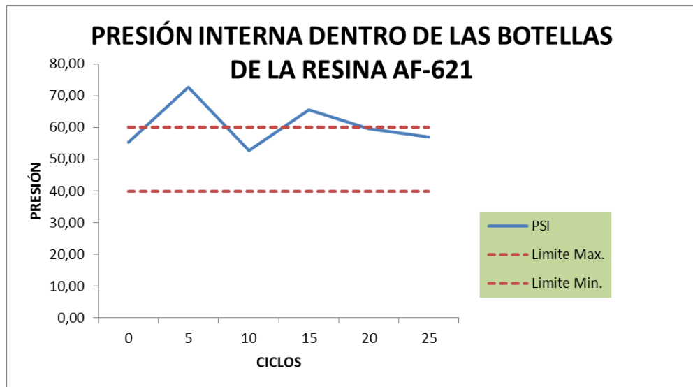
FIGURA 3.22 GRÁFICO COMPORTAMIENTO DE LA PRESIÓN INTERNA EN LOS ENVASES DE LA RESINA AF-621.
