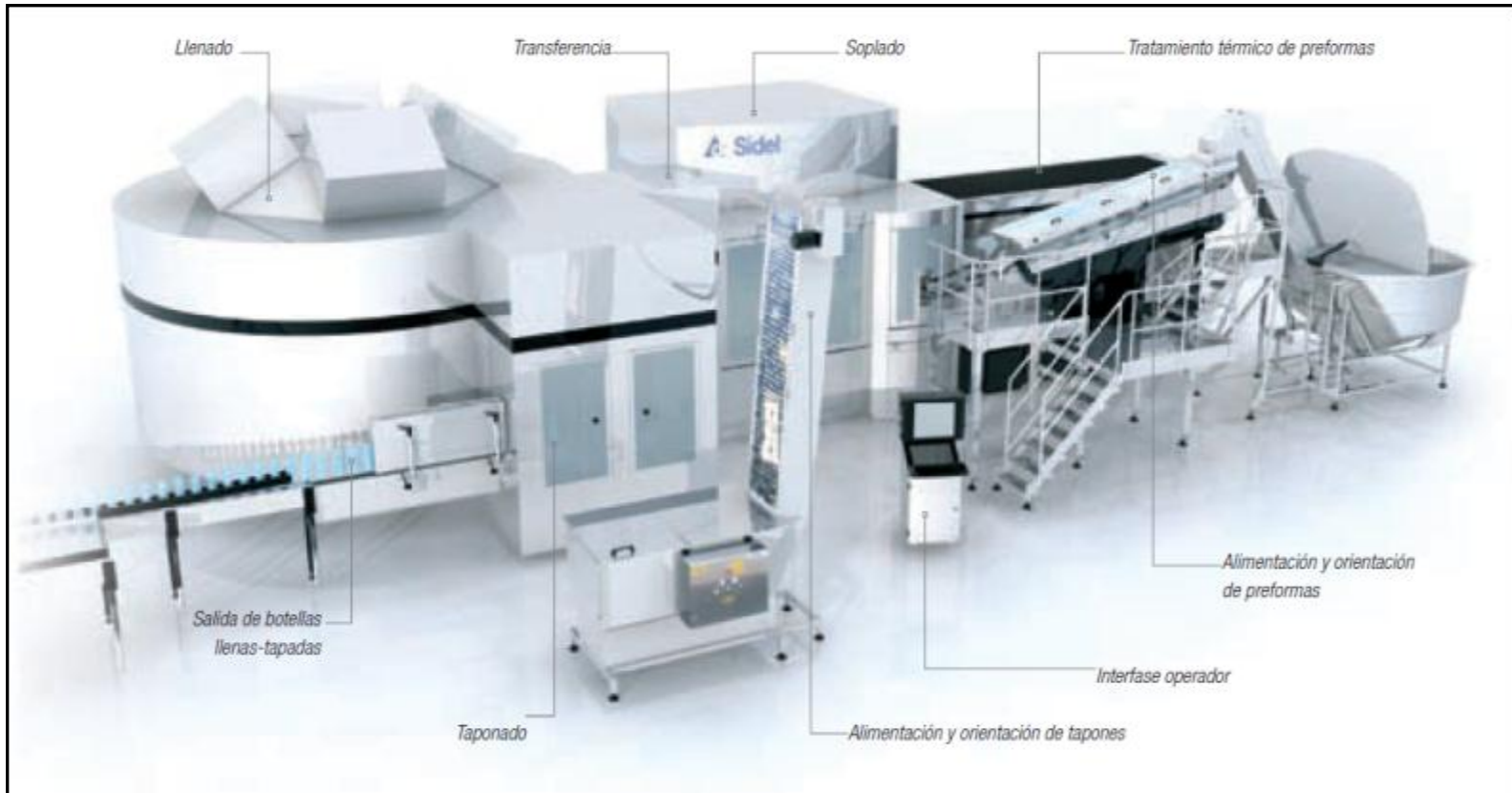
FIGURA 2.2 PROCESO DE SOPLADO Y ENVASADO DE BEBIDAS GASEOSAS EN LÍNEA.
