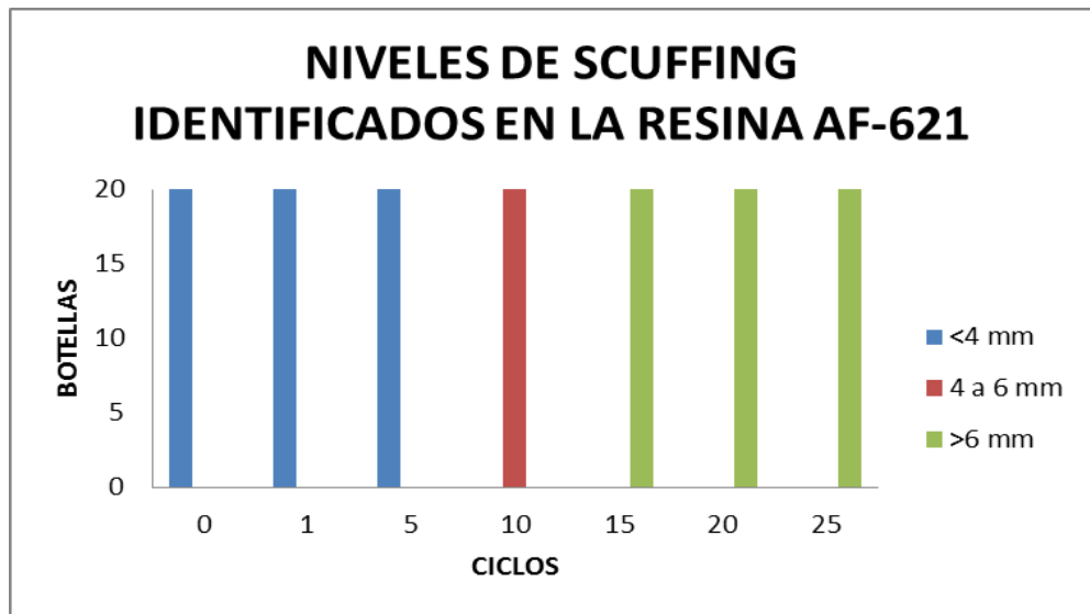
FIGURA 3.16 GRÁFICO PROCESO DE DESGASTE DEL ENVASE DE LA RESINA AF-621.
