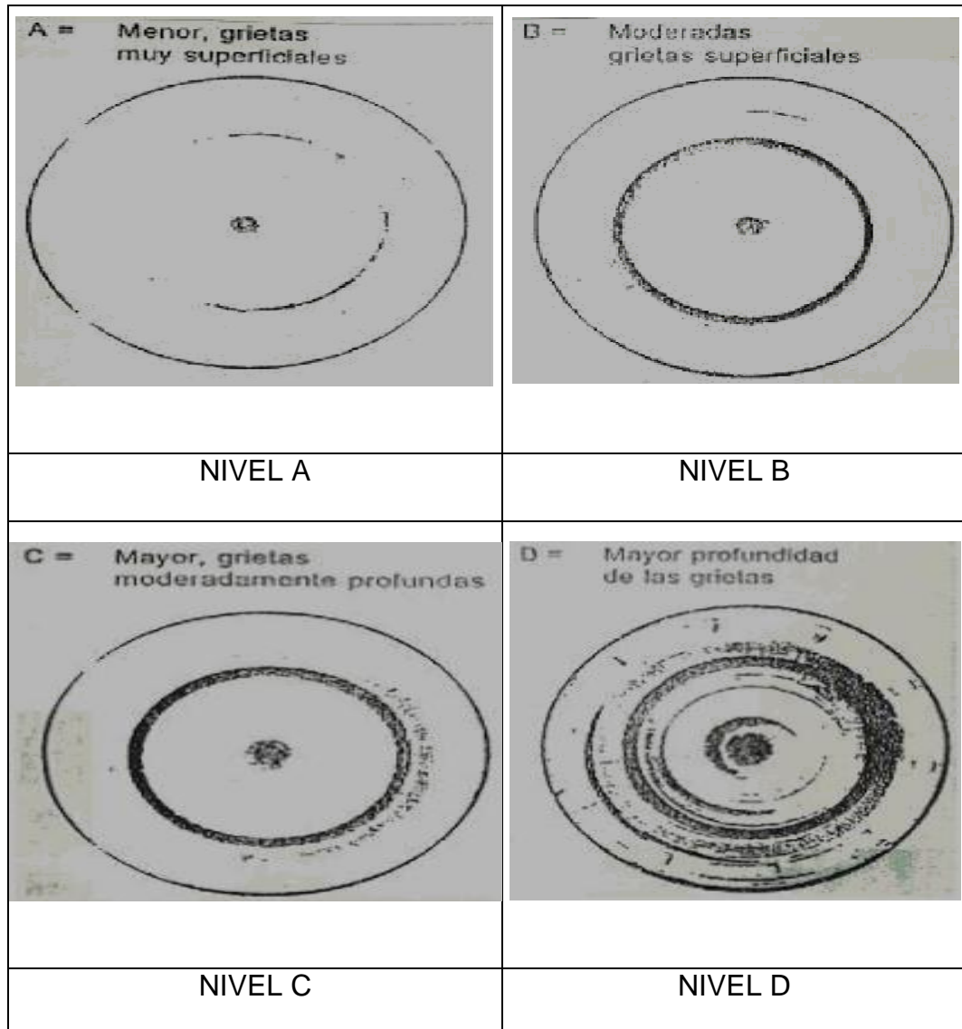
FIGURA 3.11. NIVELES DE STRESS CRACKING EN LA BASE DEL PET-RETORNABLE
