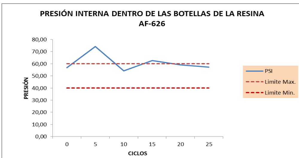
FIGURA 3.21 GRÁFICO COMPORTAMIENTO DE LA PRESIÓN INTERNA EN LOS ENVASES DE LA RESINA AF-626.
