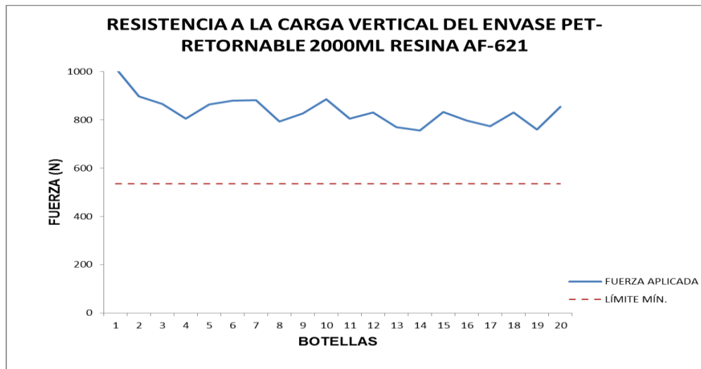
FIGURA 3.26 GRÁFICO RESISTENCIA A LA CARGA VERTICAL RESINA AF-621.
