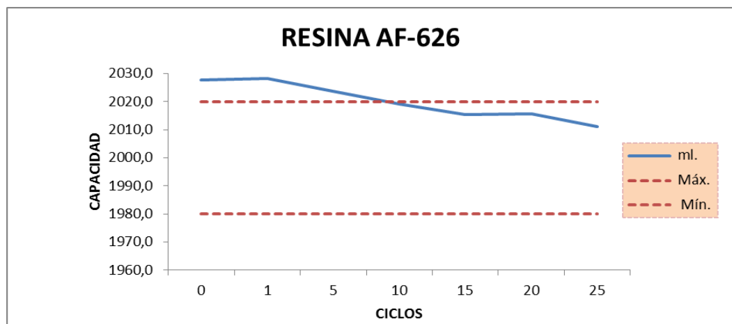
FIGURA 3.2 GRÁFICO COMPORTAMIENTO DE LA RESINA AF-626 SEGÚN LA CAPACIDAD DEL ENVASE.
