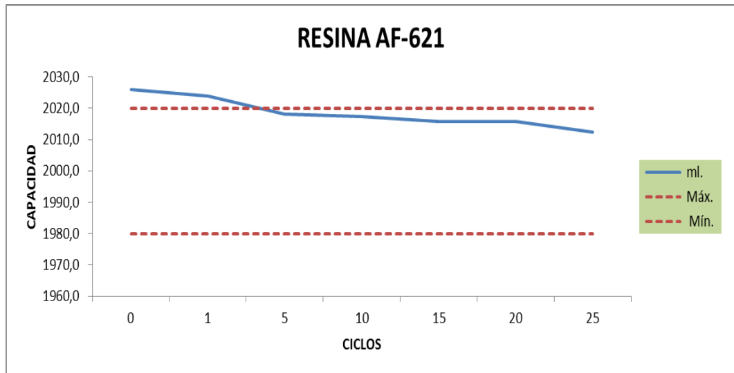
FIGURA 3.1 GRÁFICO COMPORTAMIENTO DE LA RESINA AF-621 SEGÚN LA CAPACIDAD DEL ENVASE.
