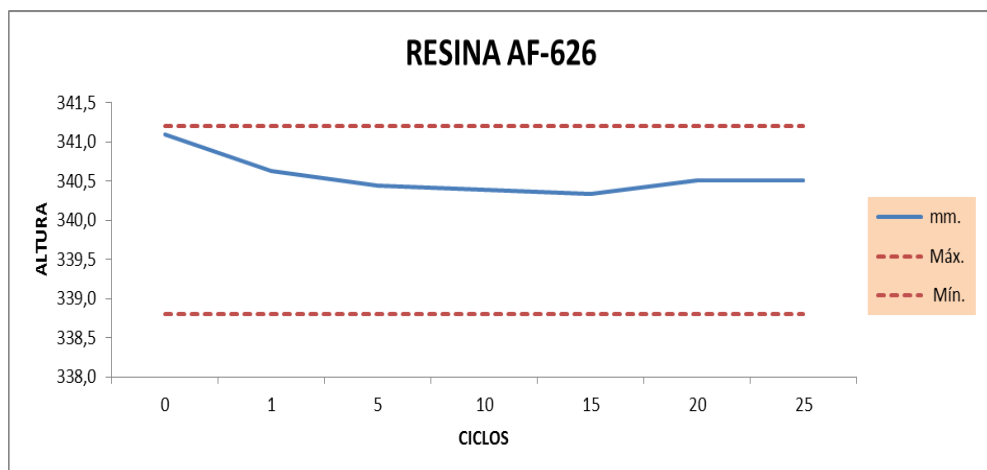
FIGURA 3.3 GRÁFICO COMPORTAMIENTO DE LA RESINA AF-626 SEGÚN LA ALTURA DEL ENVASE.
