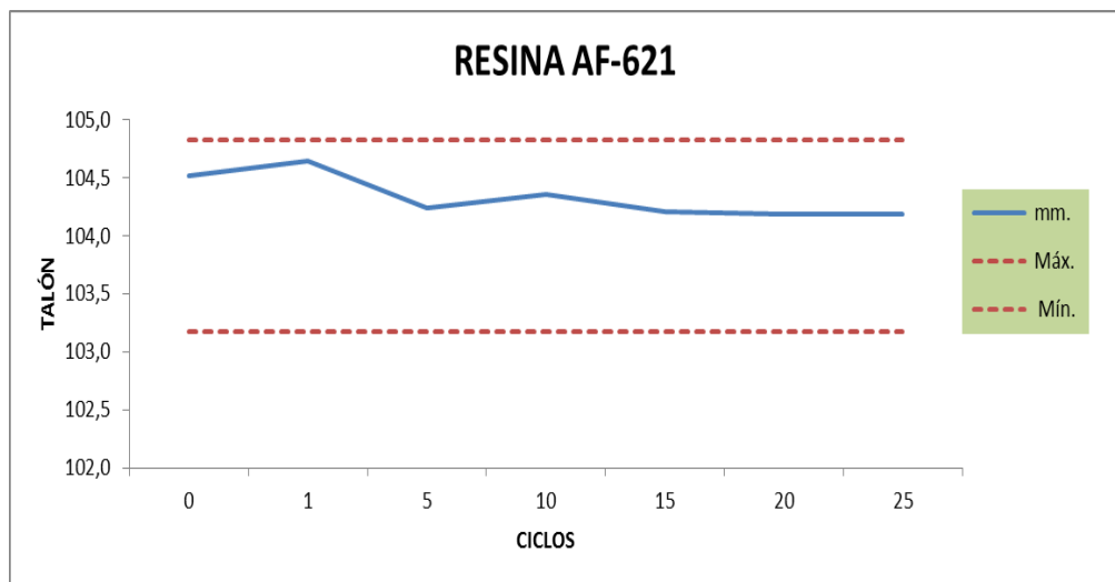
FIGURA 3.9 GRÁFICO COMPORTAMIENTO DE LA RESINA AF-621 SEGÚN EL TALÓN DEL ENVASE.
