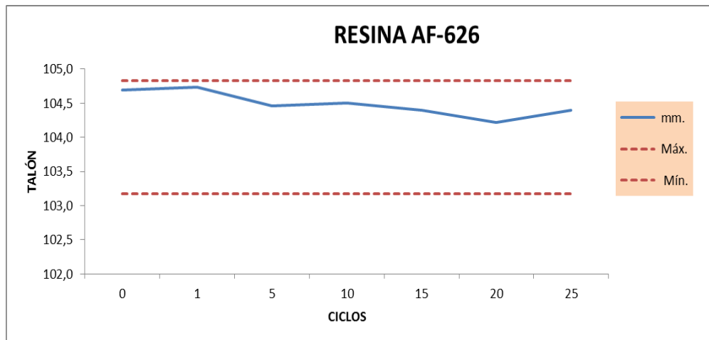
FIGURA 3.10 GRÁFICO COMPORTAMIENTO DE LA RESINA AF-626 SEGÚN EL TALÓN DEL ENVASE.
