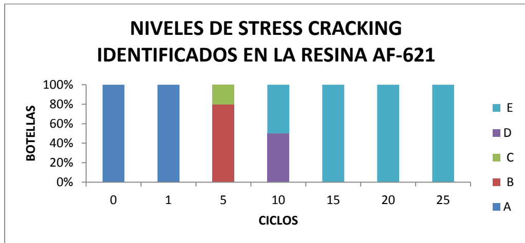
FIGURA 3.13 GRÁFICO NIVELES DE STRESS CRACKING EN LOS ENVASES DE LA RESINA AF-621
