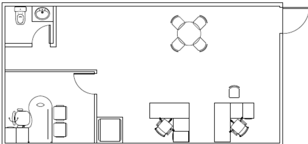
Figura 52: Plano y Análisis de Distancias para oficina administrativa (Opción 1).
