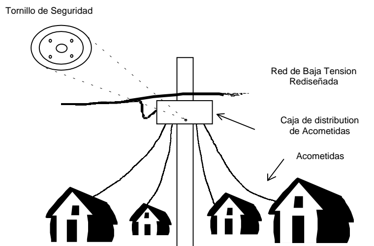
FIGURA 4.6. REDISEÑO DE LA RED DE BAJA TENSION
