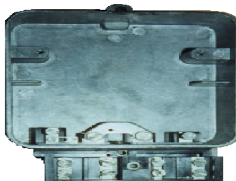
FIGURA 3.7. BASE DE UN MEDIDOR
