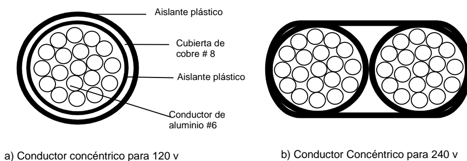
FIGURA 4.4. CONDUCTOR ANTIHURTO
